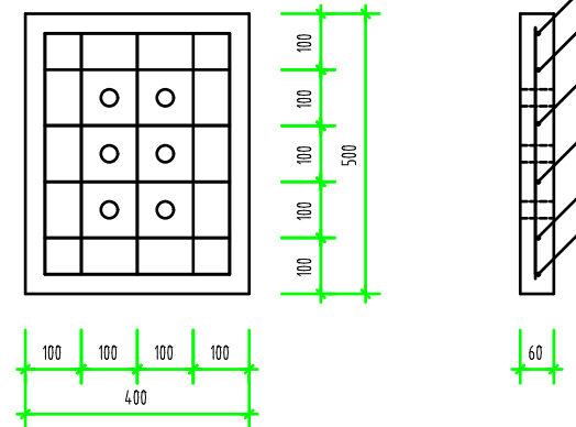
平面配筋
