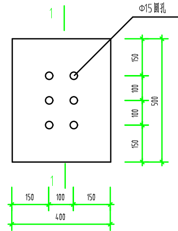
盖板平面
