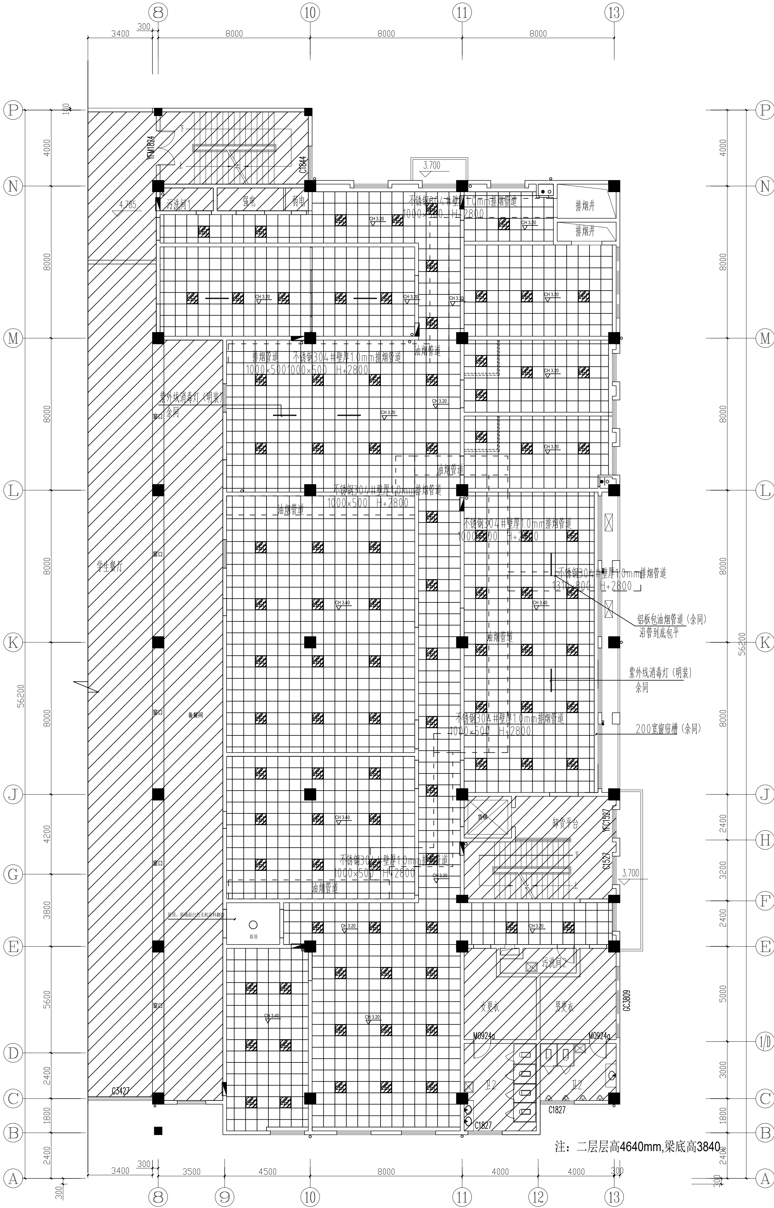
二层食堂（厨房区域）天花图 1:125
