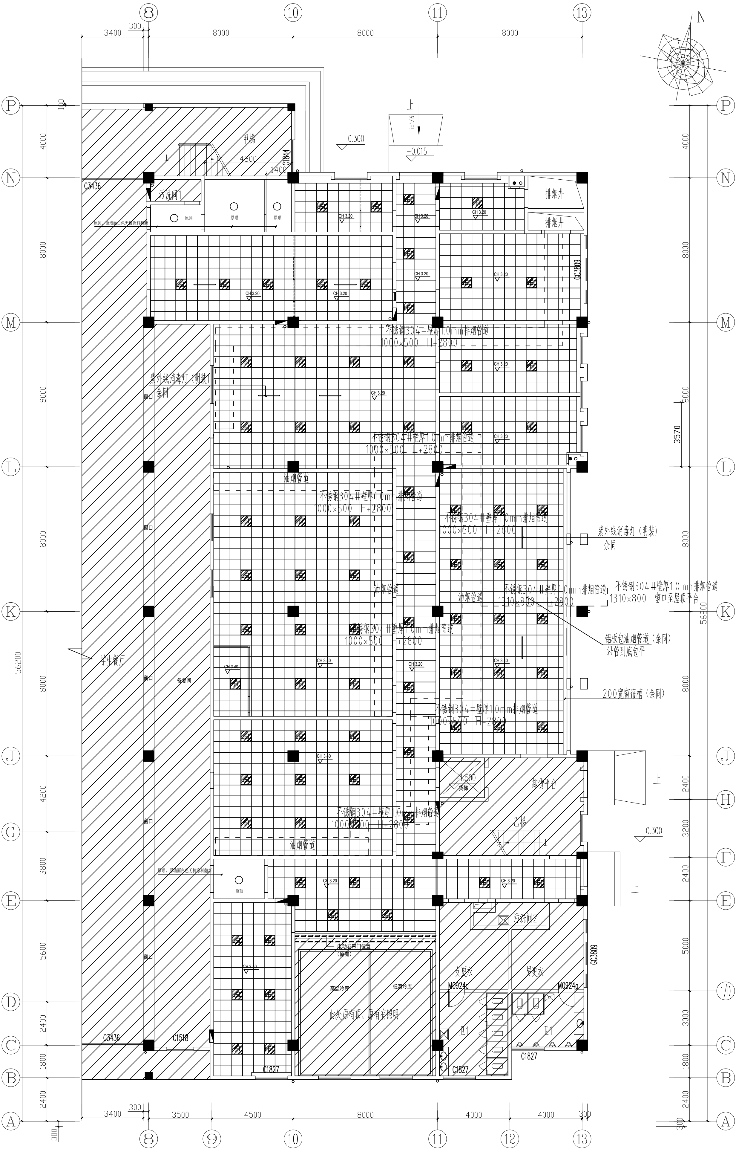
一层食堂(厨房区域)天花图 1:125
