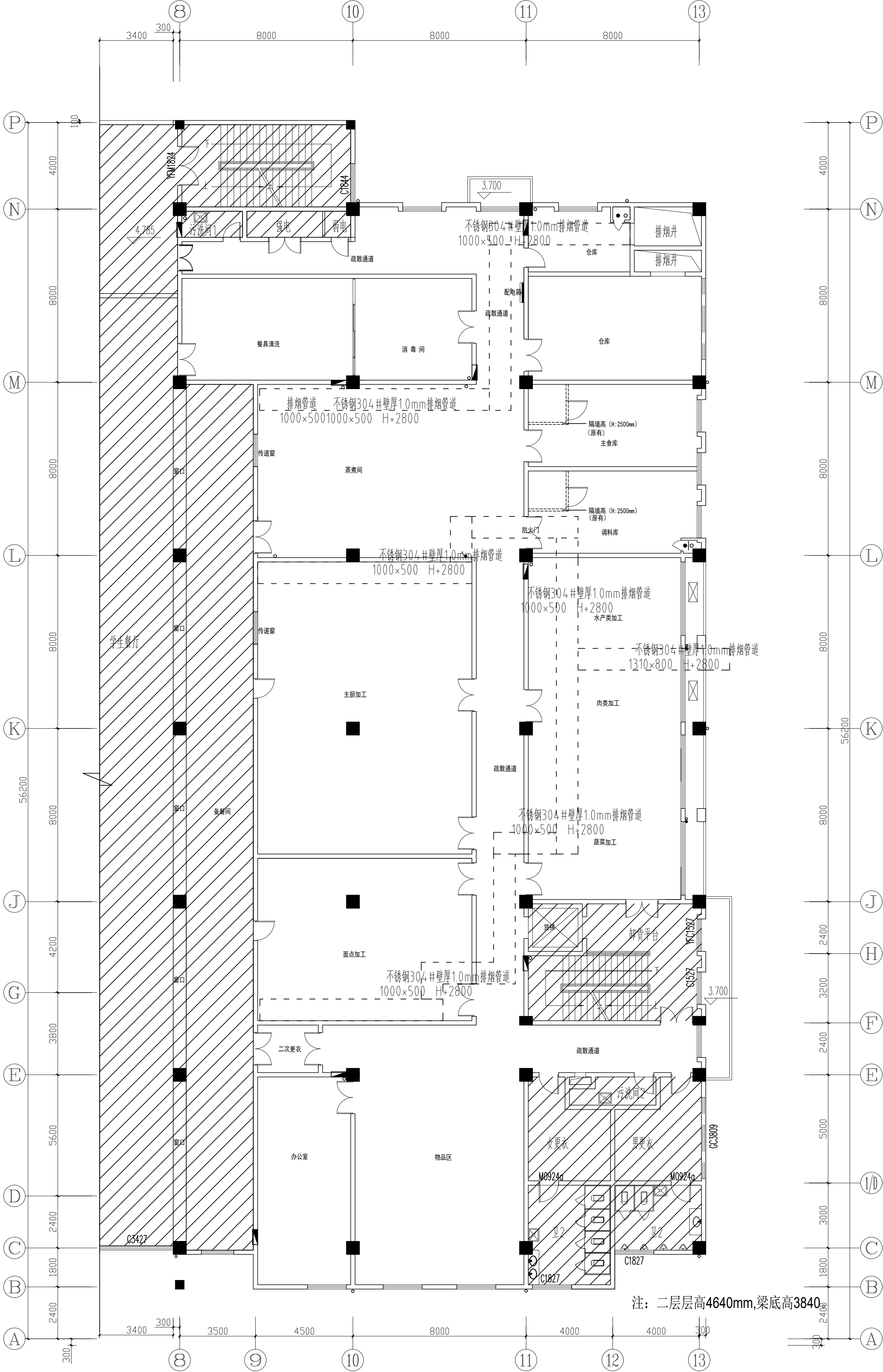
二层食堂（厨房区域）厨房油烟管道示意图
