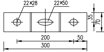
托架大样图
