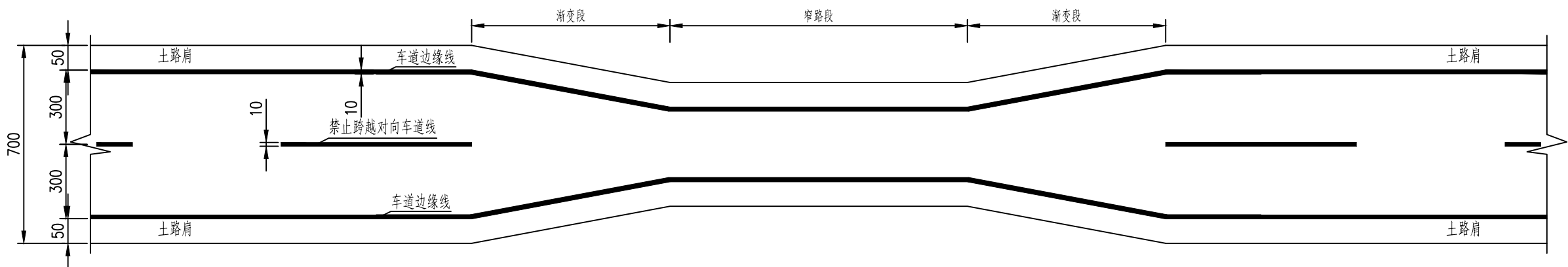
路宽变窄路段标线大样图
