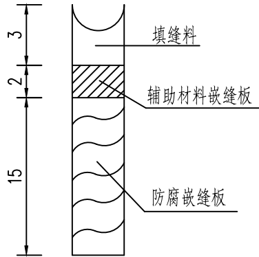
胀缝放大图
