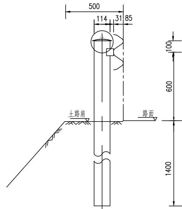
I - I 剖面图
