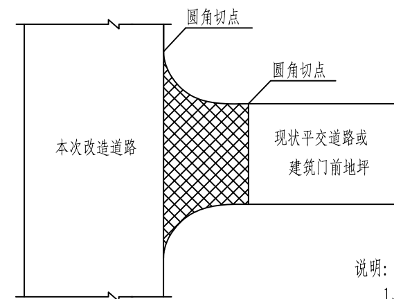
搭接平面图 有加铺转角
