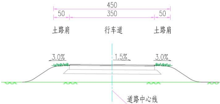
图 7 老路横断面图
