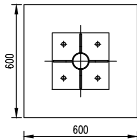
柱帽大样图
