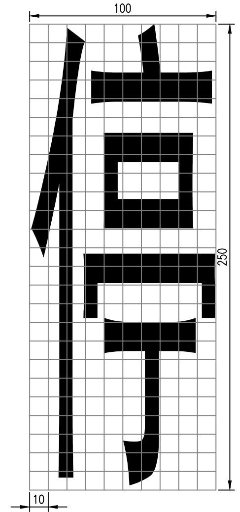
路面文字-“停”
