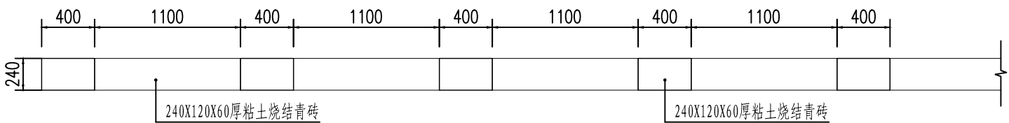
矮墙立面图
