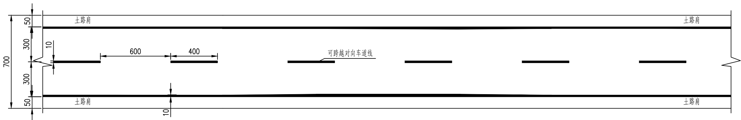
一般路段标线大样图
