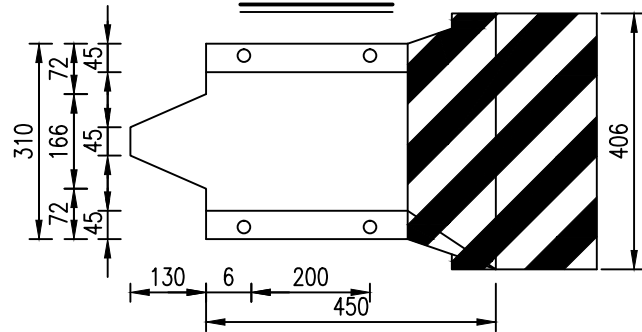
端头大样图
