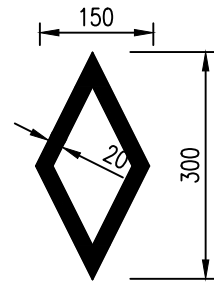
人行横道预告标识线
