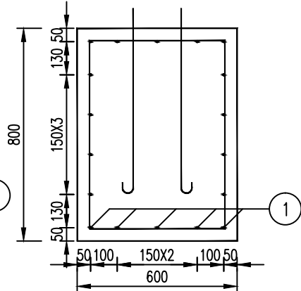
基础钢筋侧面图
