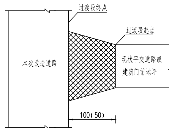
搭接平面图 无加铺转角
