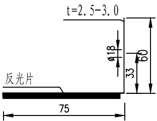
侧面图
