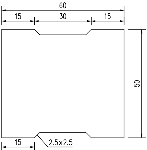
盖板平面图 1:10
