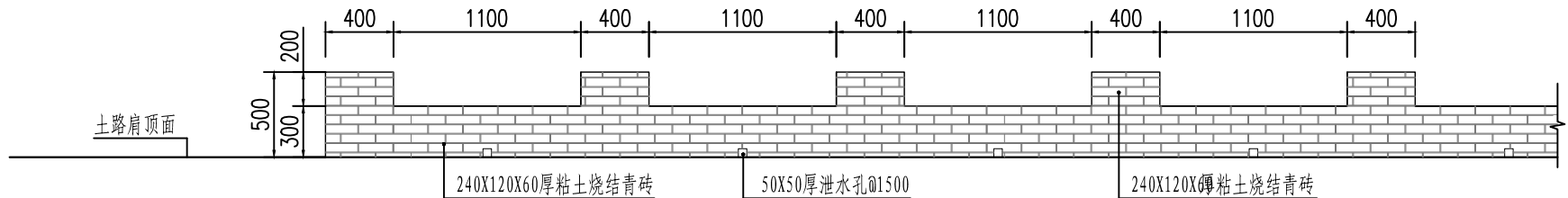
矮墙立面图
