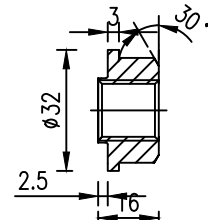
防盗螺母
