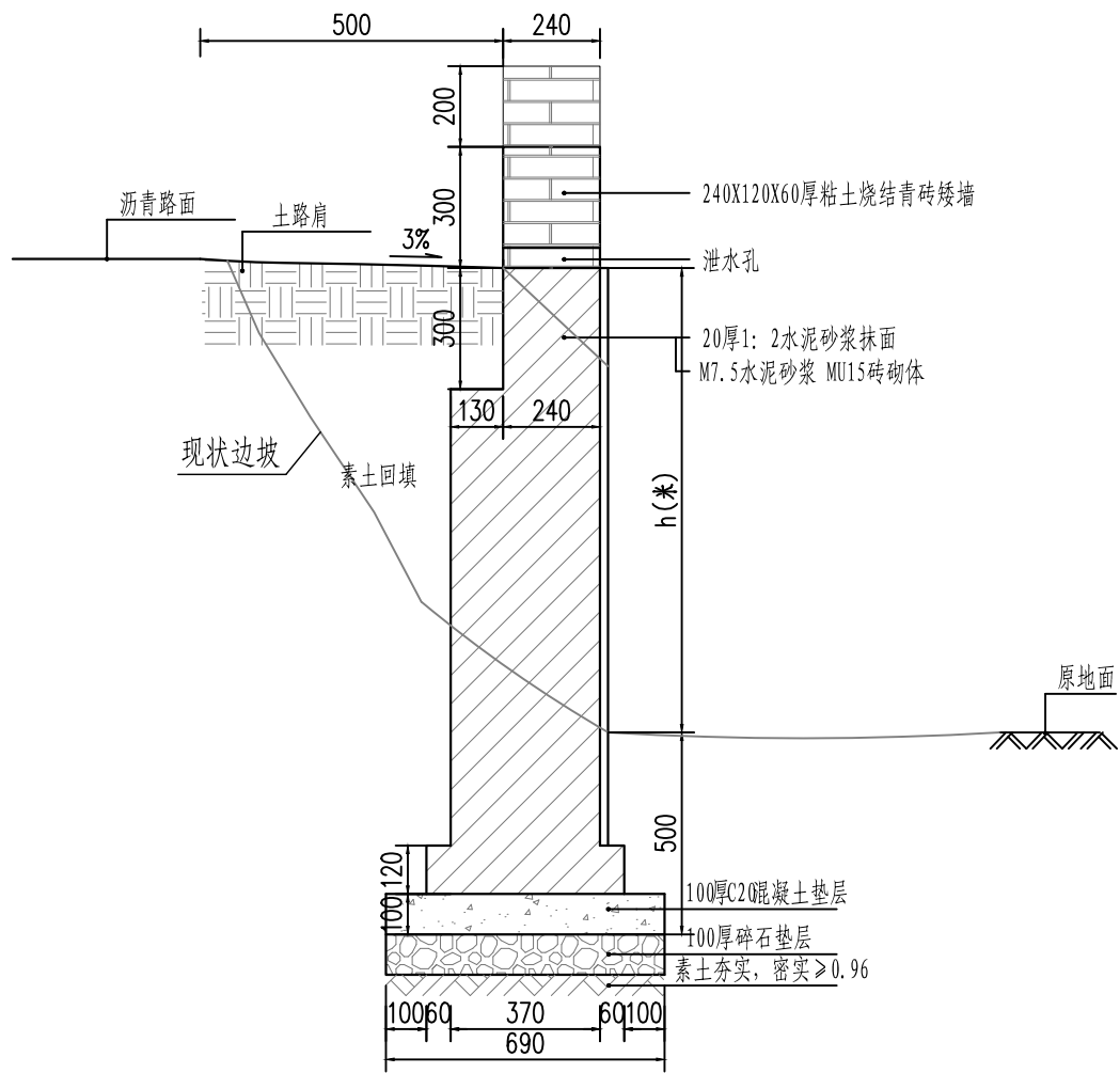
砖砌挡墙做法
