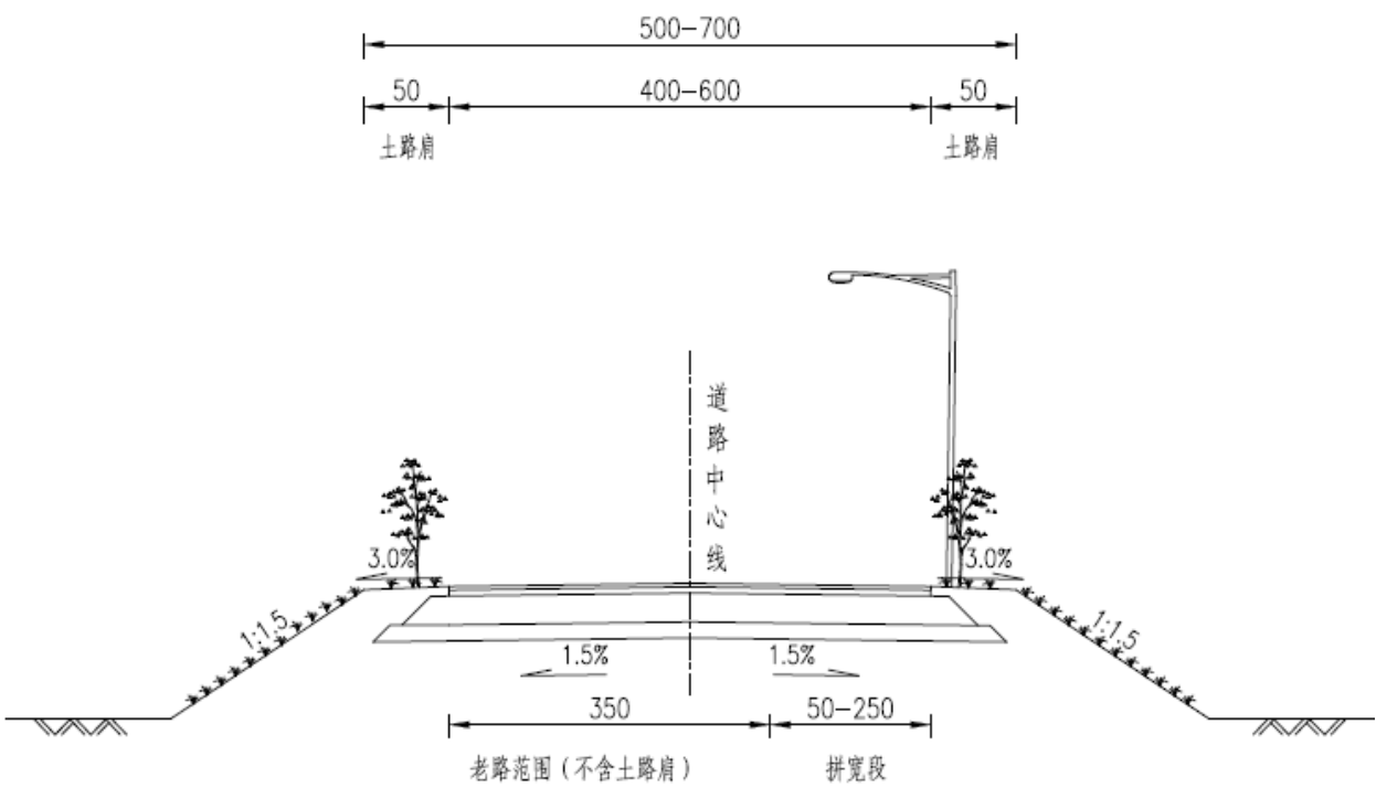
图 18 路基标准横断面图
