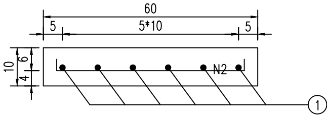
立面 1:10
