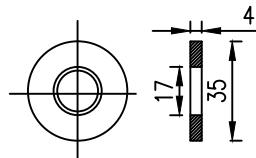
垫片
