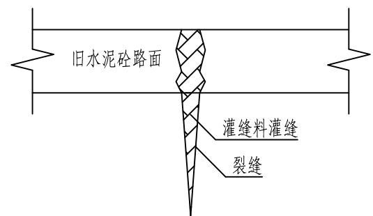
灌缝处理方案
