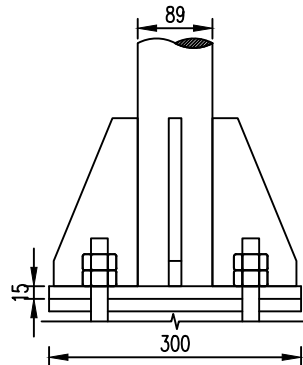
立柱底连接大样图
