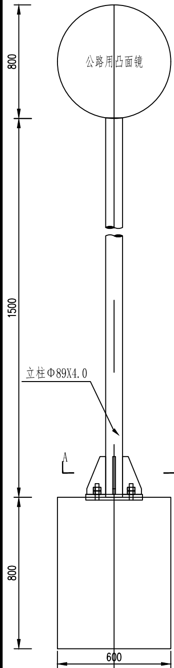
标志立面图
