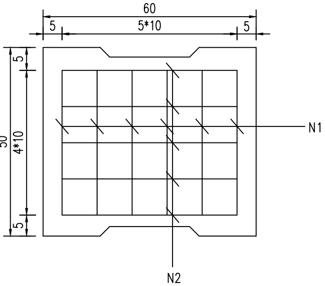
平面 1:10
