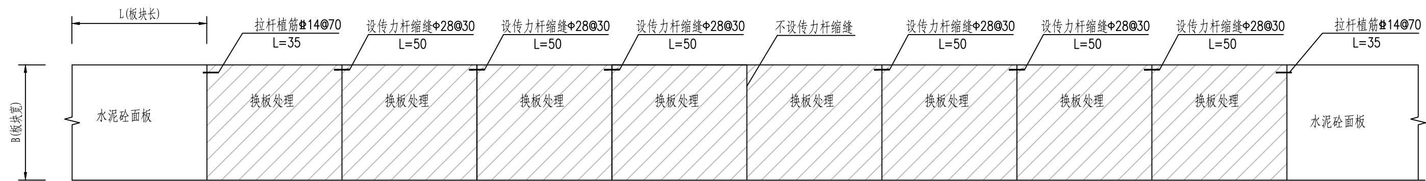
连续换板平面图
