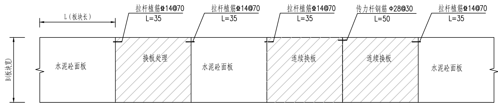
连续换板平面图
