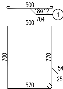
基础钢筋大样
