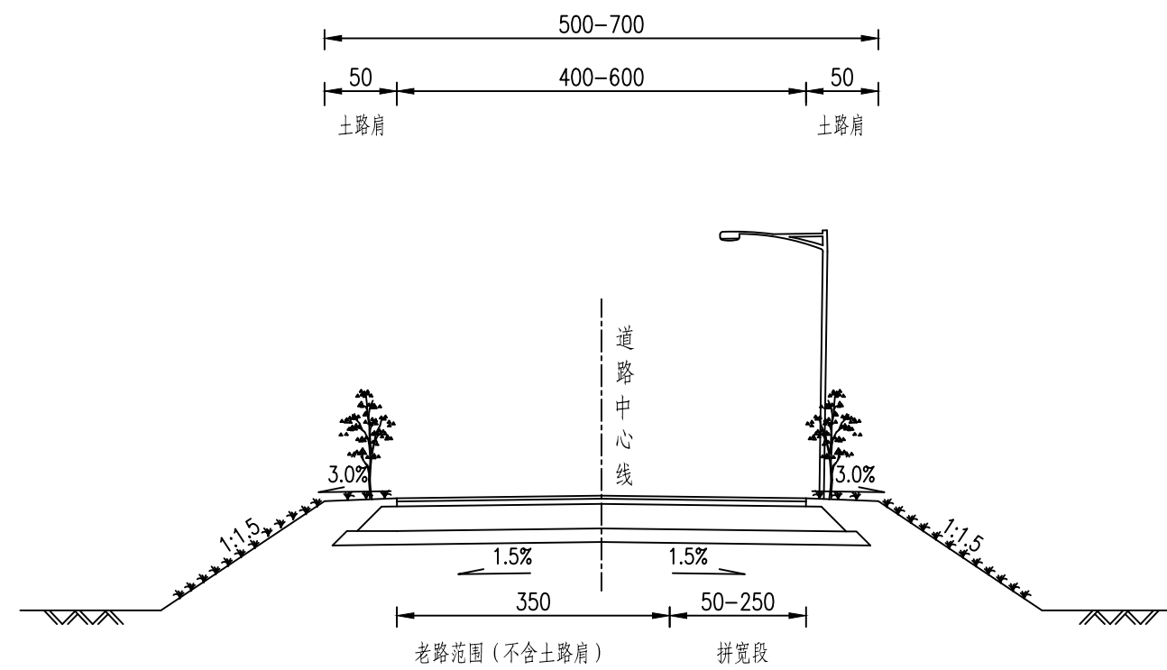
路基标准横断面图
