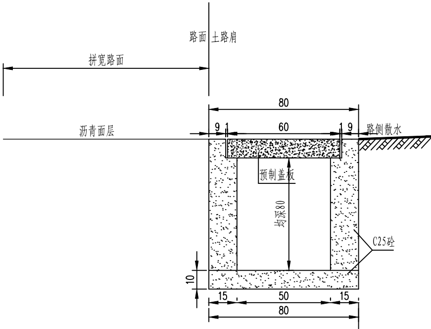
盖板边沟设计图
