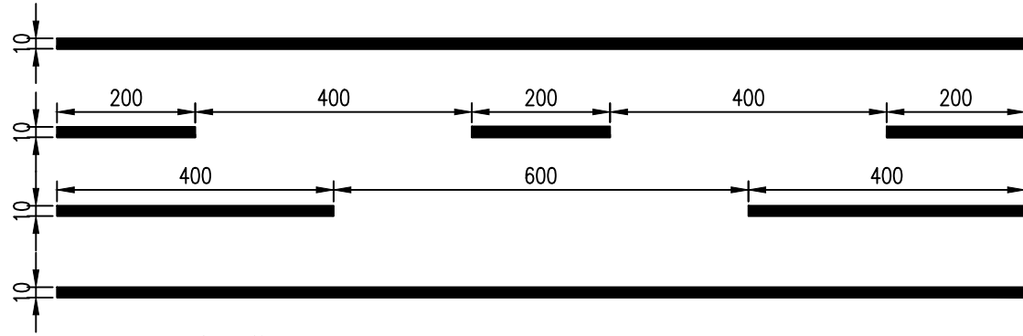
人行横道预告标识线
