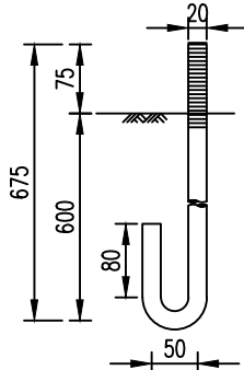
地脚螺栓大样图
