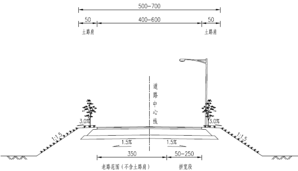
图 1 路基标准横断面图
