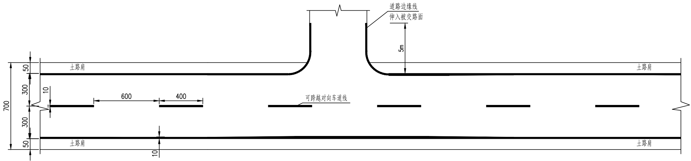
接入口大样图二 (接入口为非铺装路面)
