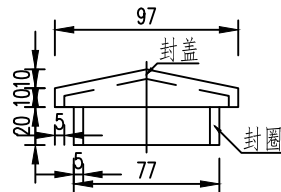
柱帽大样图
