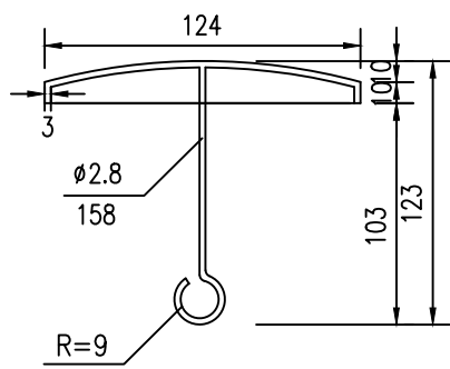
A大样
