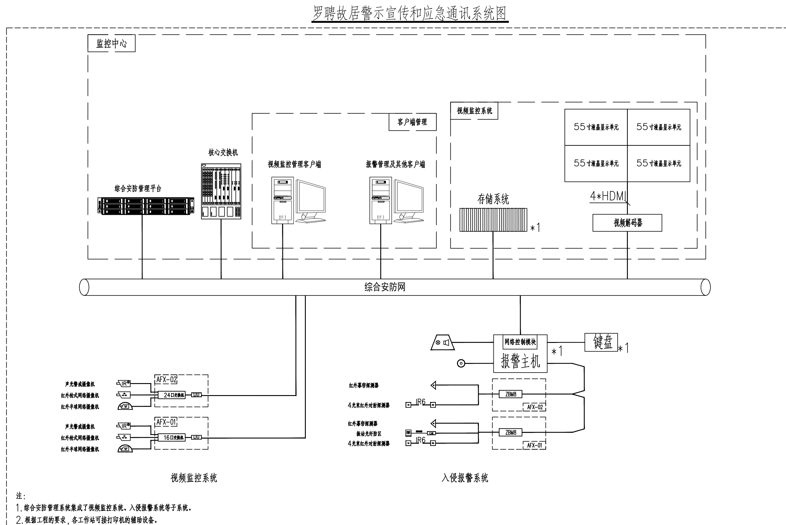
综合安防系统集成图 注：各系统设备配置详见各子系统图
