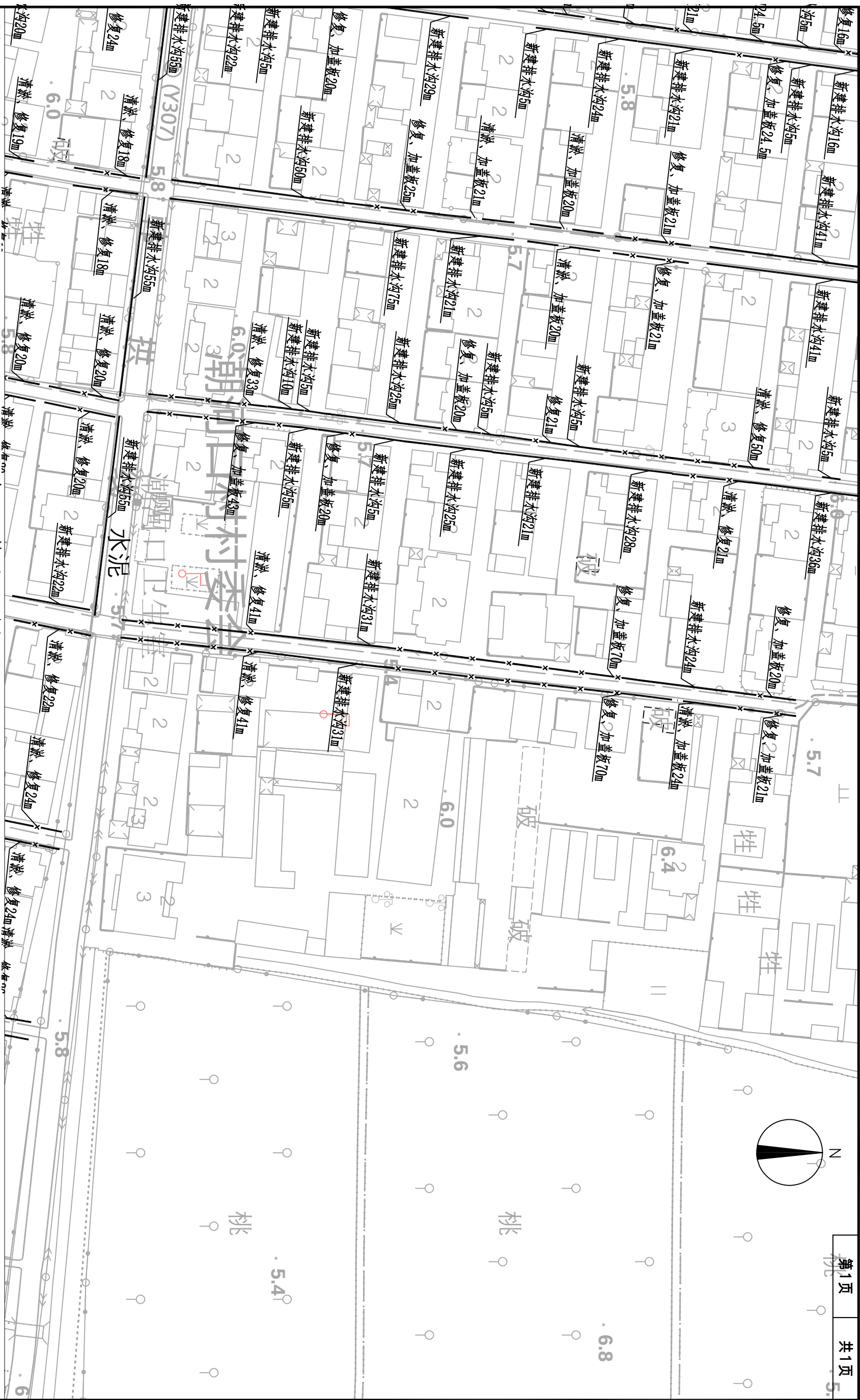
潮河口管网平面图1:1000
