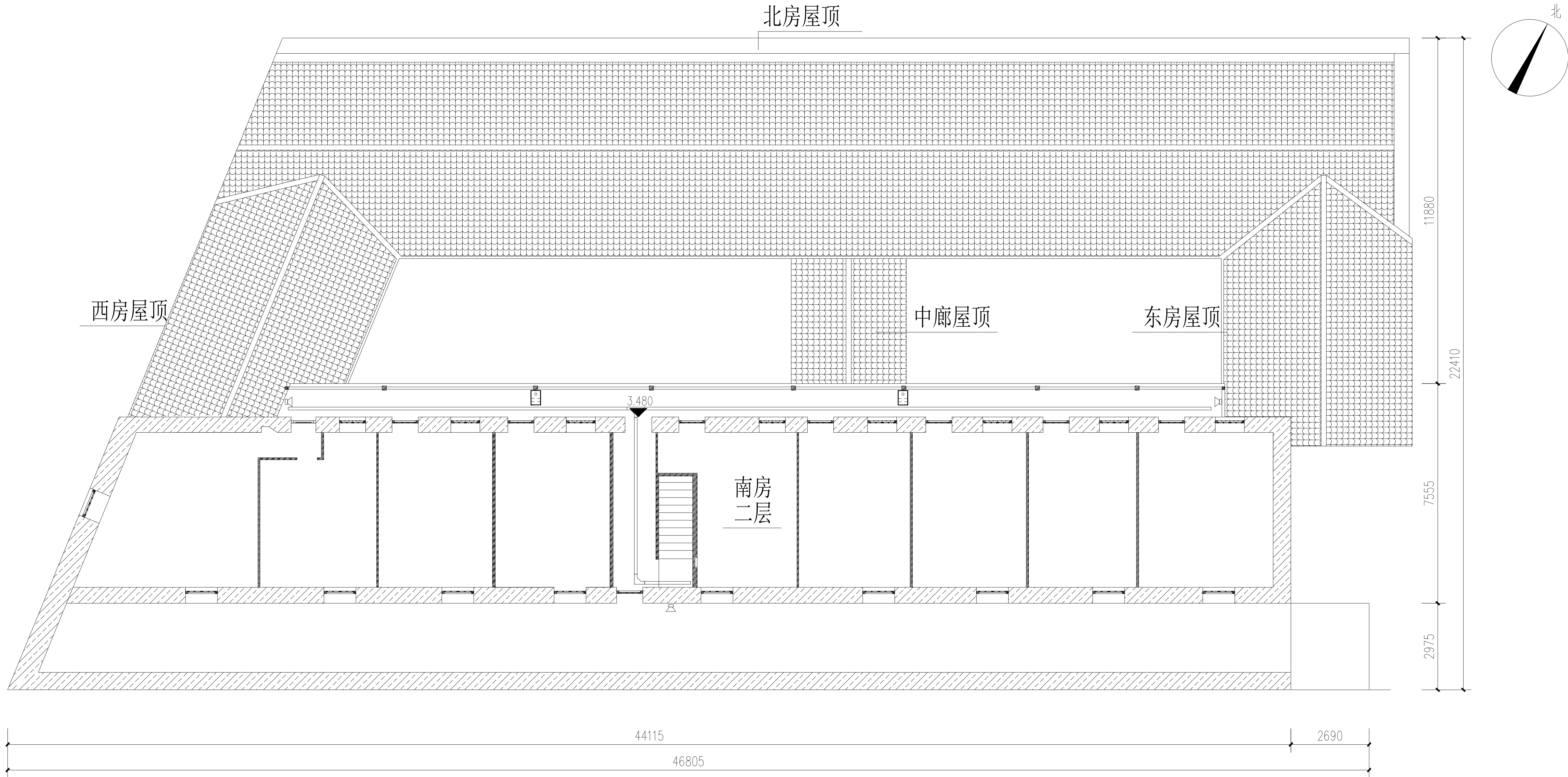
院落二层总平面图 (1/10)
