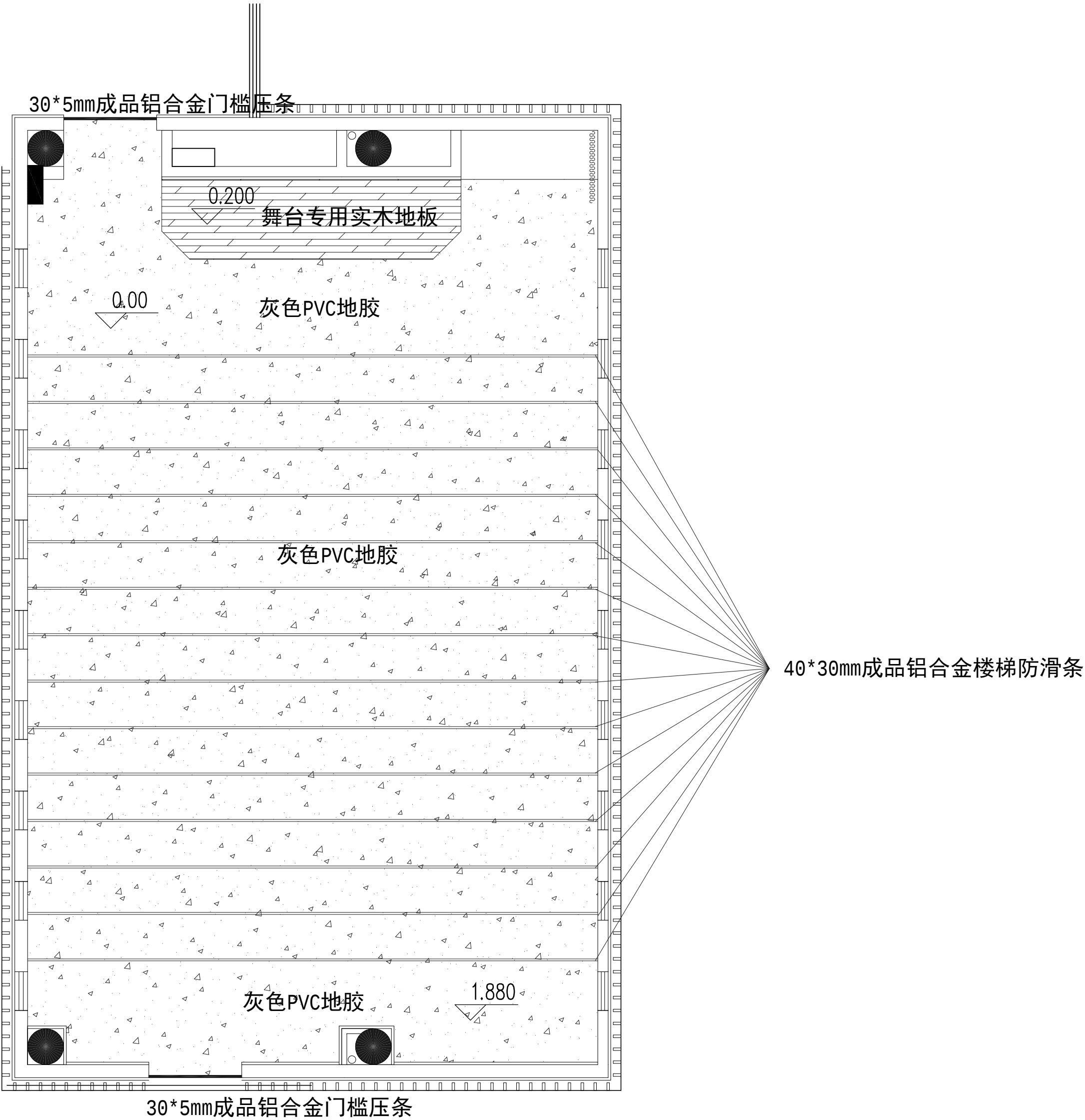
阶梯教室地面布置图 1:100
