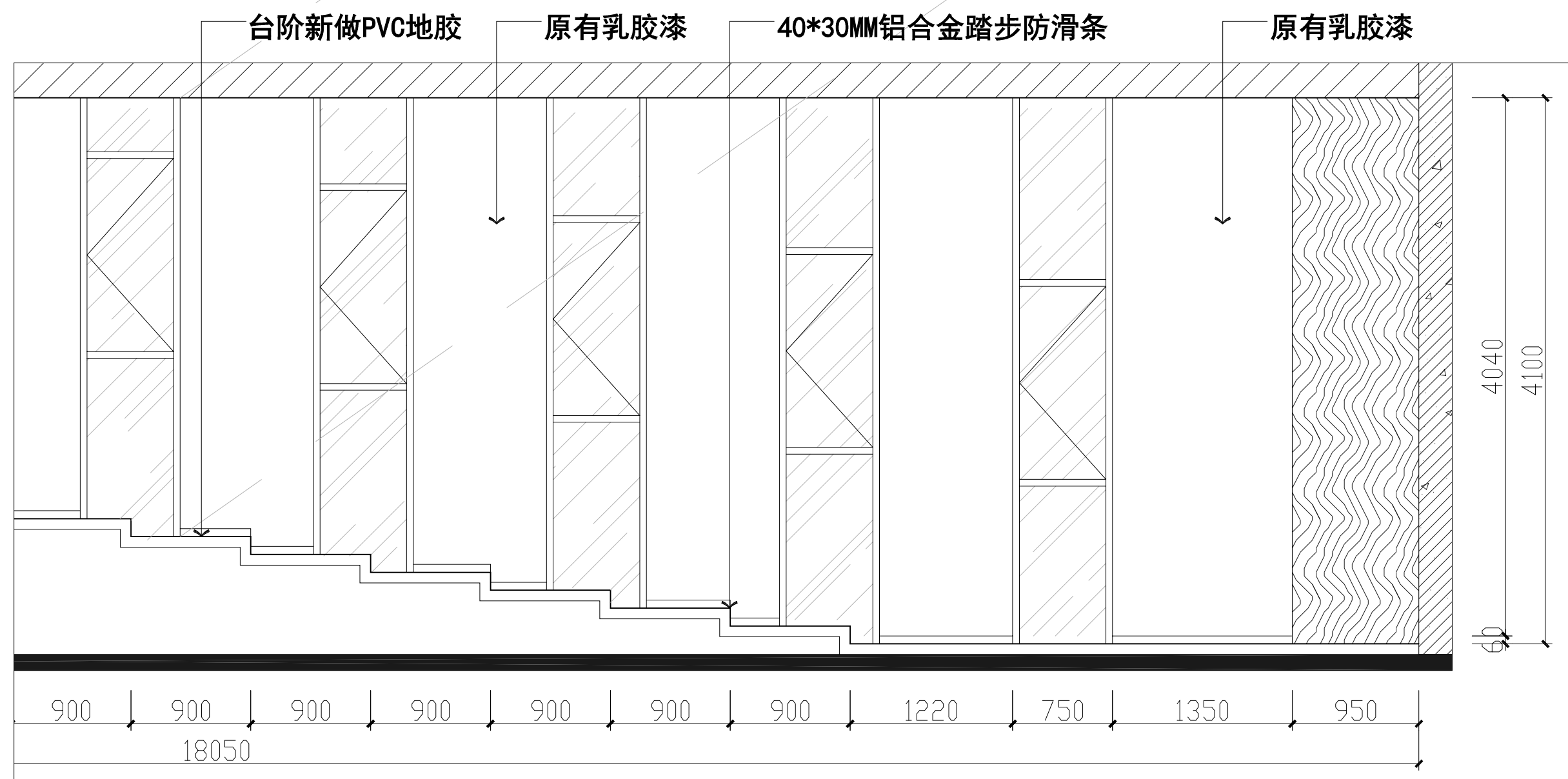
阶梯教室立面图2 1:50
