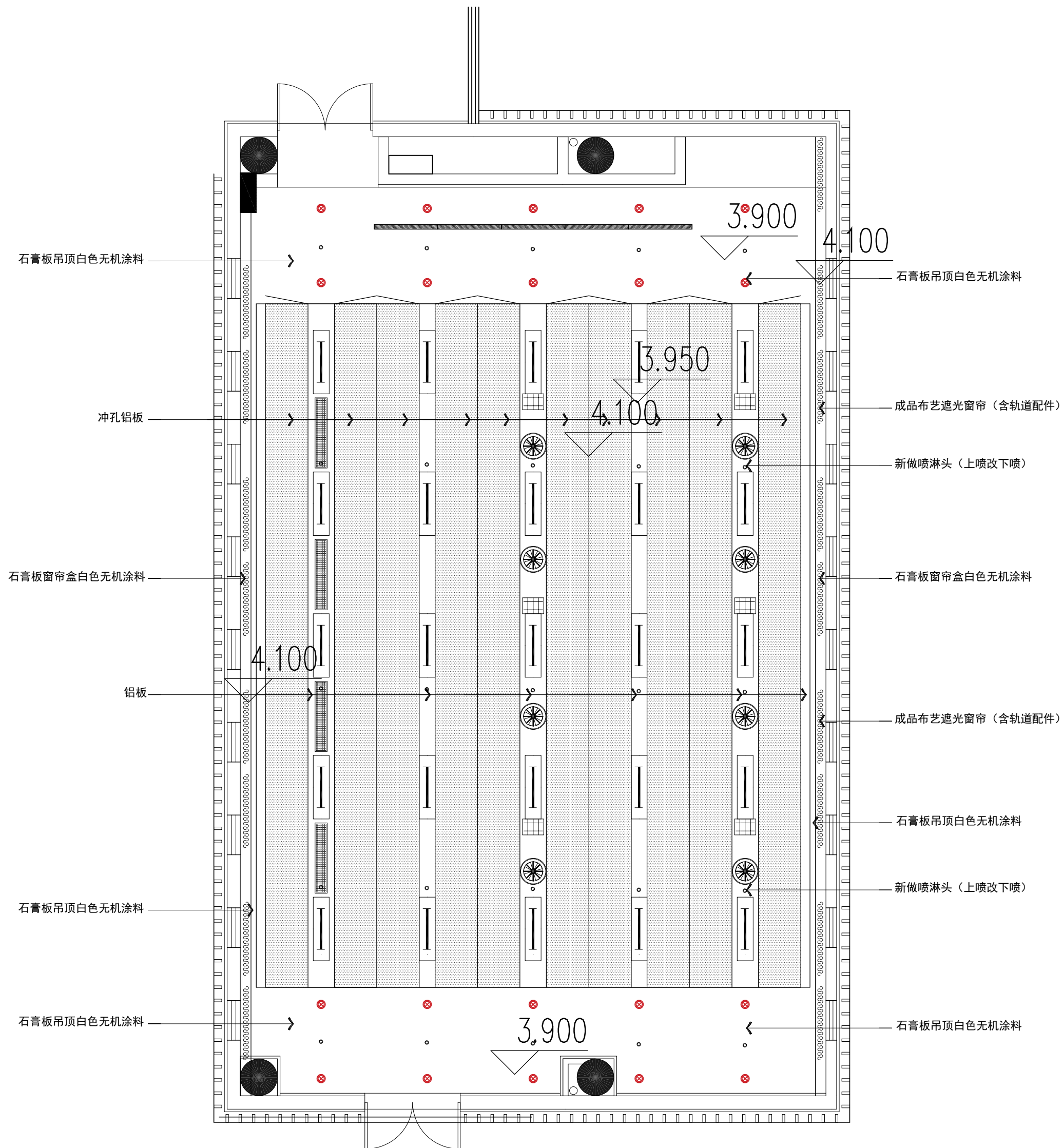
阶梯教室顶面布置图 1:100
