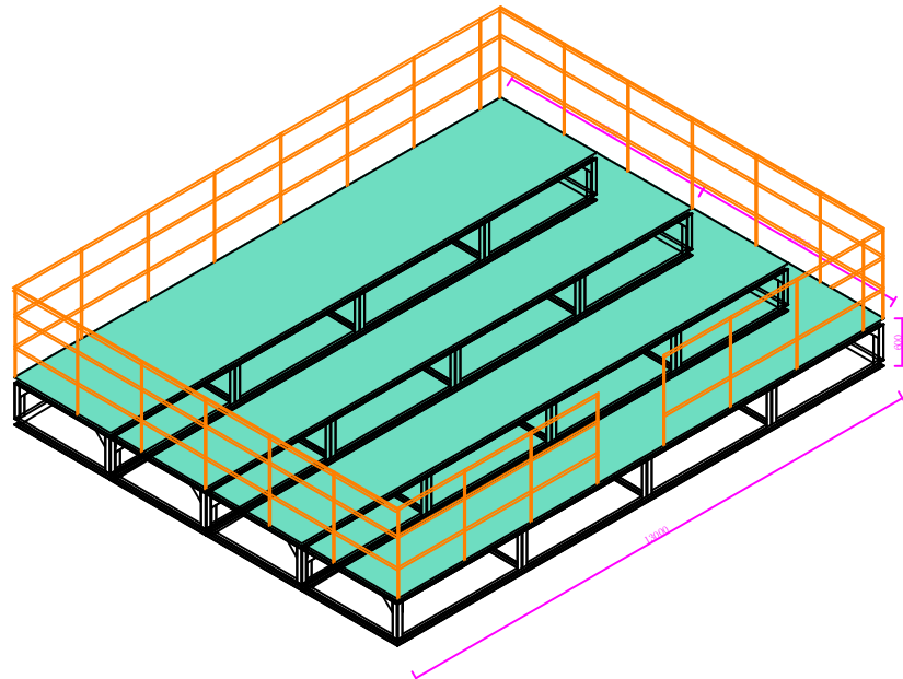
平台尺寸13000*6000*600 材料10#国标槽钢+花纹板
