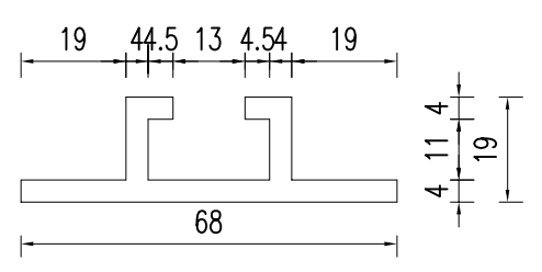
铝合金龙骨截面
