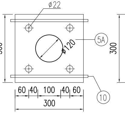
立柱法兰盘平面
