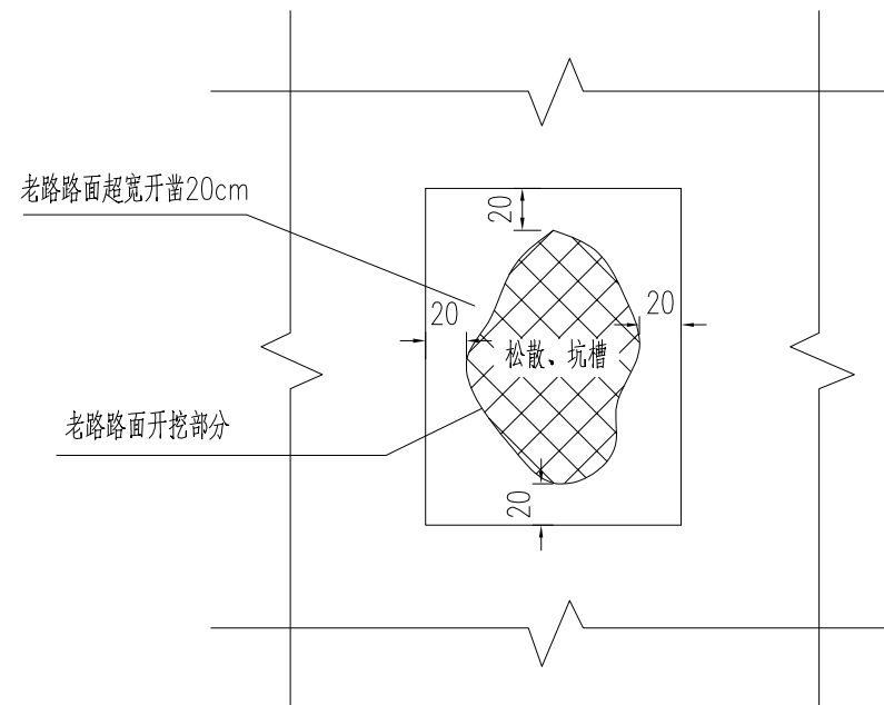
水泥砗板板角损坏处理示意图
