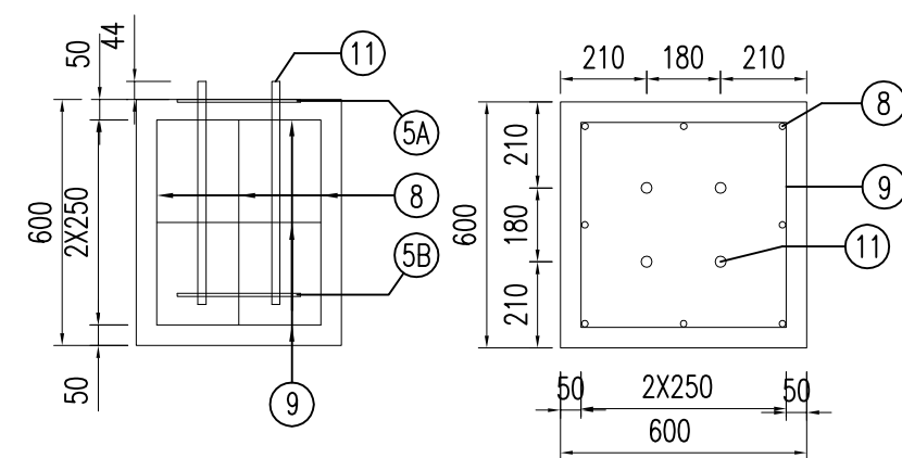
基础钢筋立面
