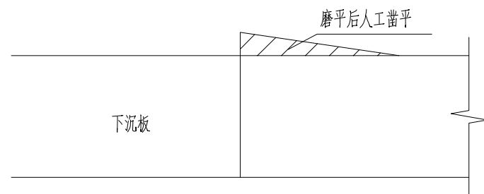
砗板块错台处治图
