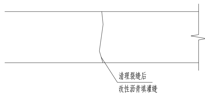
砗板块裂缝处处理图
