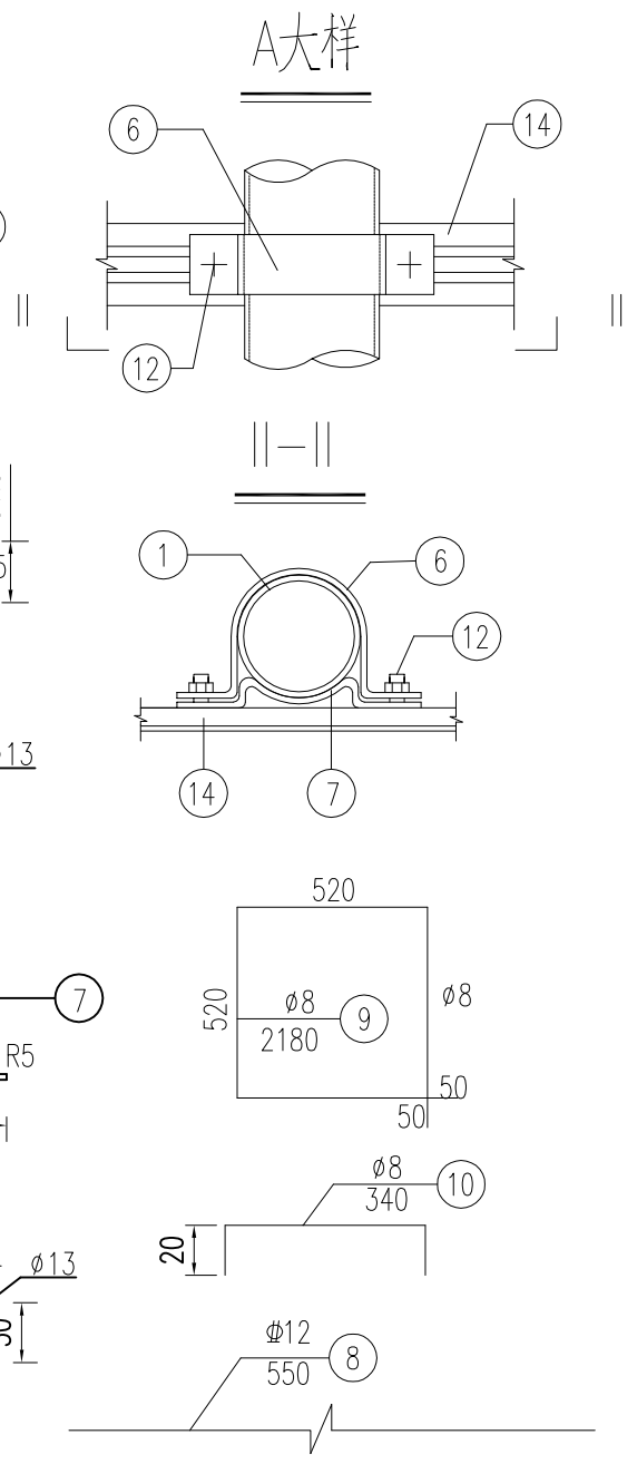
基础锚板平面
