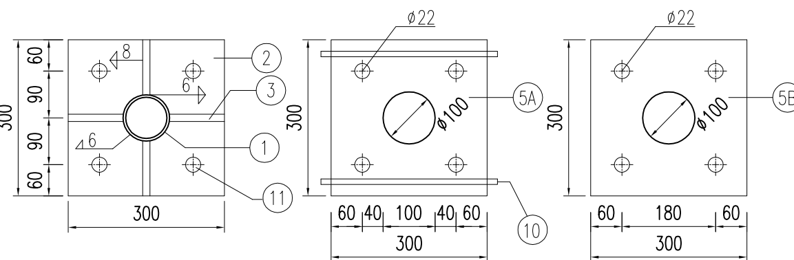
立柱法兰盘平面
