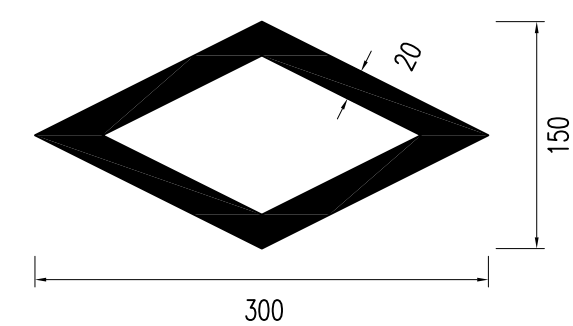
人行横道预告标识线
