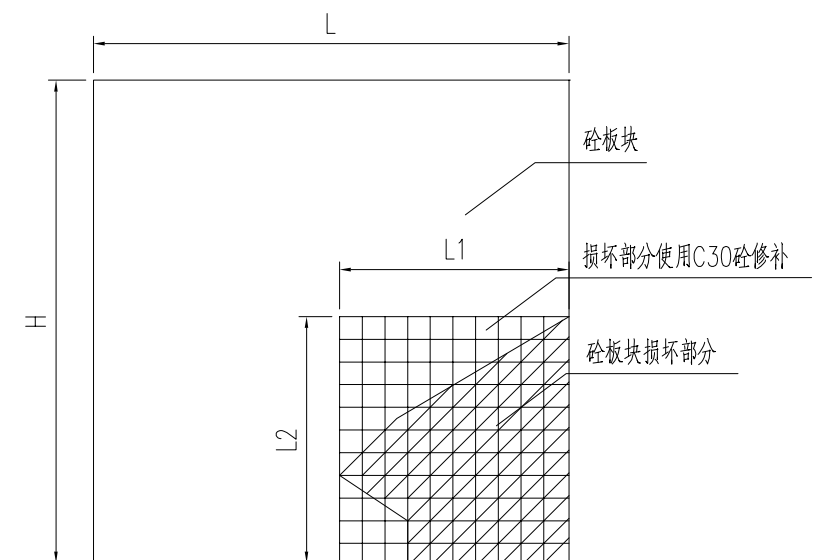
水泥砗板板角损坏处理示意图
