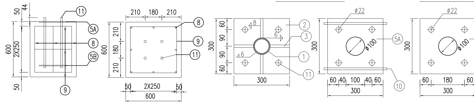
立柱法兰盘平面
