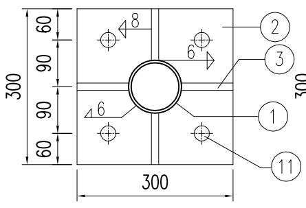
立柱法兰盘平面
