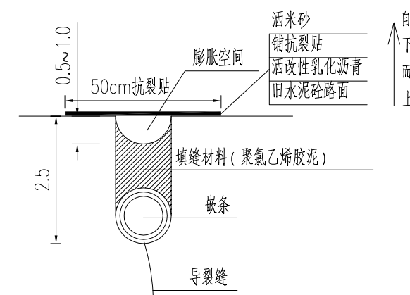
接缝填料修补示意图
