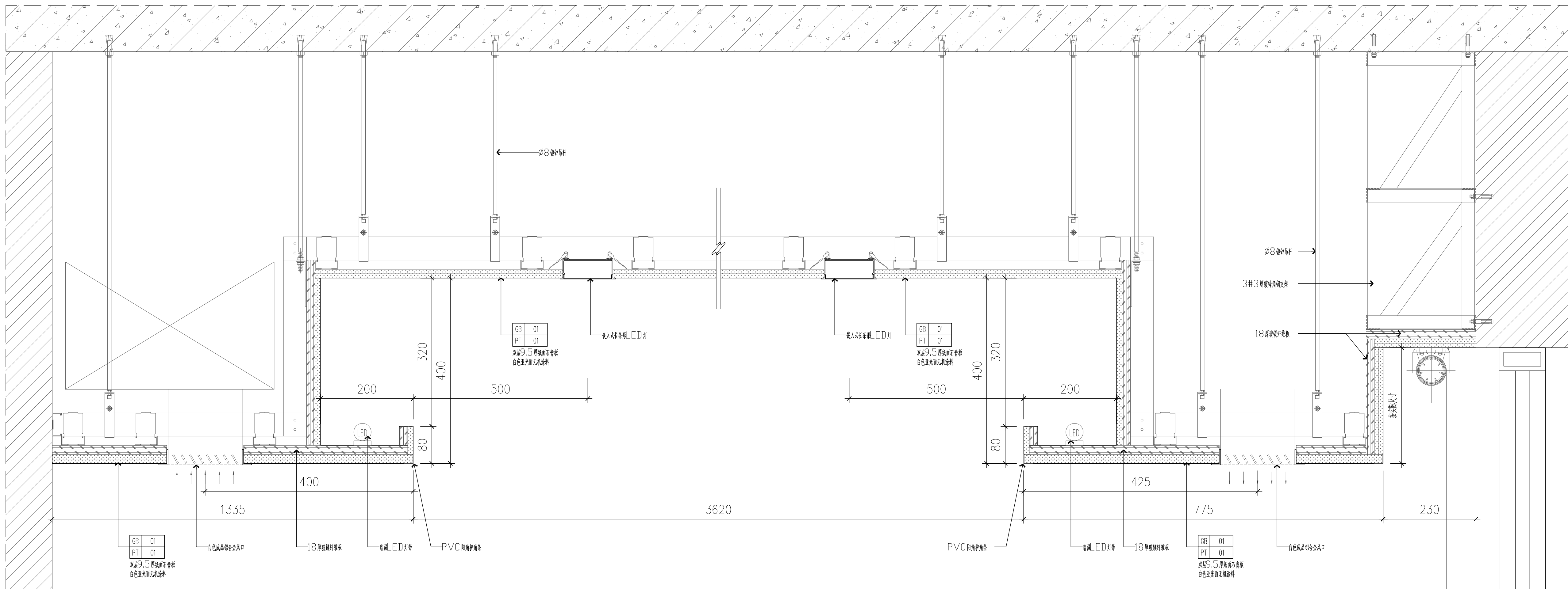
S10 部分用房1大会议室吊顶节点图 -- SECTION 1:5
