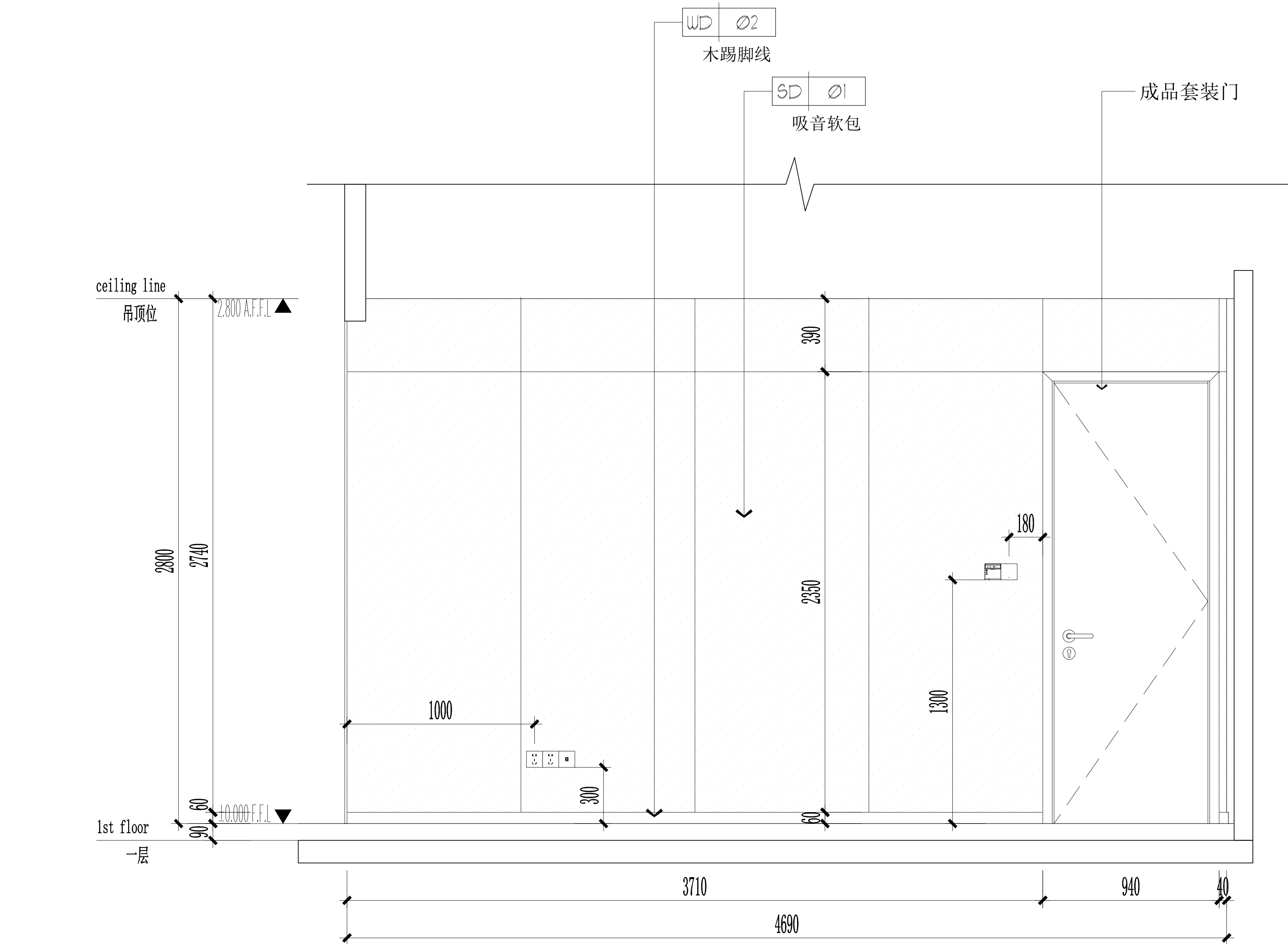
07 40-P-12 ELEVATION 独立学习室1立面图 SCALE 1:30
