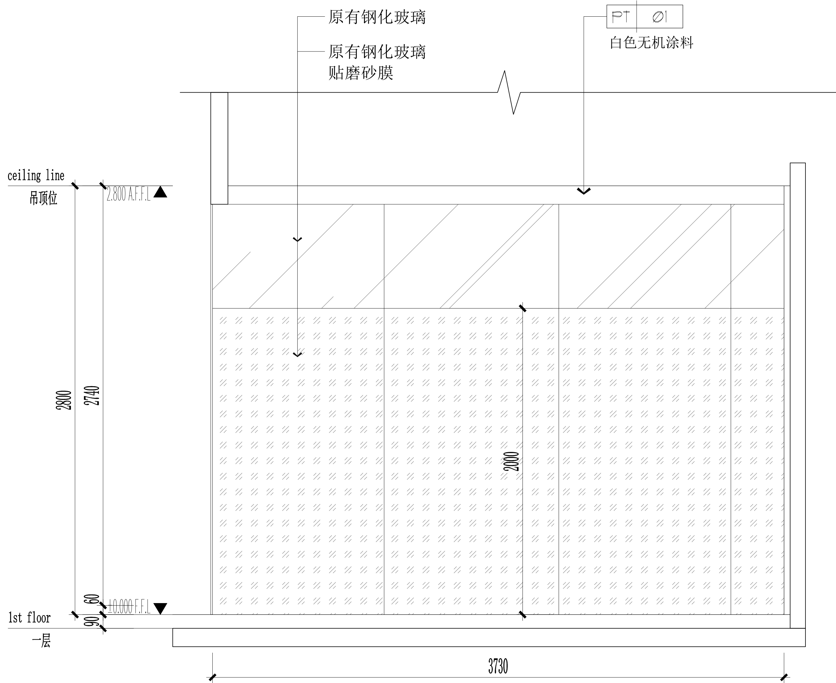
06 40-P-12 ELEVATION 独立学习室1立面图 SCALE 1:30
