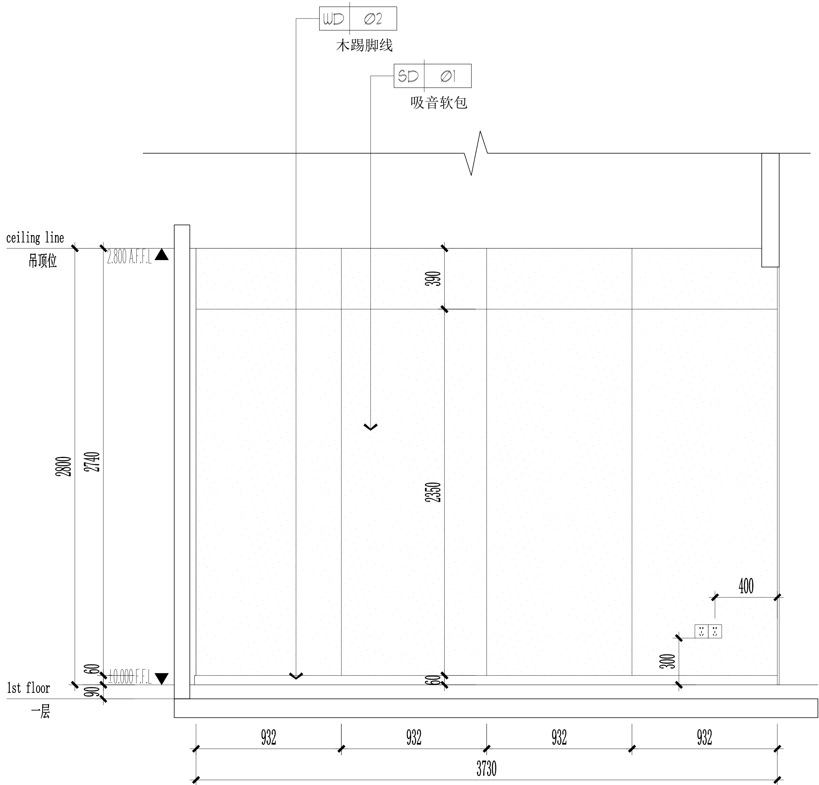
08 40-P-12 ELEVATION 独立学习室1立面图 SCALE 1:30
