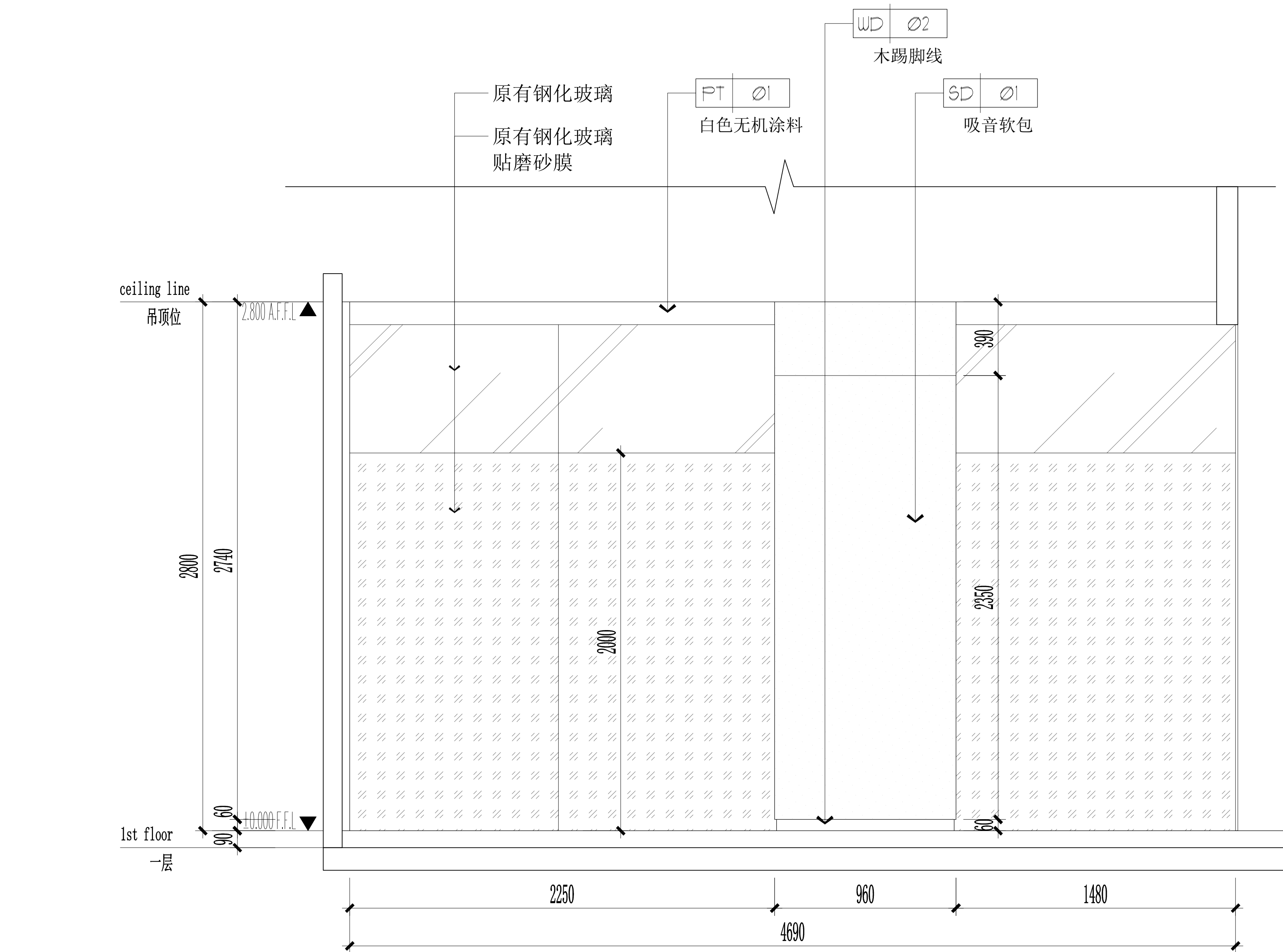
05 40-P-12 ELEVATION 独立学习室1立面图 SCALE 1:30
