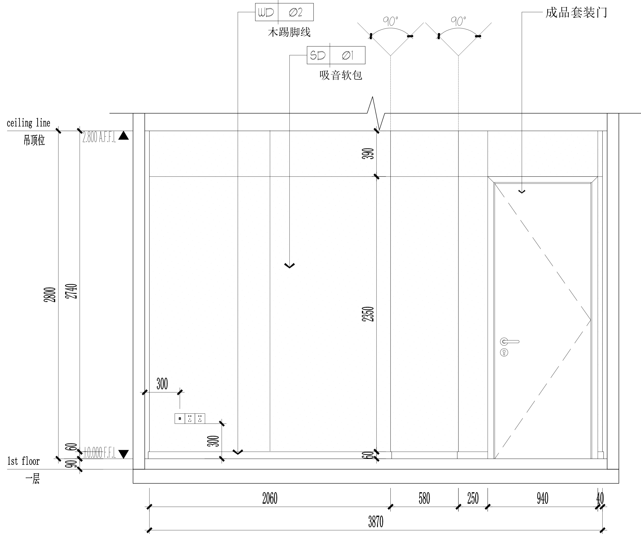
12 40-P-12 ELEVATION 独立学习室2立面图SCALE 1:30
