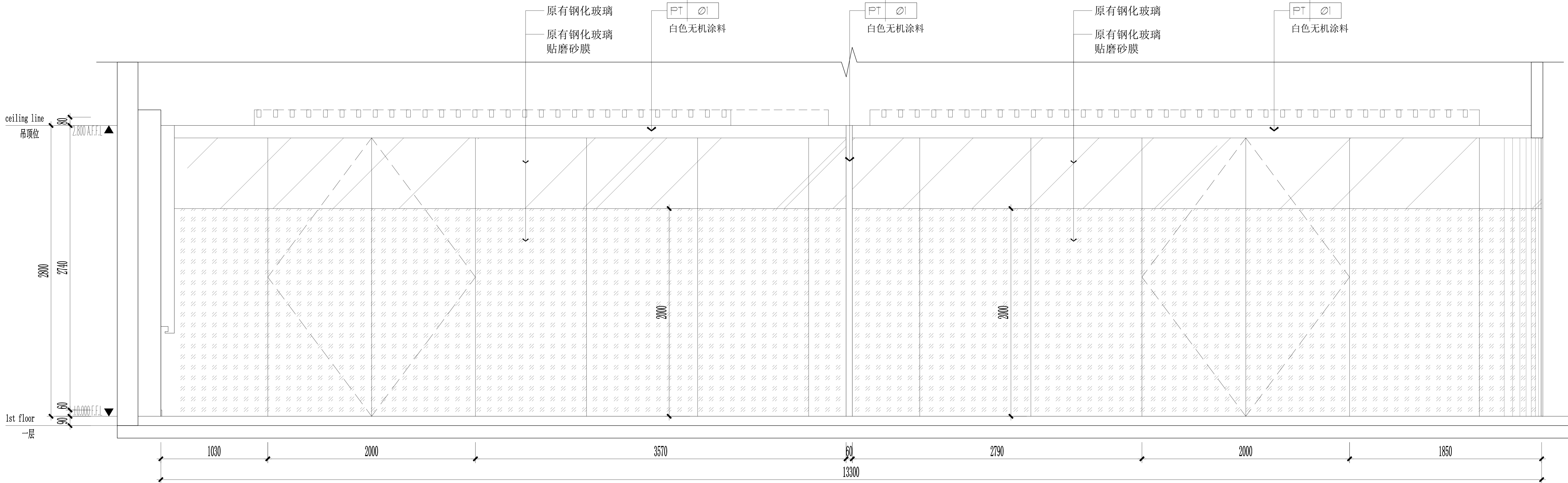
04 4Q-P-12 多功能教室立面图 SCALE 1:30
