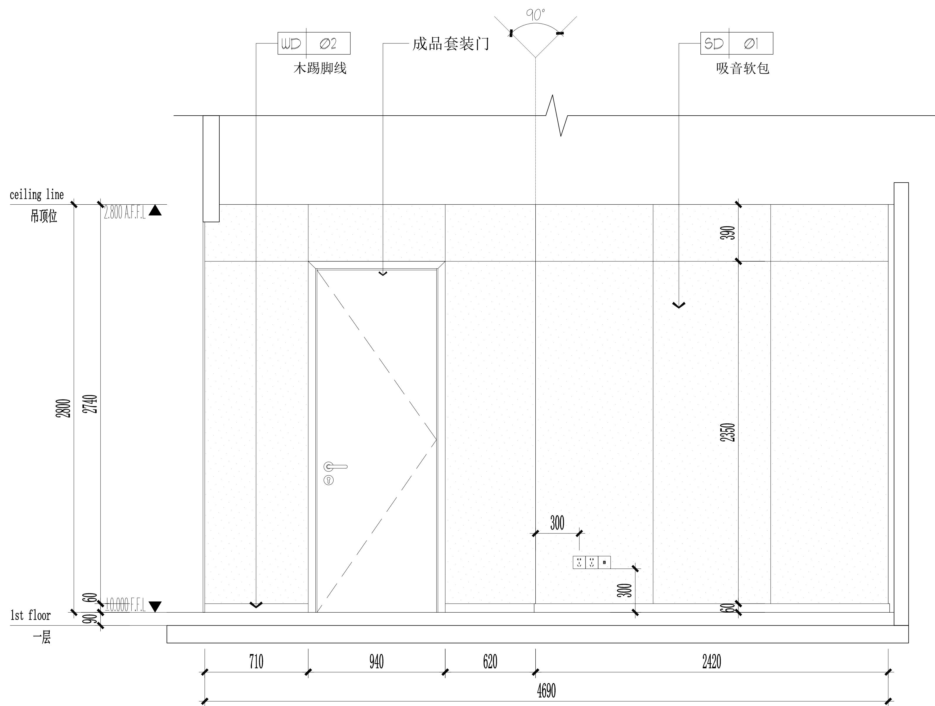
15 40-P-12 ELEVATION 独立学习室3立面图 SCALE 1:30
