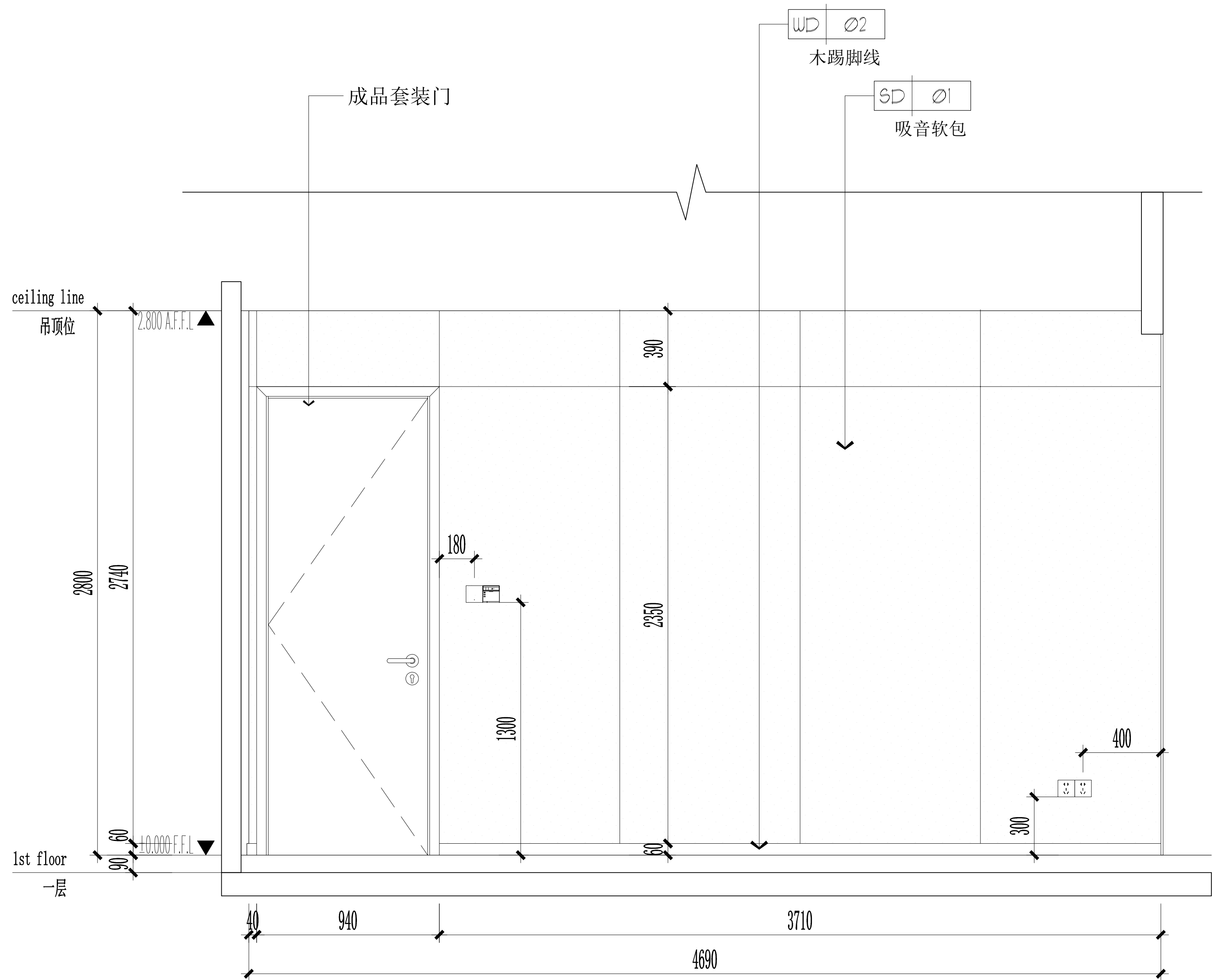
13 40-P-12 ELEVATION 独立学习室3立面图 SCALE 1:30
