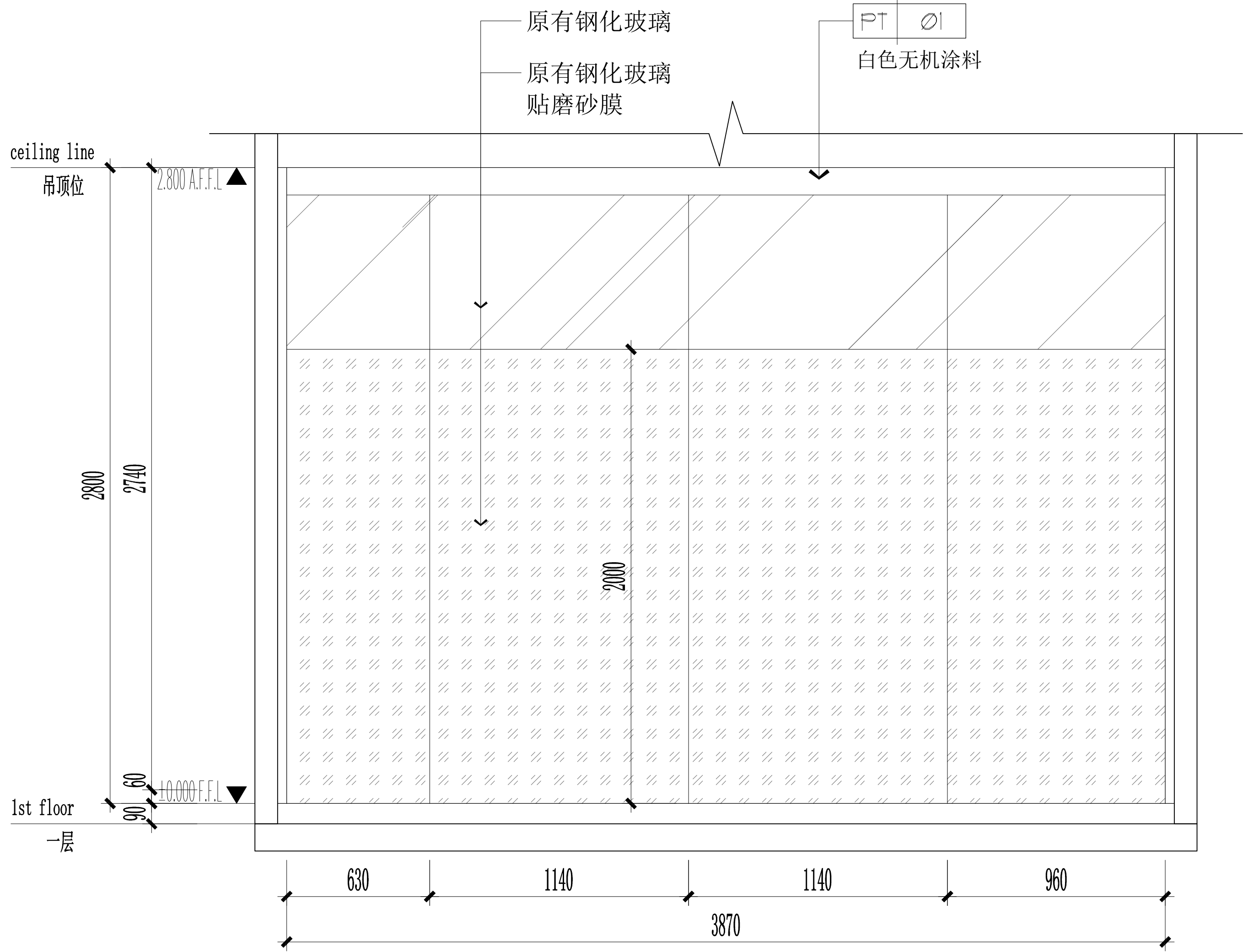
10 40-P-12 ELEVATION 独立学习室2立面图SCALE 1:30
