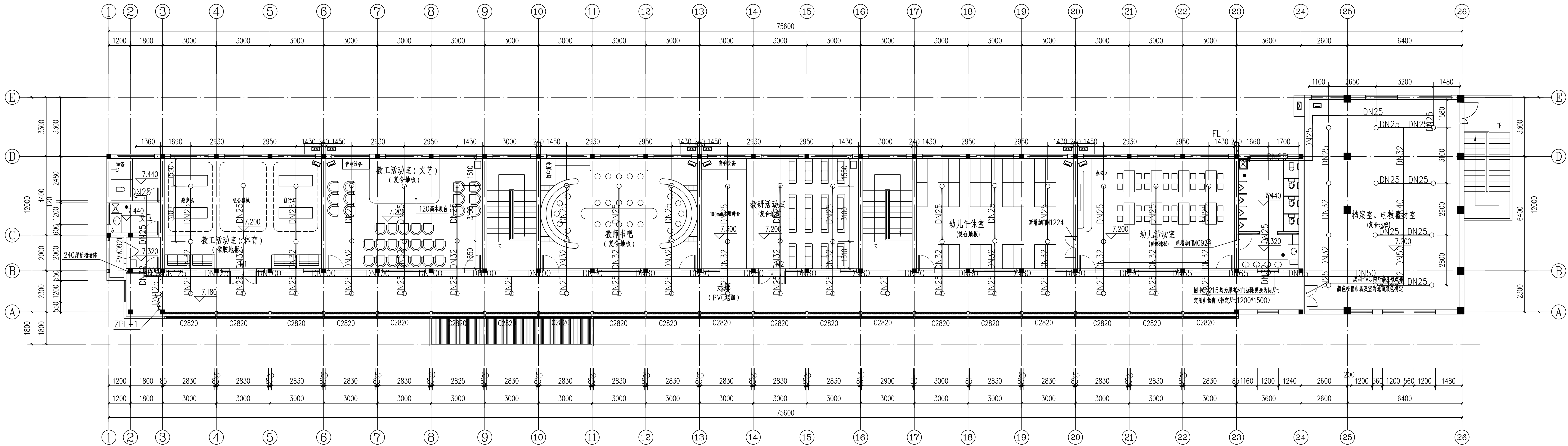
三层自动喷淋平面图 1:100
