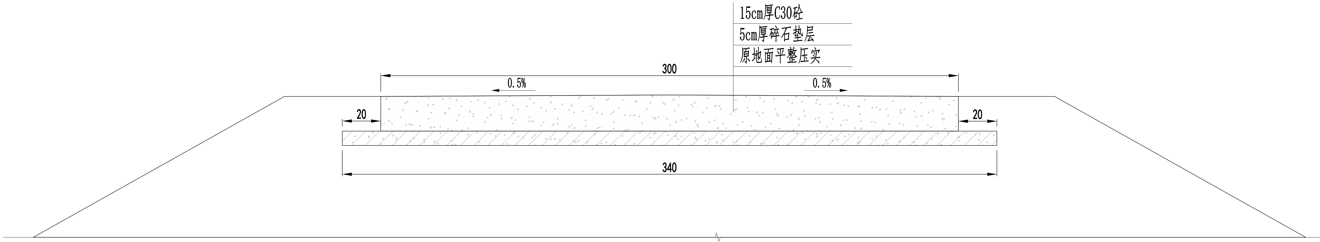
3.0m宽15cm厚砼路面断面图 1:100
