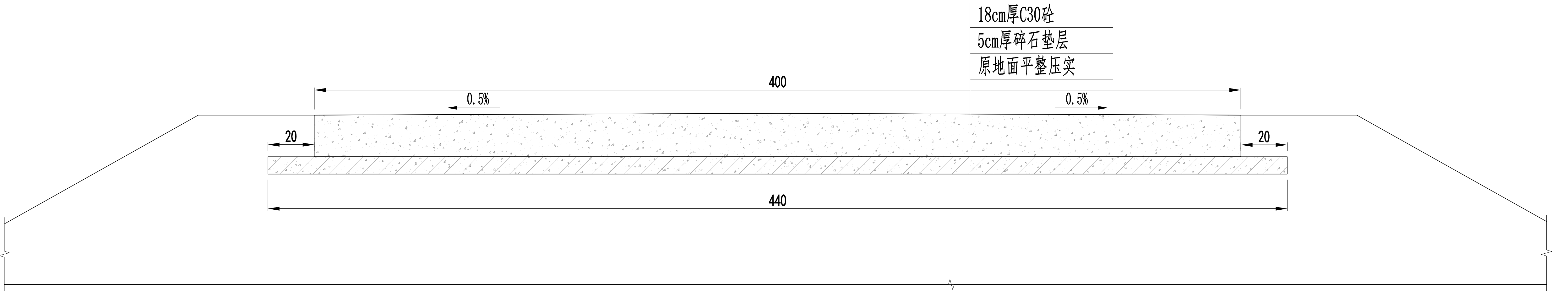
4. 0m宽18cm厚砼路面断面图 1:100
