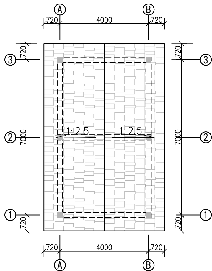
屋面平面图 1:100
