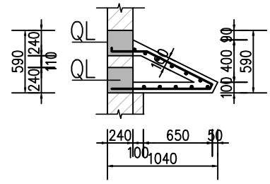
窗檐大样图 1:50
