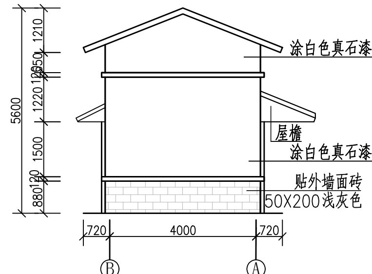
B-A侧立面图 1:100
