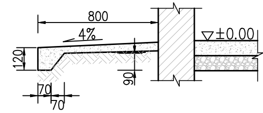
散水坡 1:25
