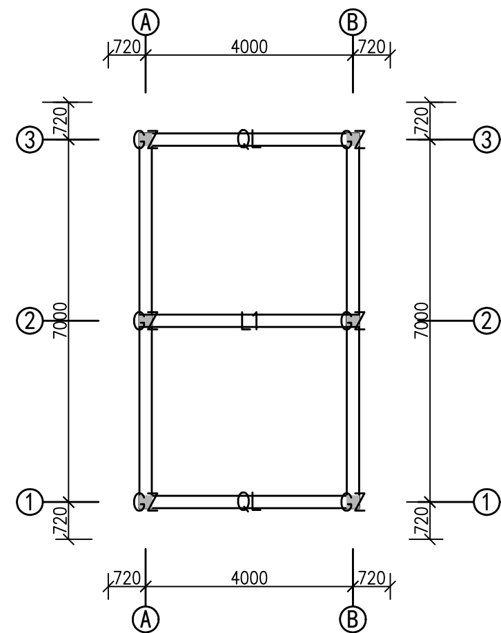
隔层平面图 1:100
