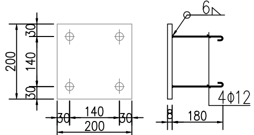
M1 1:25
