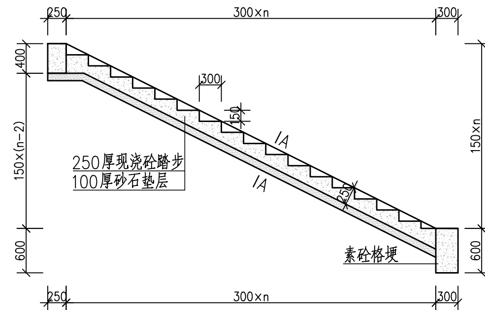
踏步纵剖视图 1:50
