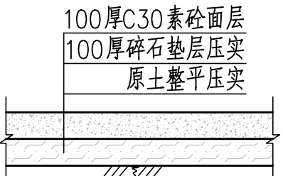
素砼场地 1:50
