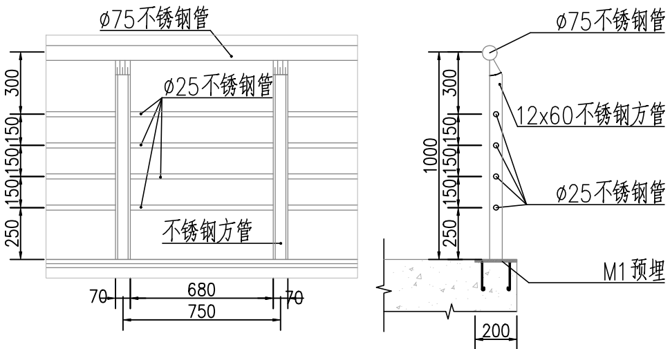
不锈钢栏杆结构图 1:25
