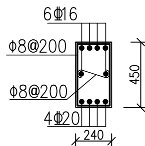
L1 1:25
