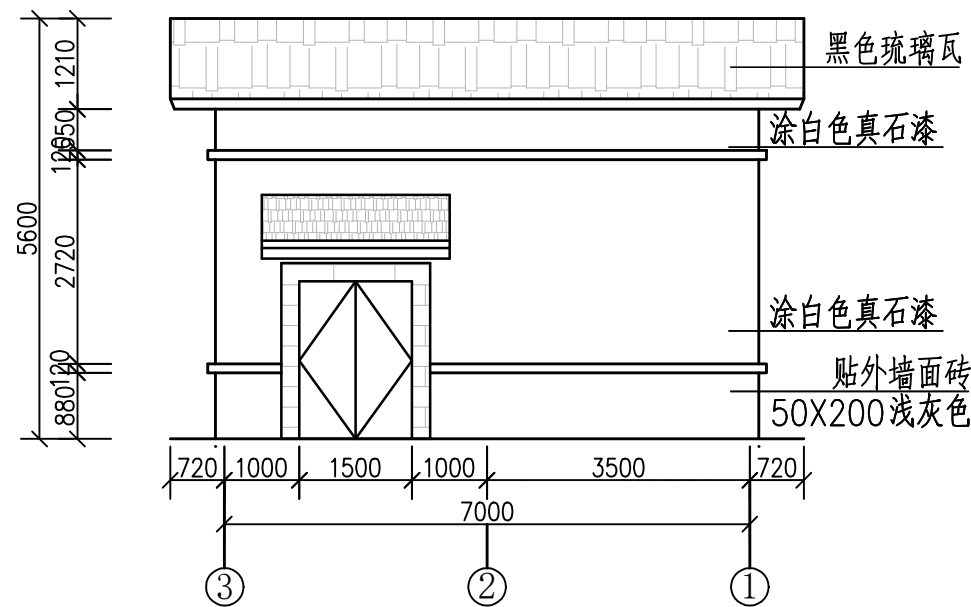
③-①立面图 1:100
