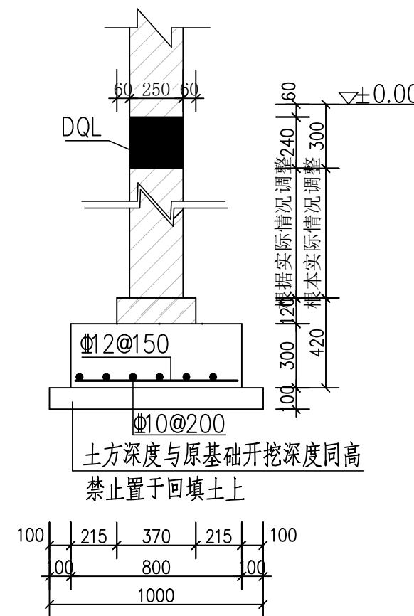
M-M 剖面图 1:25
