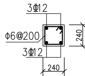
DQL 1:25
