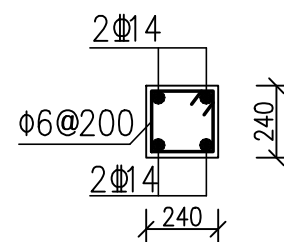
GZ 1:25
