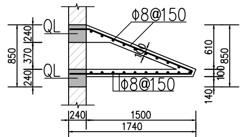
屋檐大样图 1:50
