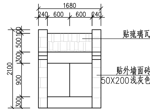
窗户立面图 1:50
