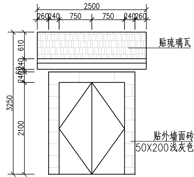
正门立面图 1:50
