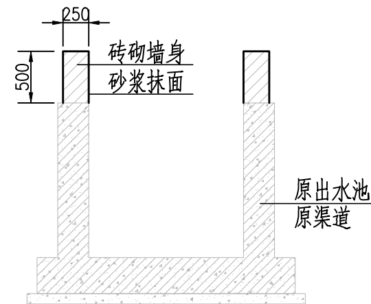
出水池、渠道加高 1:50
