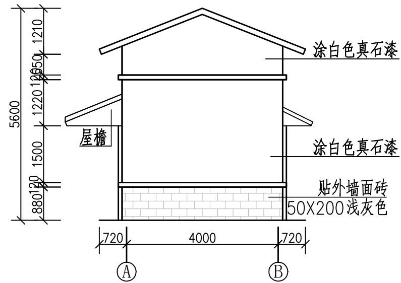
A-B侧立面图 1:100
