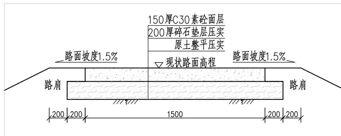
素砼道路 1:25
