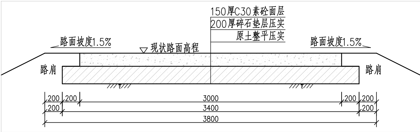
道路剖面图 1:25
