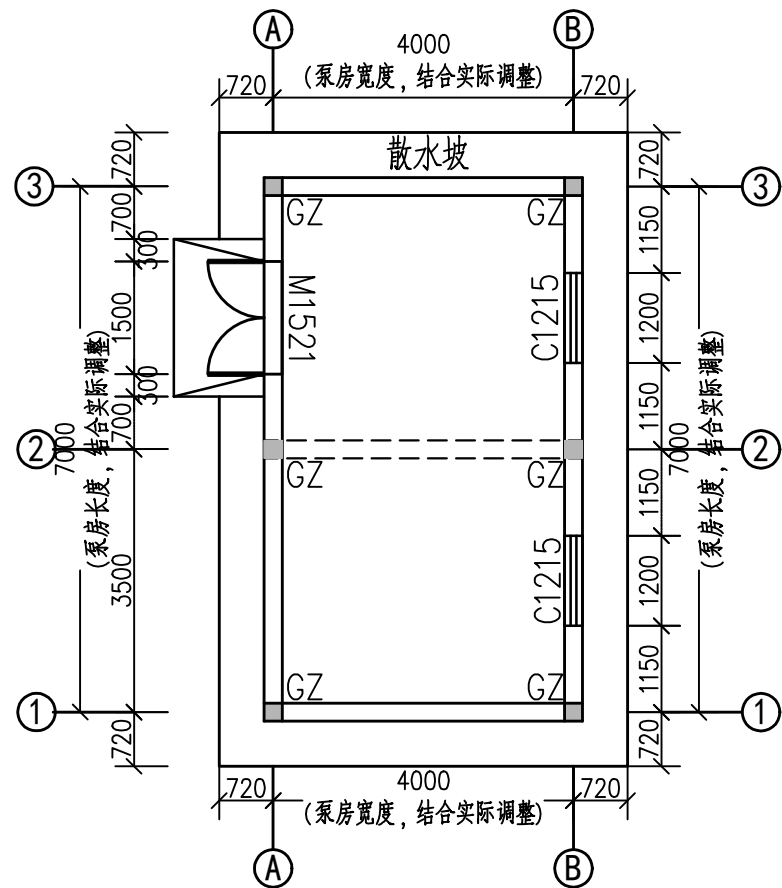
底层平面图 1:100
