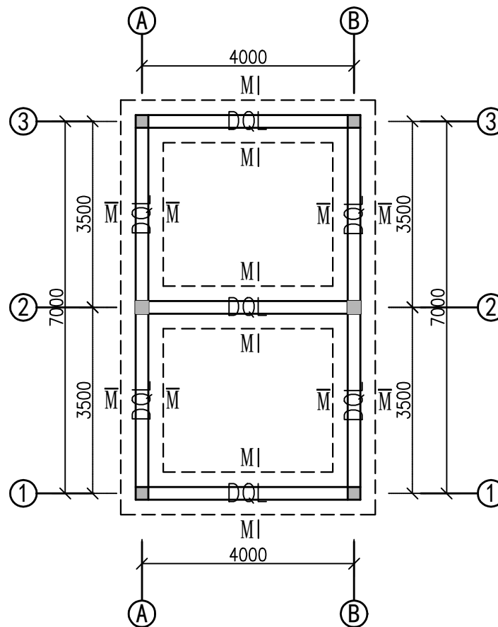
泵房基础平面图 1:100
