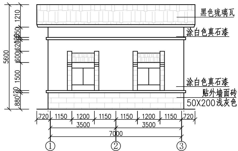
①-③立面图 1:100
