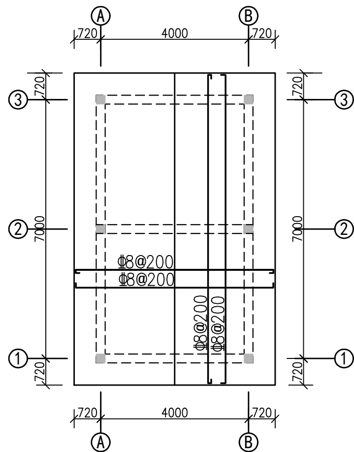
屋顶结构图 1:100
