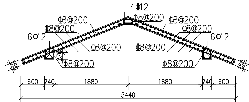
屋面配筋图 1:50
