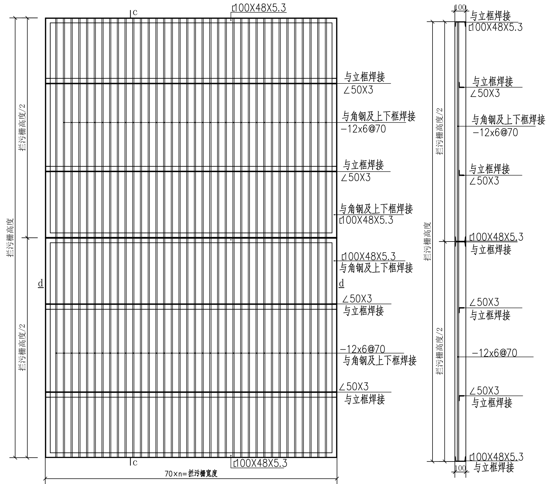
c-c 剖面结构图 1:50
