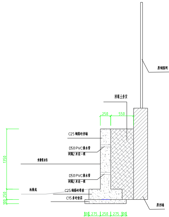
挡墙剖面图
