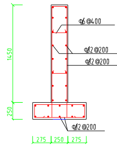
挡墙配筋图
