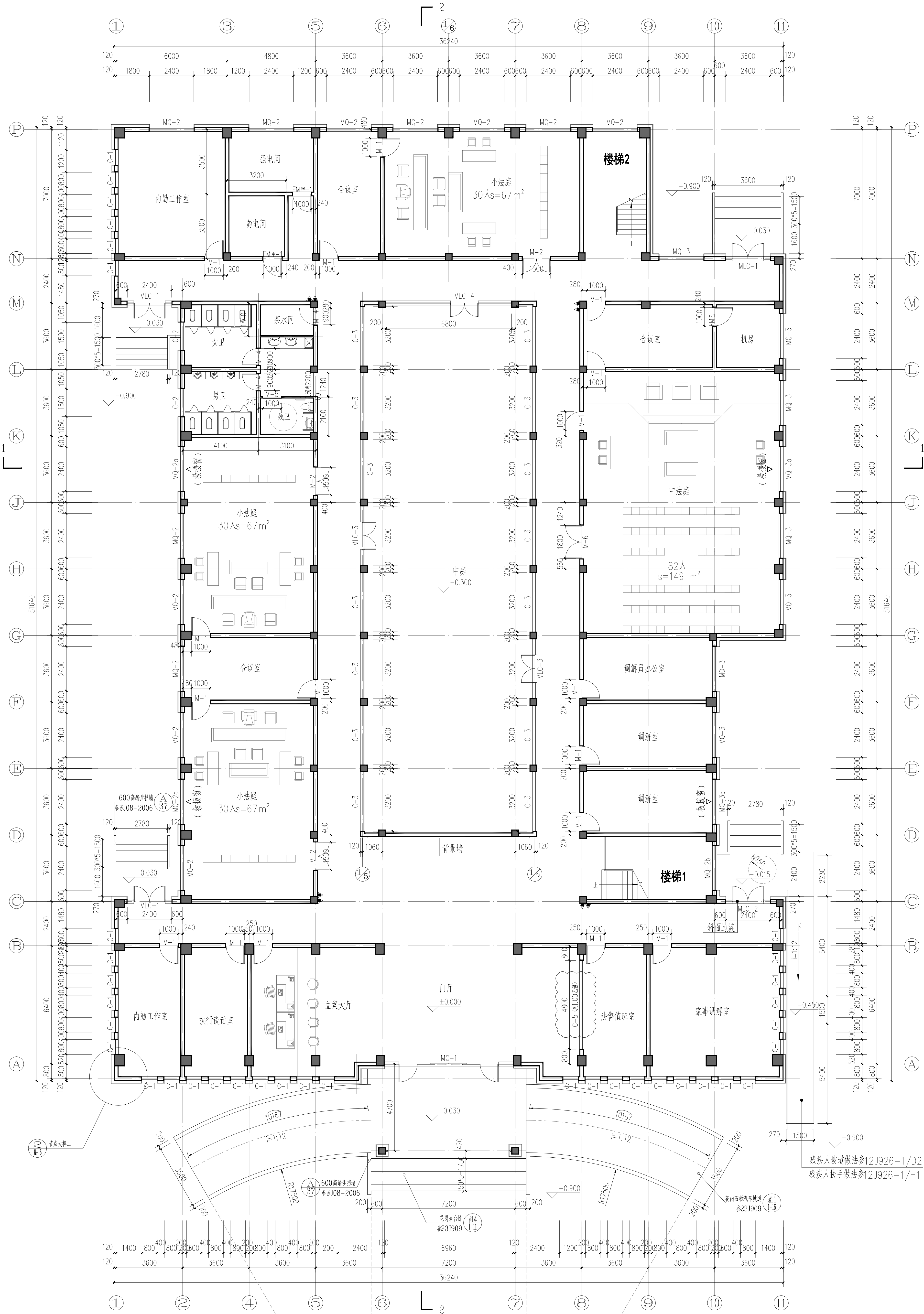
一层平面图 1:100
