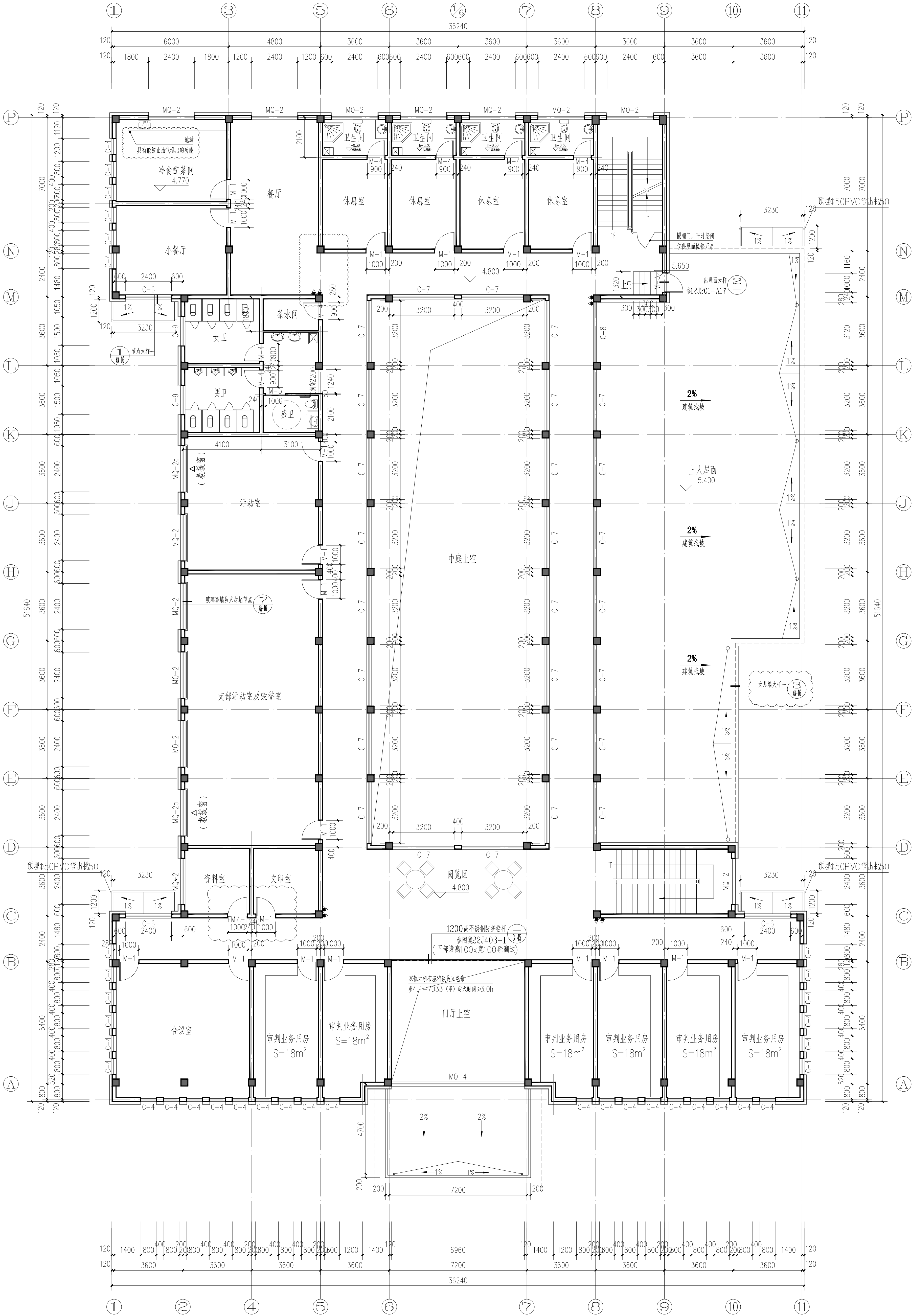
二层平面图 1:100
