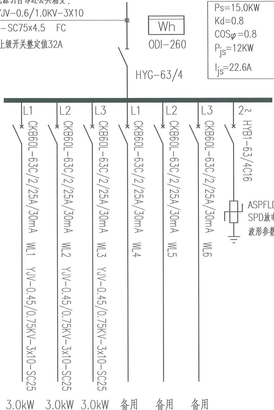
配电系统图
