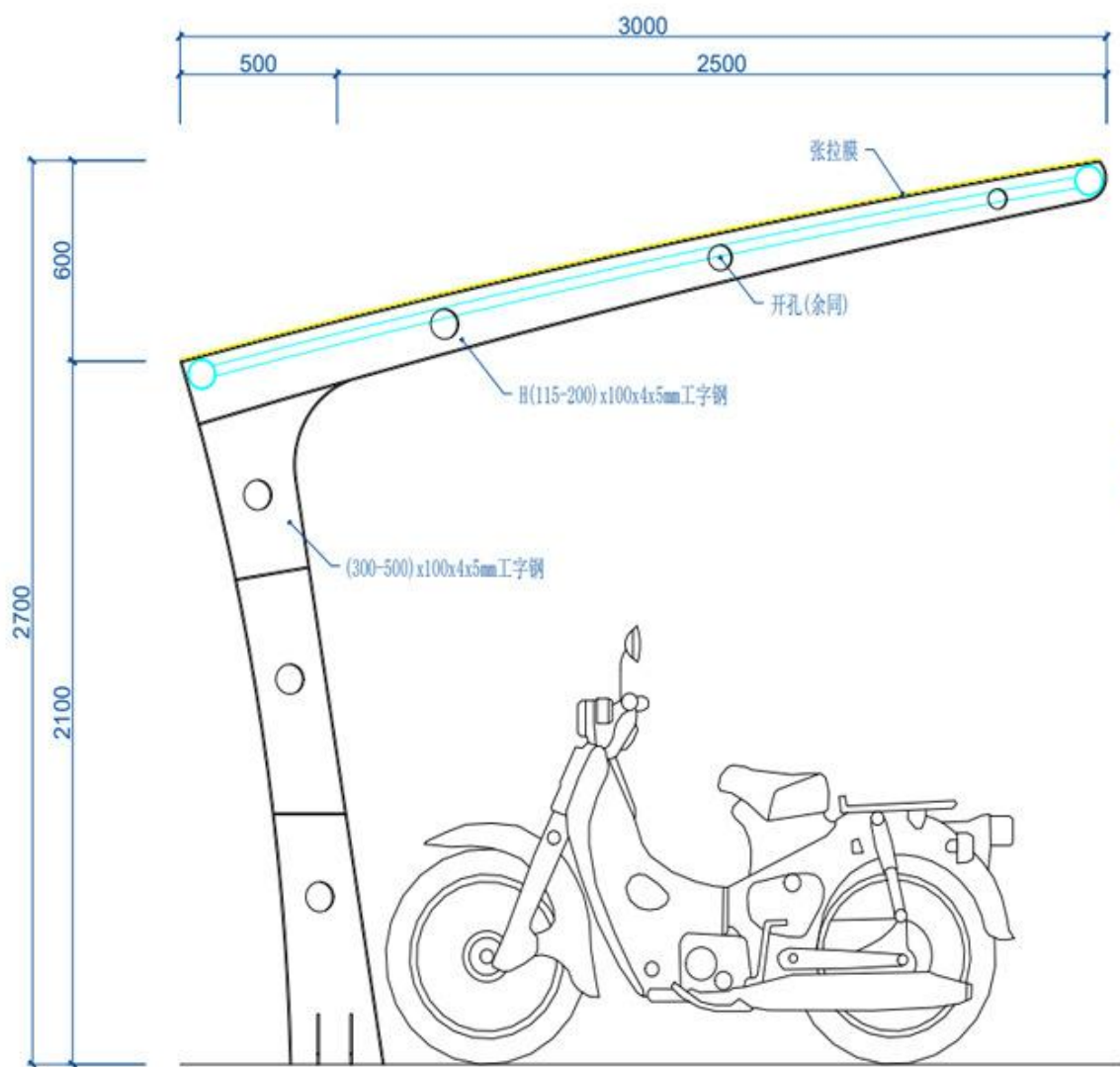
张拉膜节点图
