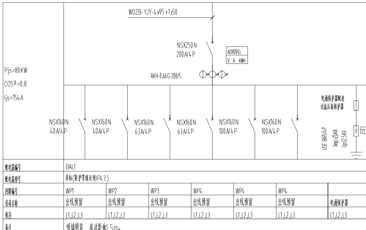
地下室配电间配电箱系统图
