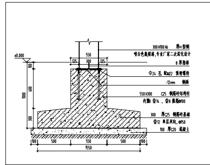
5 立柱基础A-A剖面图 SCALE 1:20
