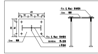
3 YMJ1大样图 SCALE 1:30
