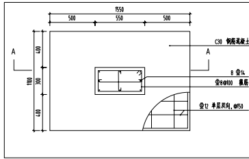
4 JC配筋图 SCALE 1:30
