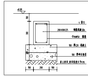
2 DL配筋图 SCALE 1:30
