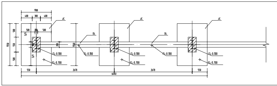
1 单轨动车棚—结构布置图 SCALE 1:30
