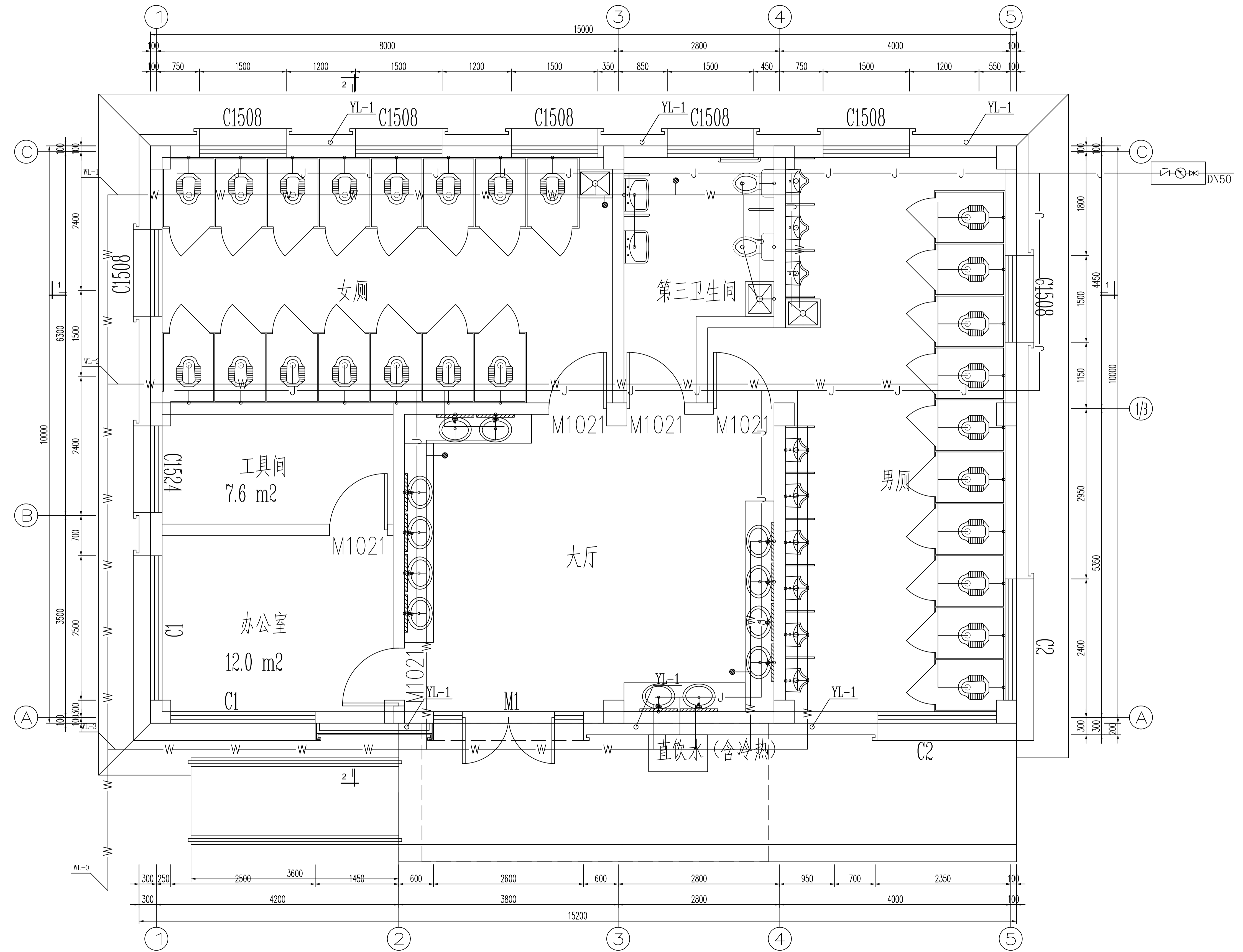
一层接地平面图 1:20
