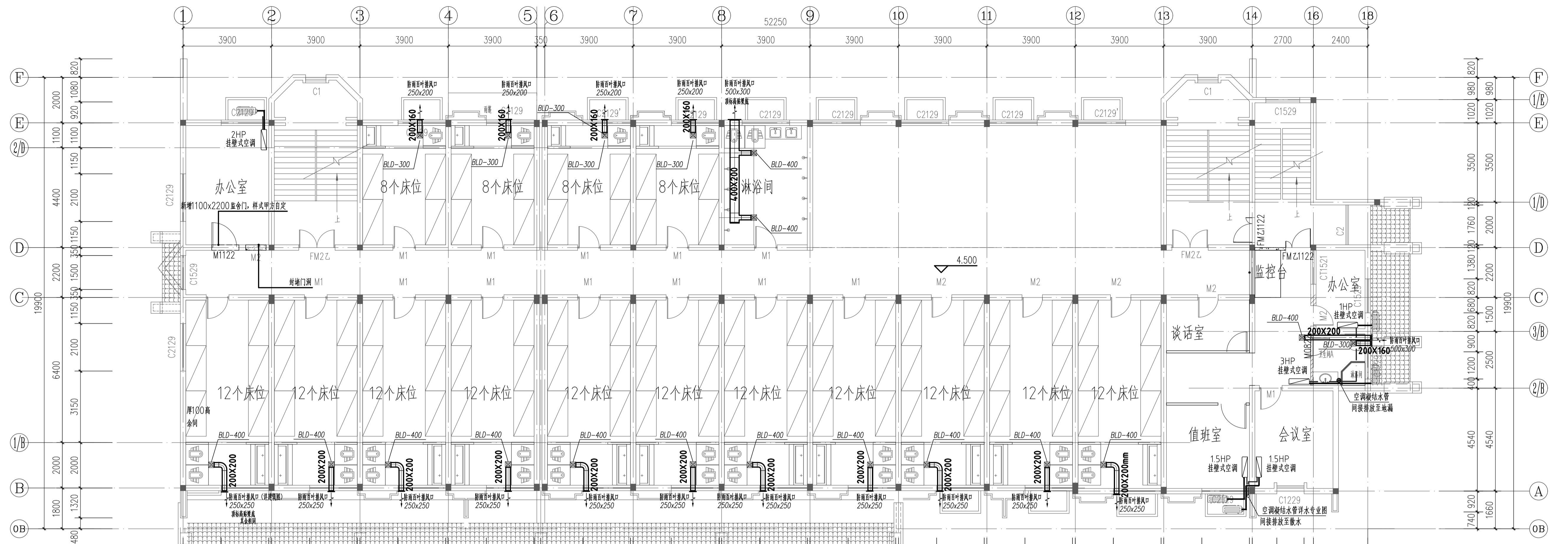
二层改造暖通平面图 1:100
