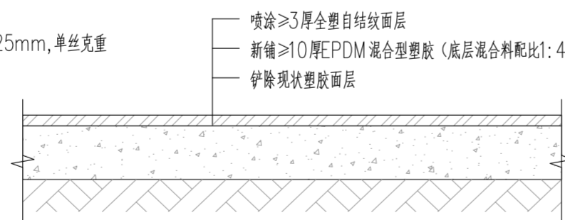
操场改造做法详图 1:10
