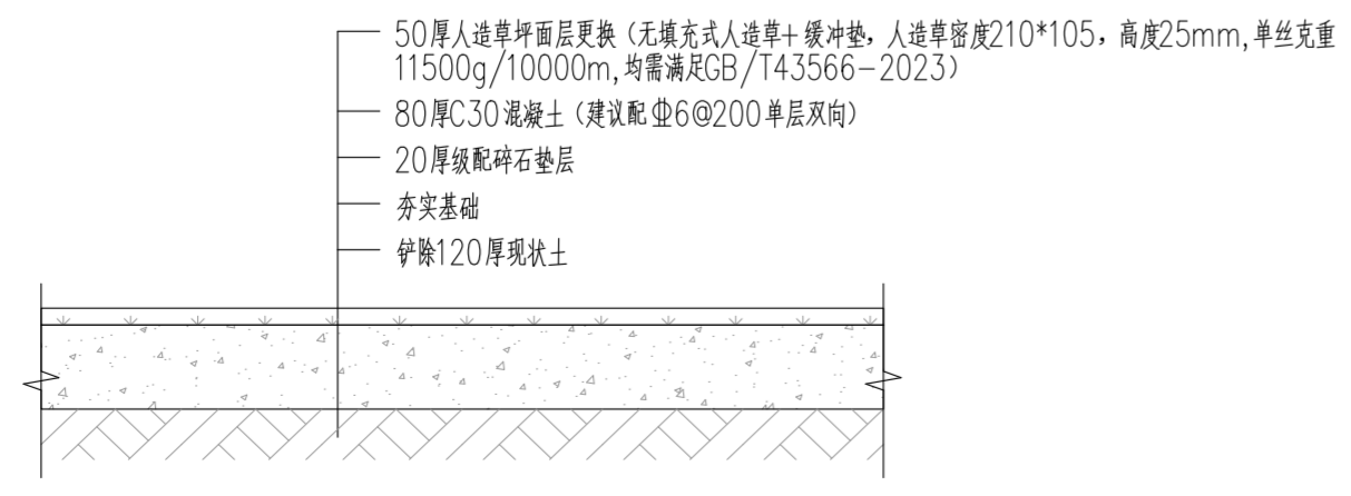
足球场改造做法详图 1:10
