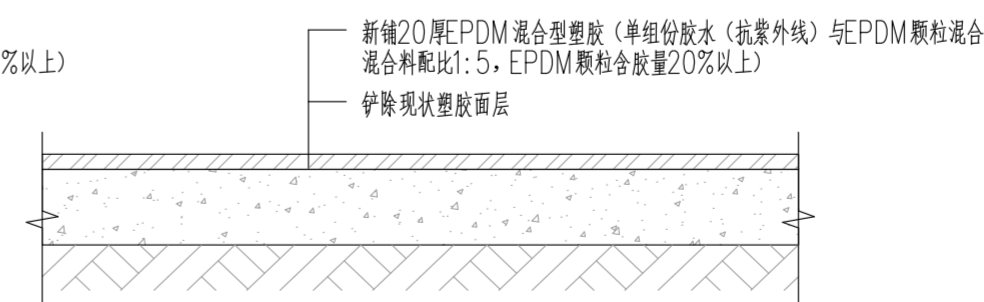
器械区地面改造做法详图 1:10
