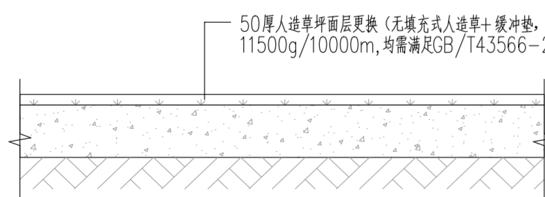
足球场改造做法详图 1:10
