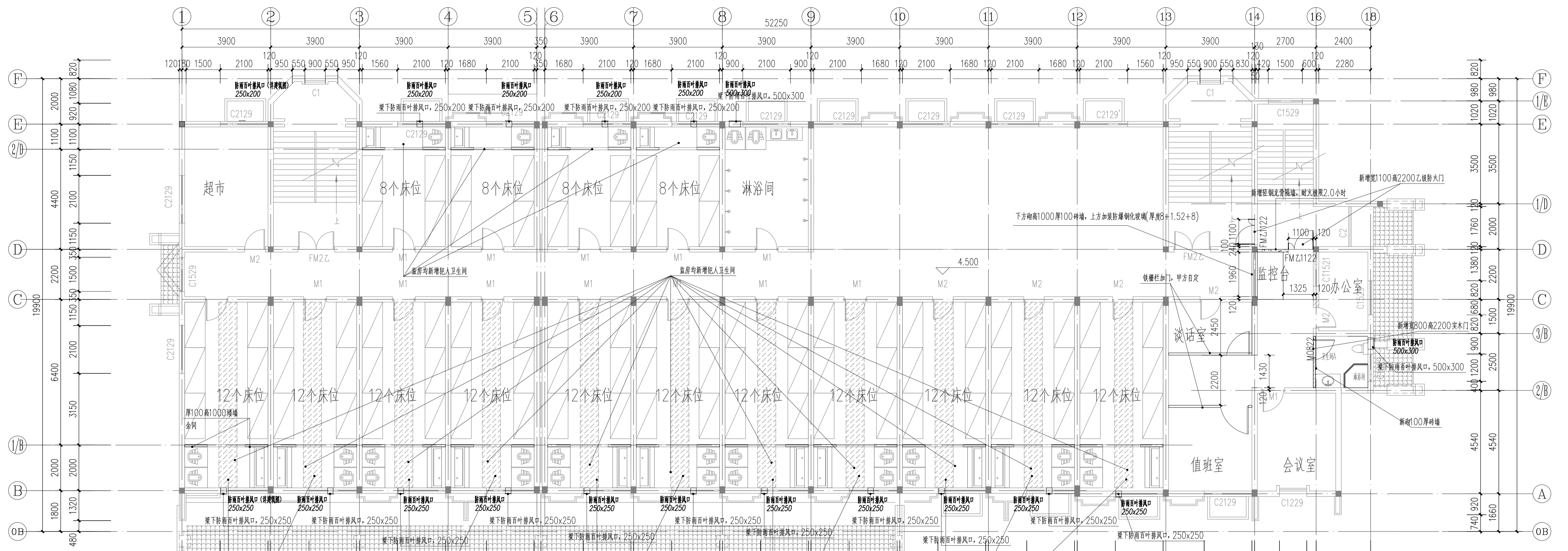
二层改造平面图 1:100
