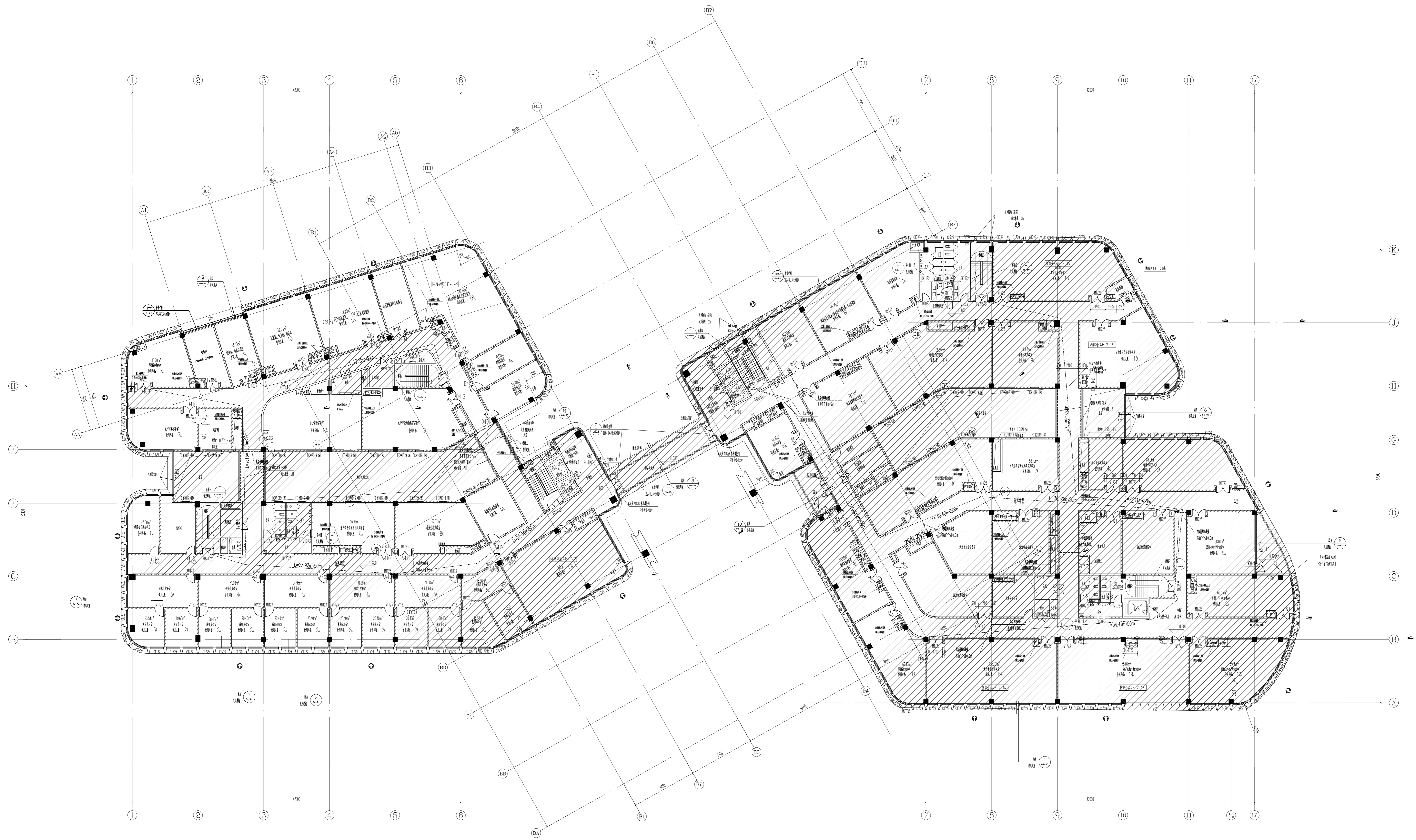
四层平面图 1:150 本层建筑面积: 5274.84平方米
