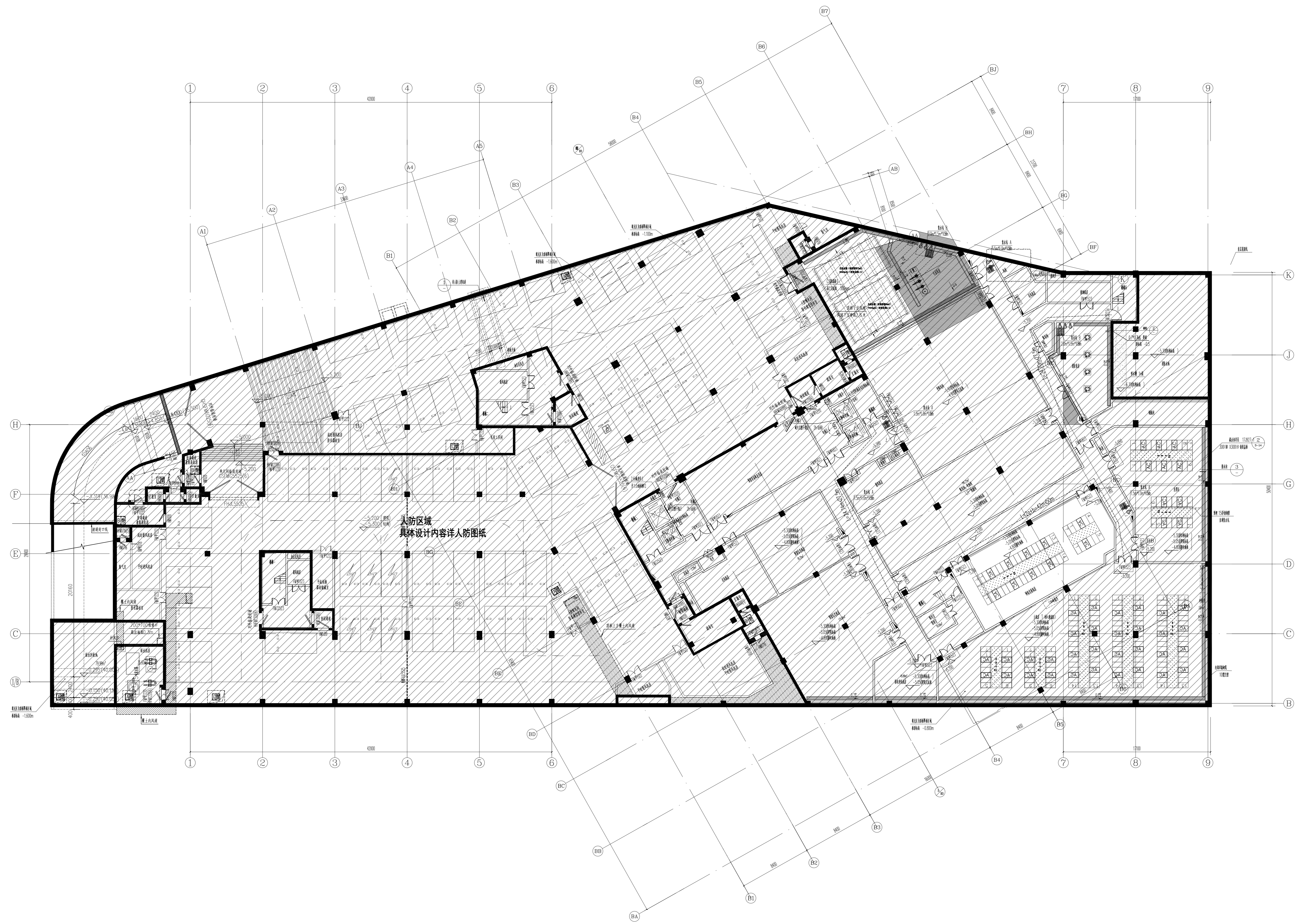
地下一层平面图 1:150 本层建筑面积: 6416.39平方米
