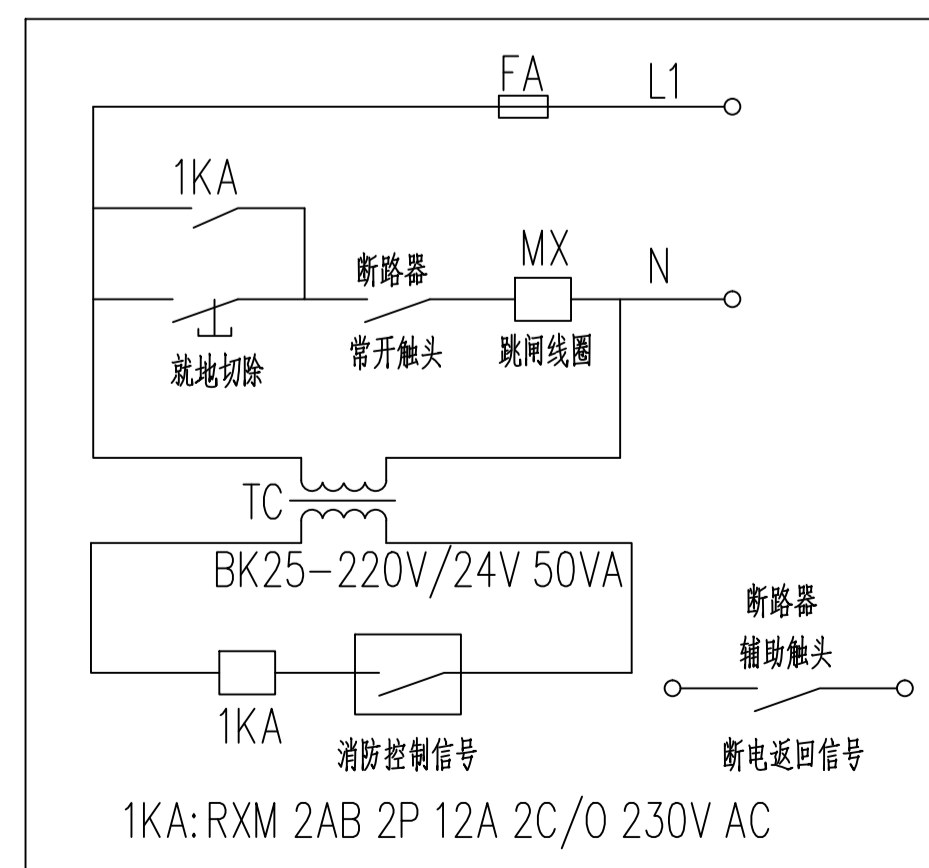
非消防电源切断控制原理图
