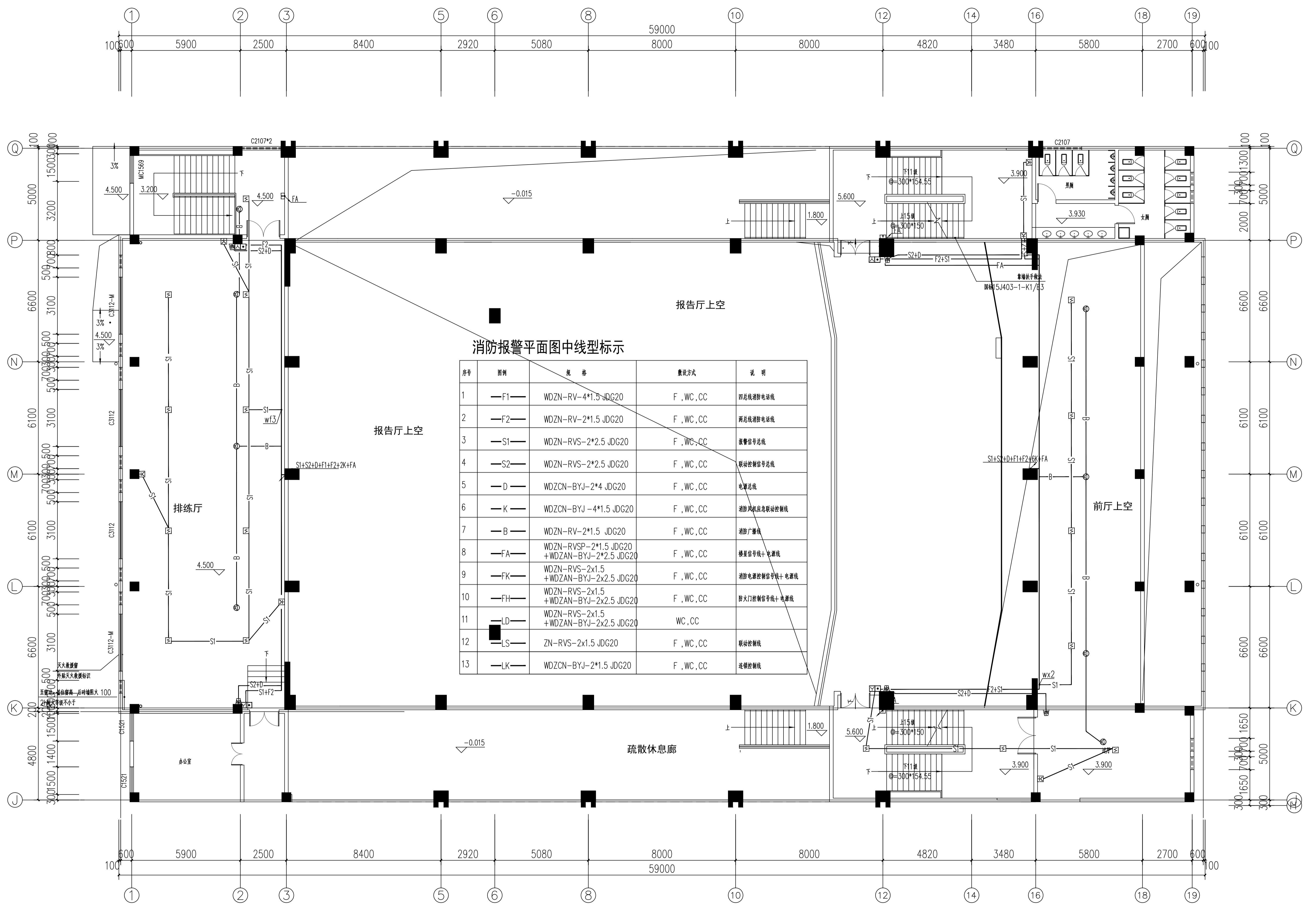
二层消防报警平面图 1:100
