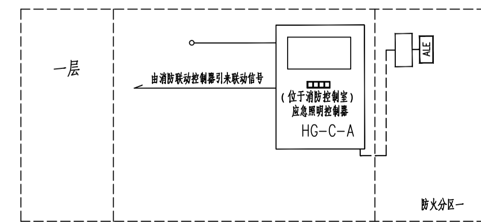
应急照明控制系统图
