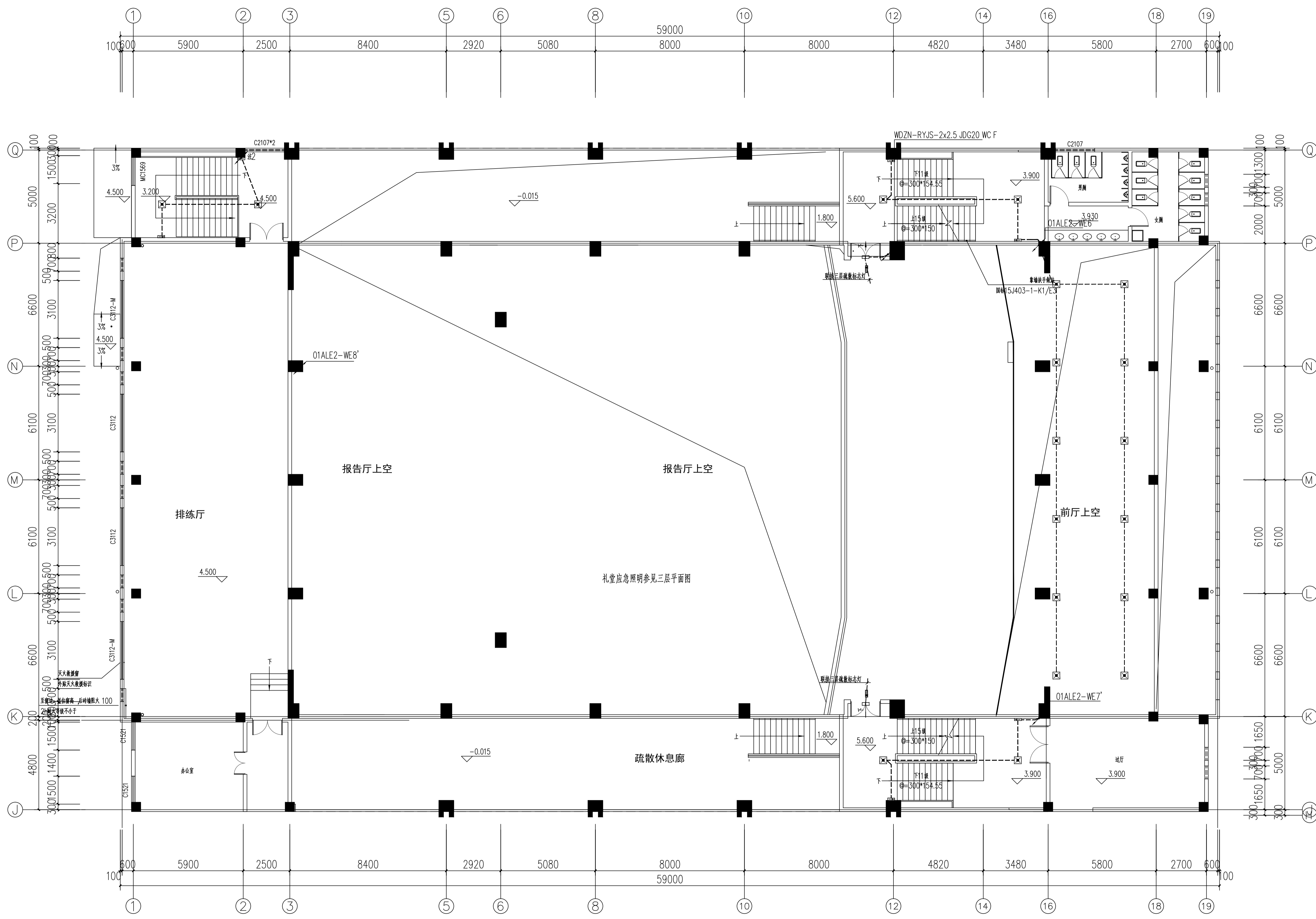
二层应急照明平面图 1:100
