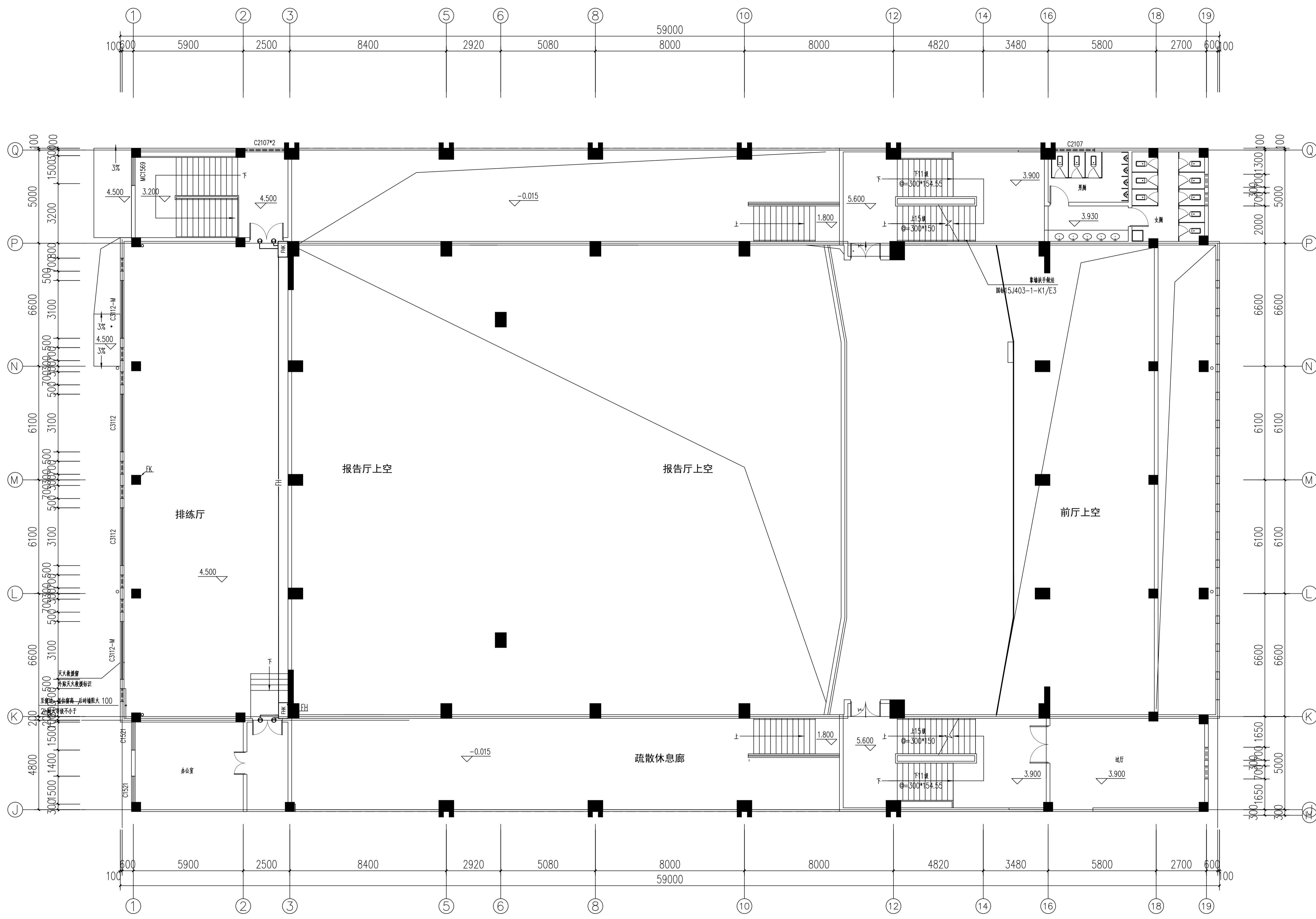
二层消防干线平面图 1:100
