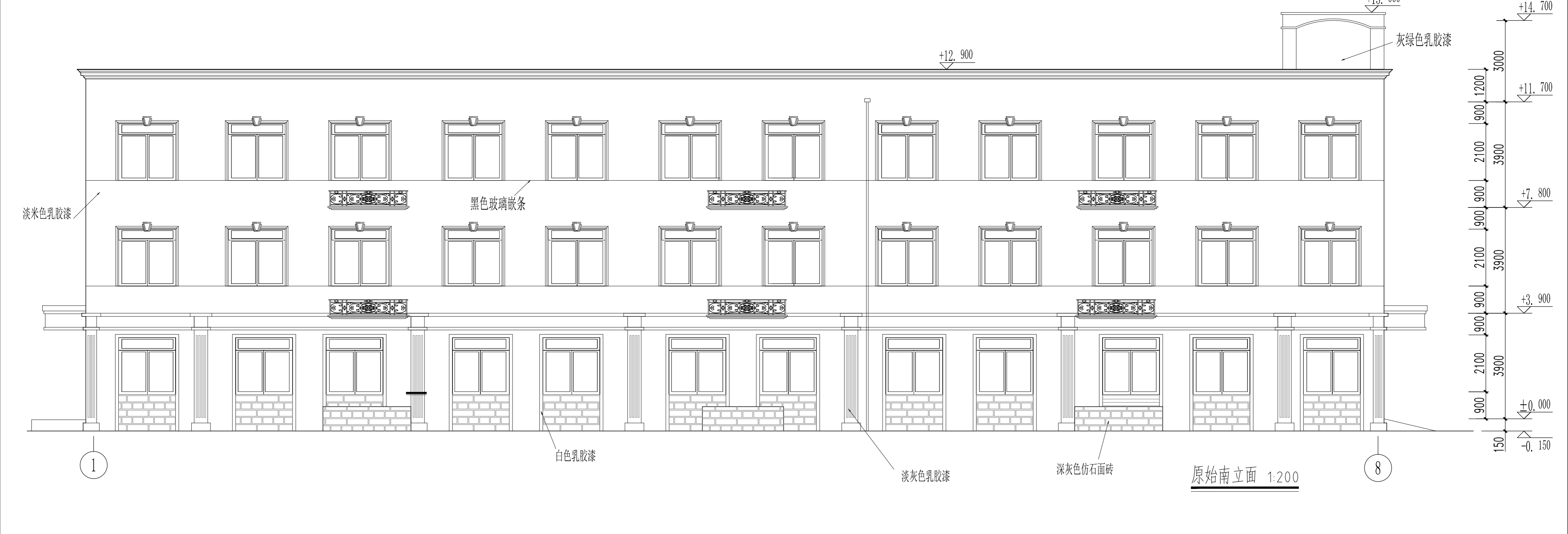
原始北立面 1:200
