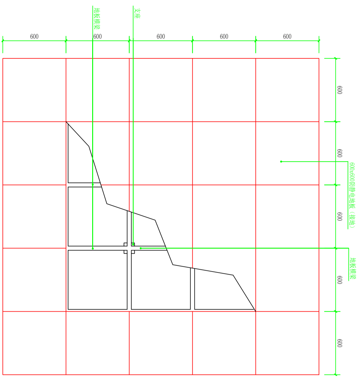
防静电地板铺设平面示意图 1:10
