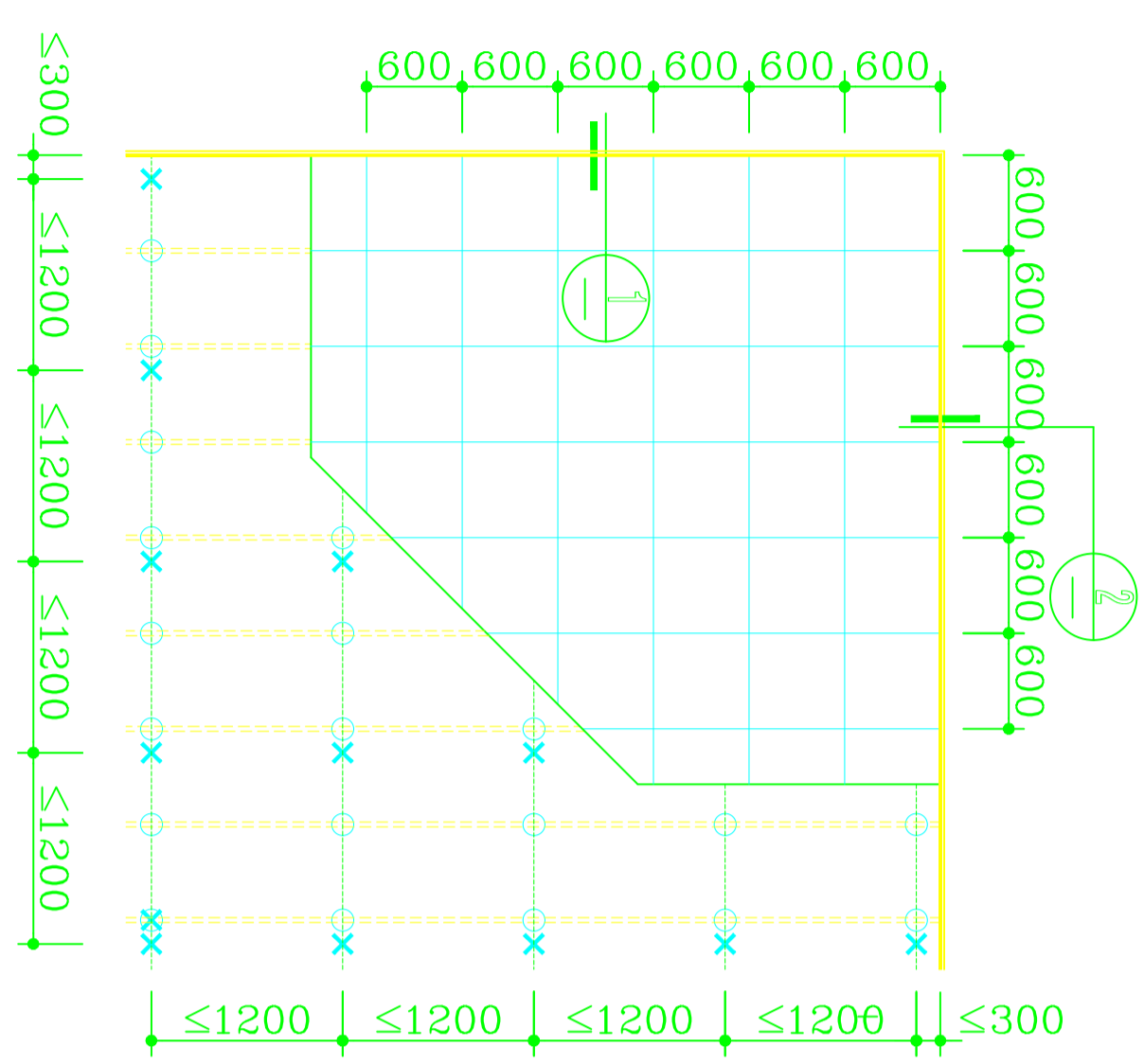
方块板与暗架龙骨组合图
