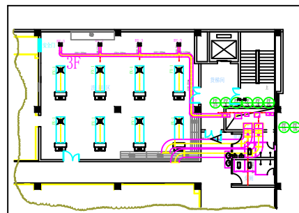
三层洗刷间夹层风机盘管平面
