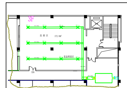
三层洗刷间夹层风管平面
