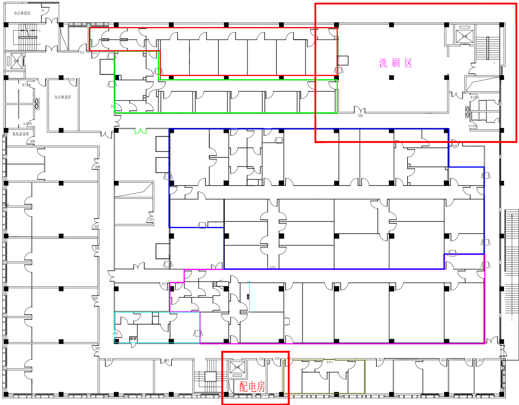
三层洗刷间→配电房平面
