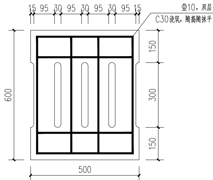
混凝土盖板配筋平面图 1:10
