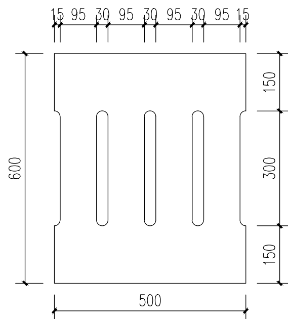
混凝土盖板平面图 1:10
