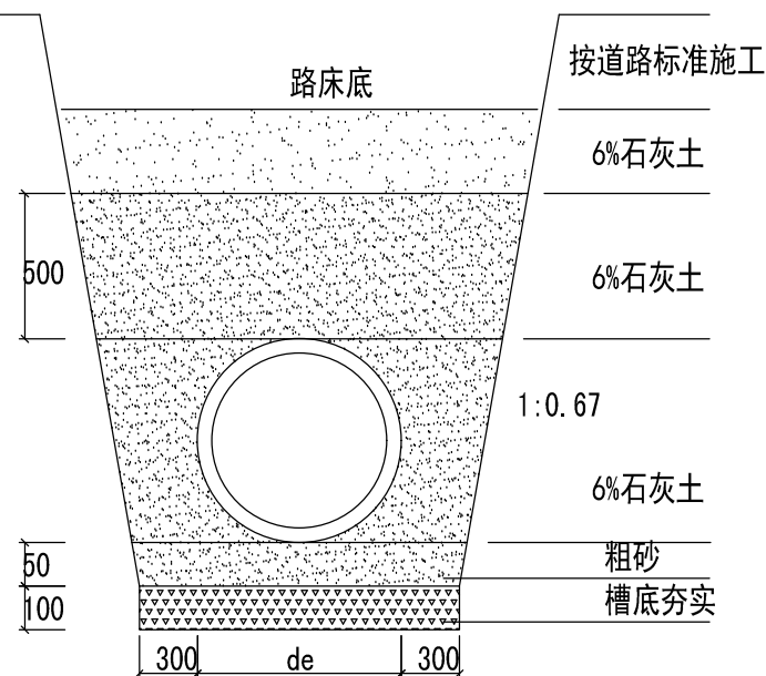
管道回填及基础图 1:20
