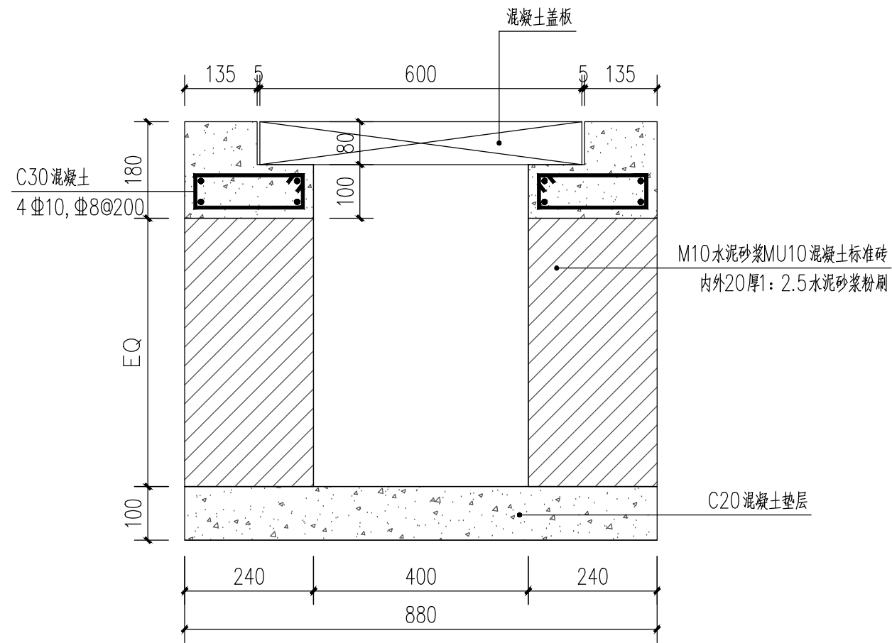
混凝土盖板明沟做法详图 1:10
