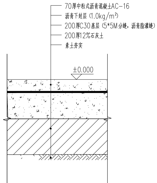
沥青场地恢复做法断面图 1:10
