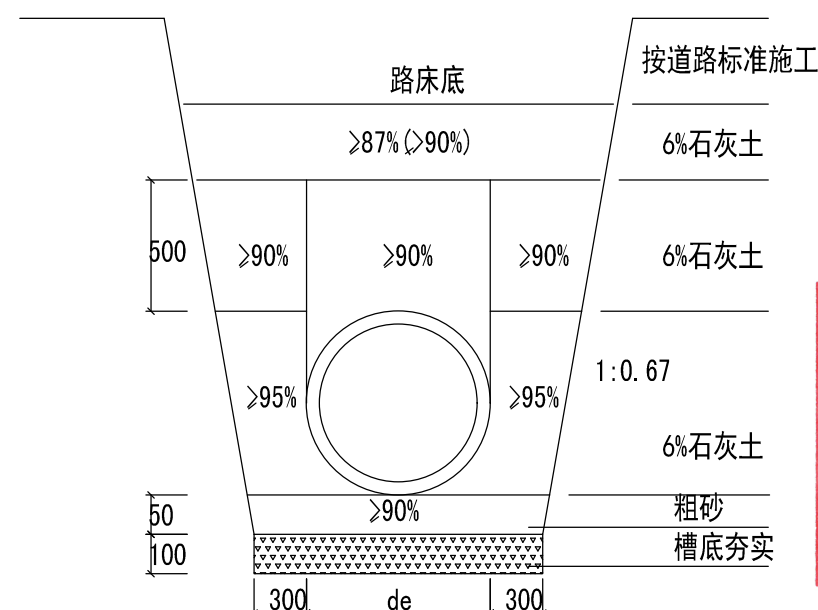
沟槽回填压实度要求示意图 1:20
