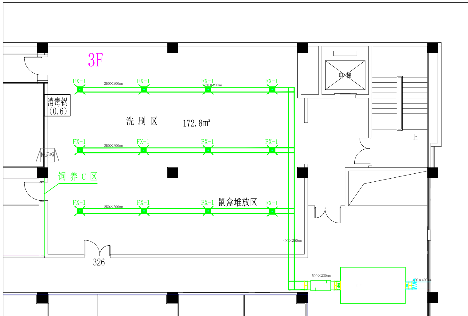
三层洗刷间夹层风管平面
