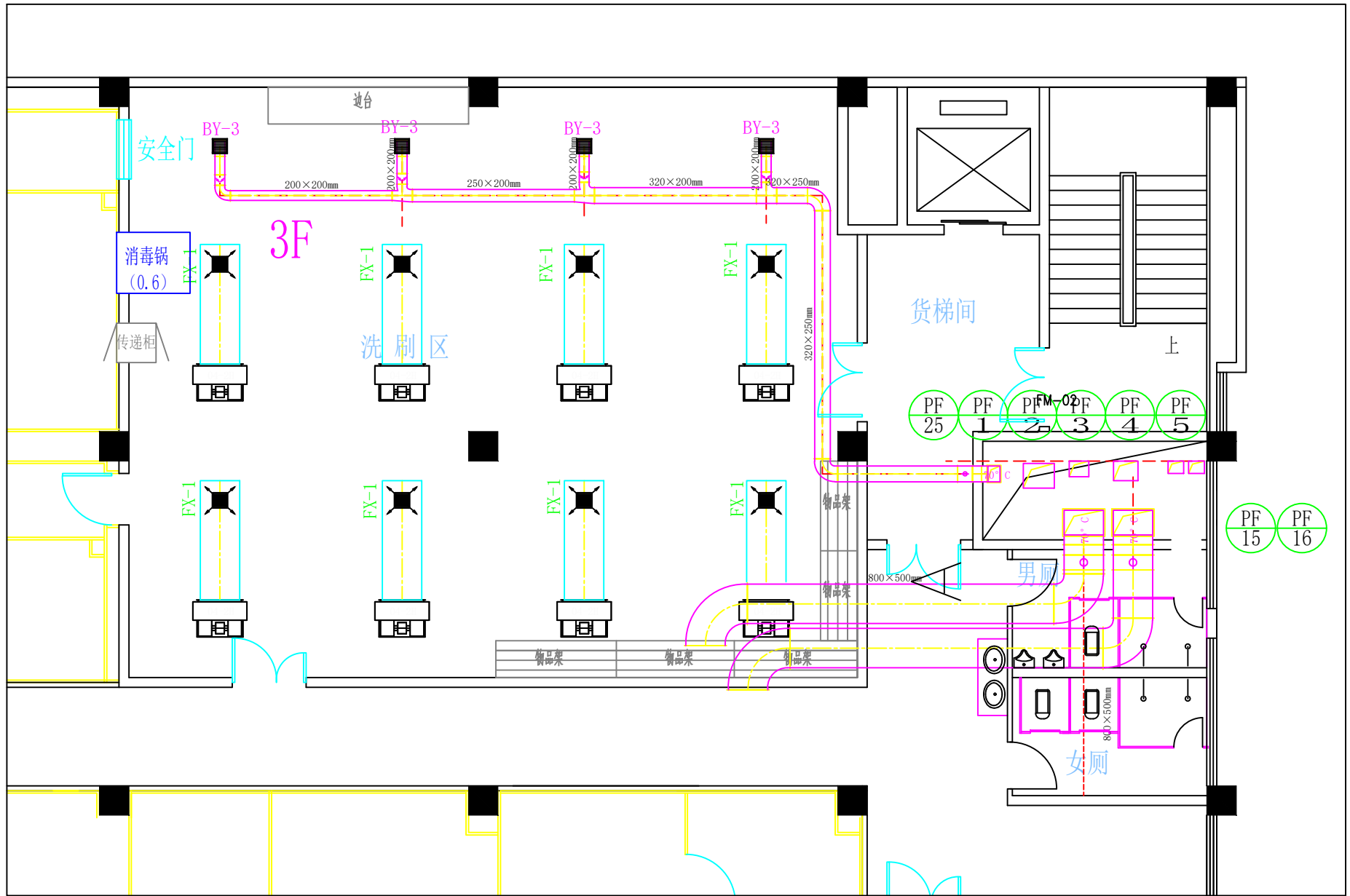
三层洗刷间夹层风机盘管平面
