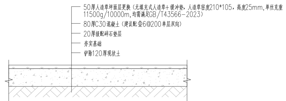
足球场改造做法详图 1:10
