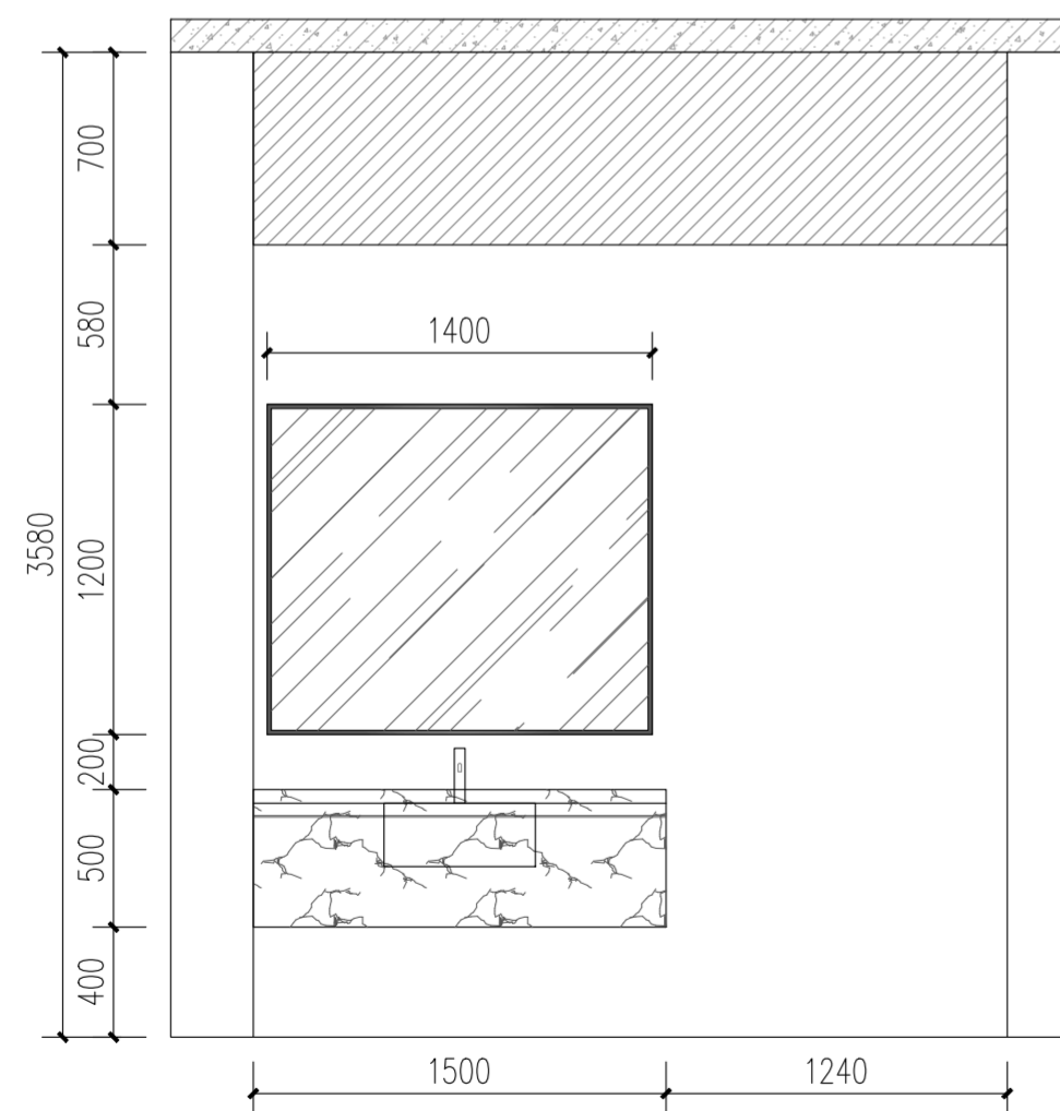
③ 公厕立面图C 1:30
