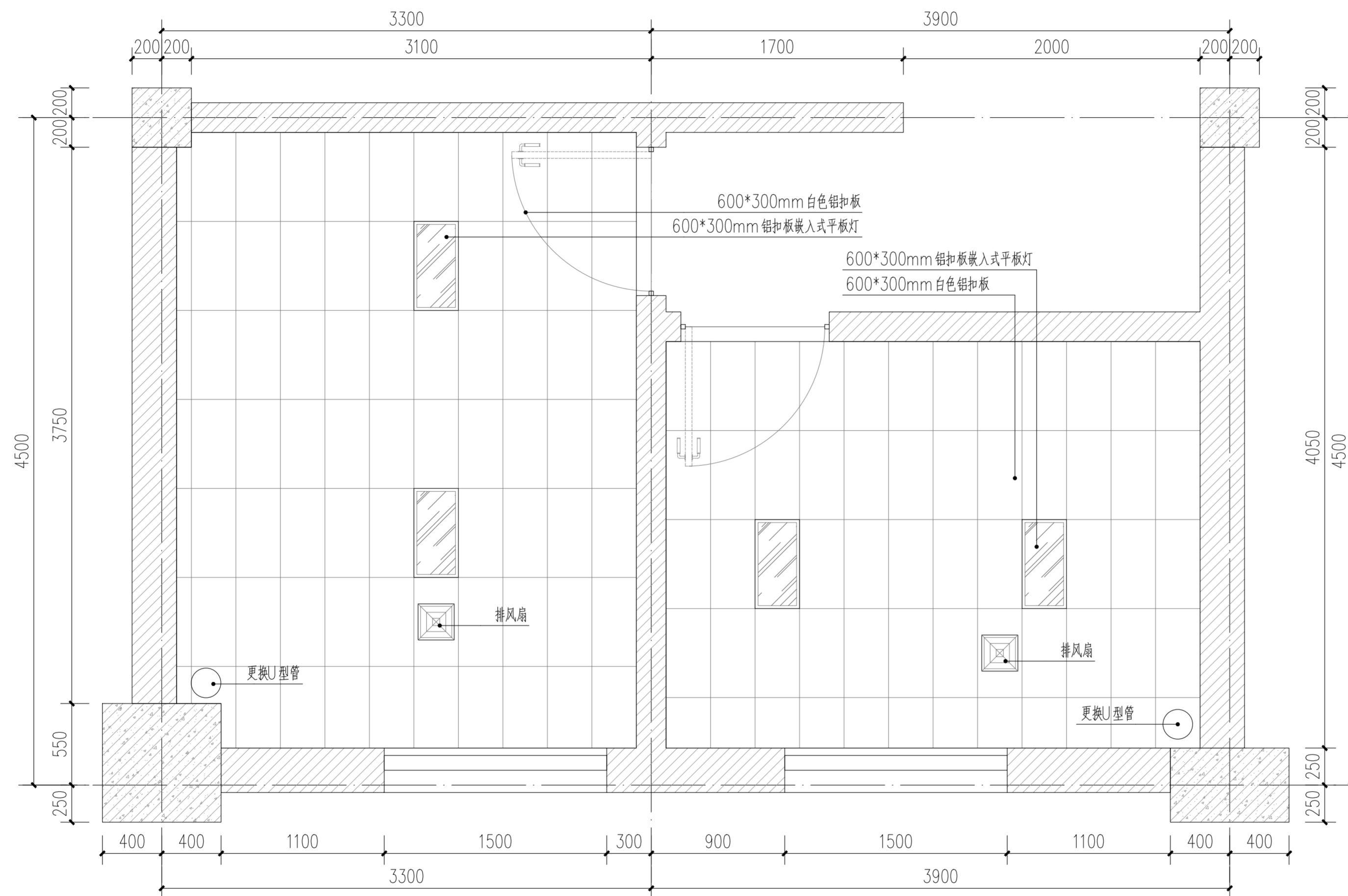
公厕一综合天花板平面图 1:30
