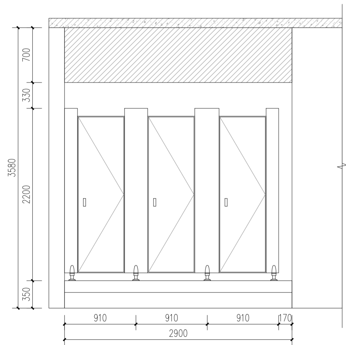
② 公厕立面图F 1:30
