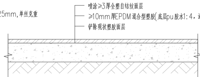
操场改造做法详图 1:10
