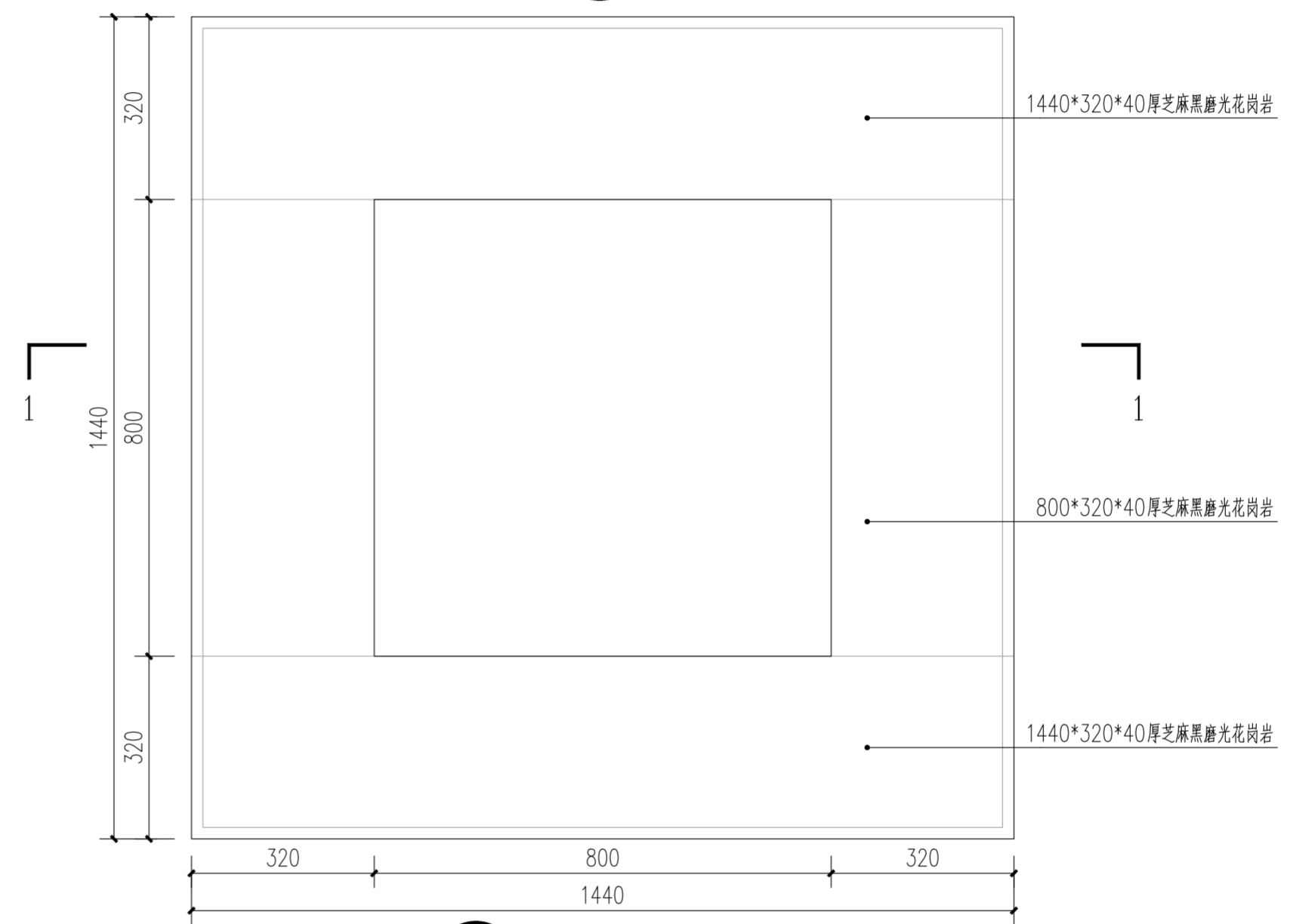
⑤ 树池平面图 1:10
