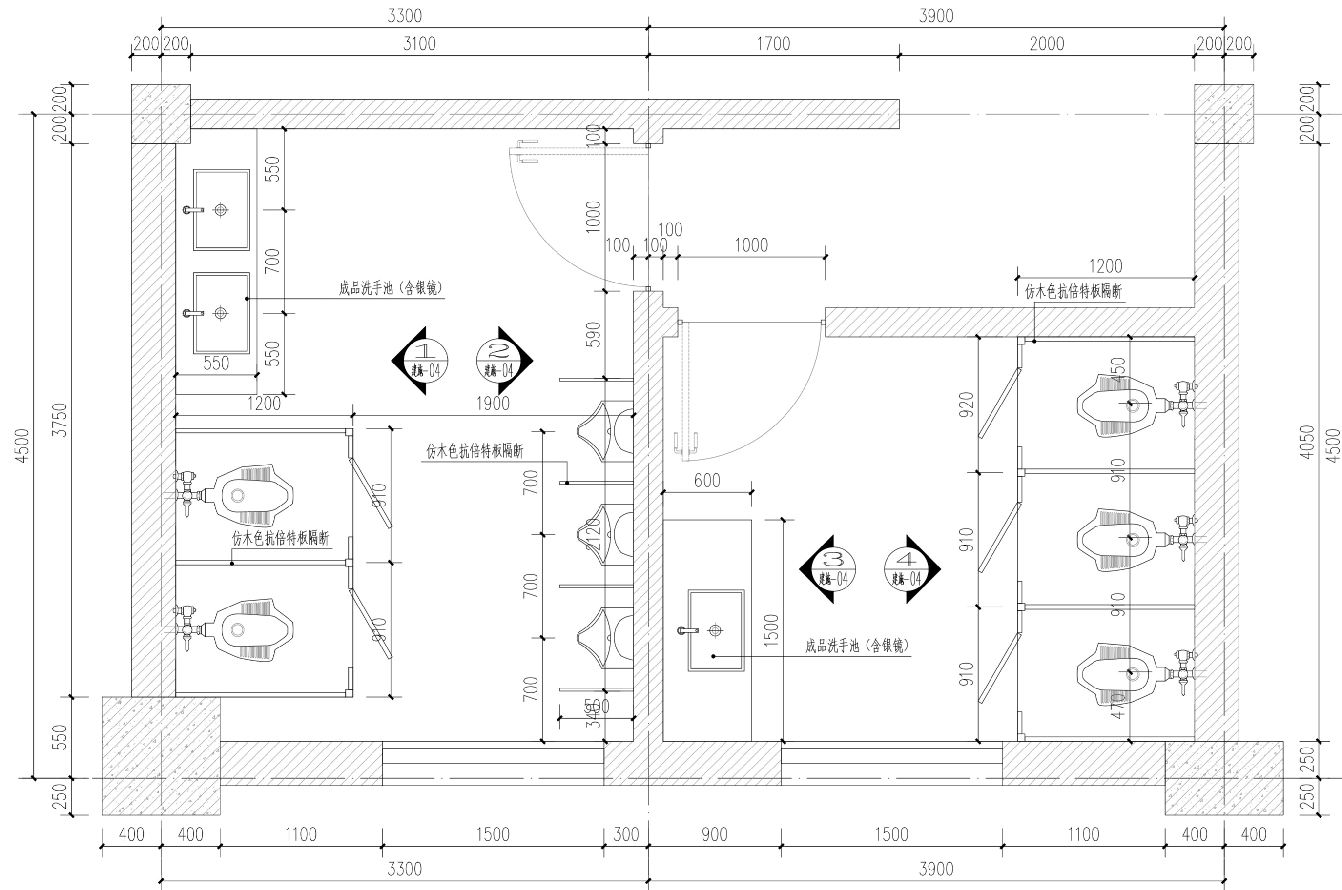
公厕一平面布置图 1:30
