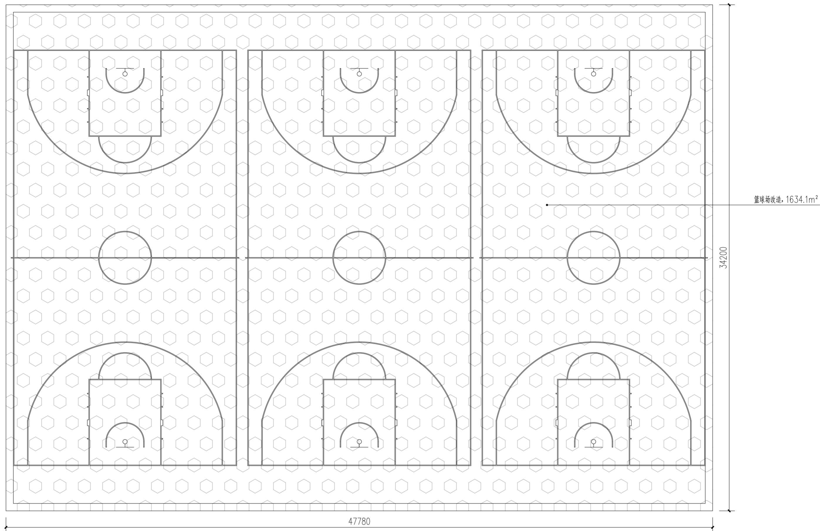
实验小学篮球场平面图 1:300
