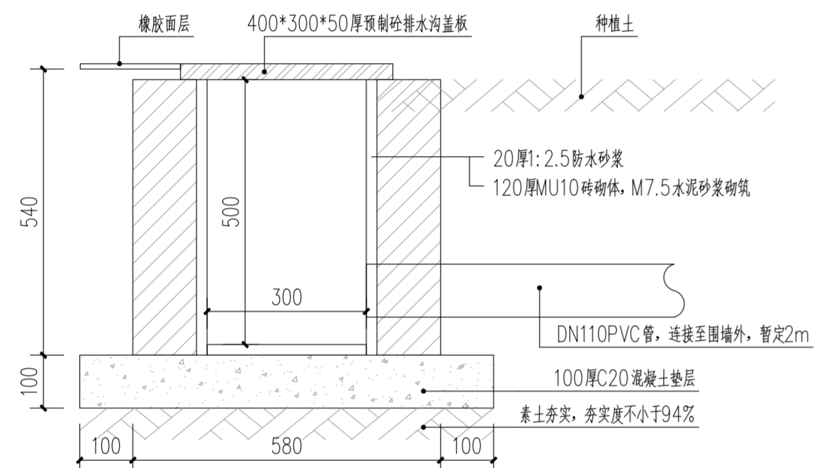
④ 新建排水沟做法详图 1:10
