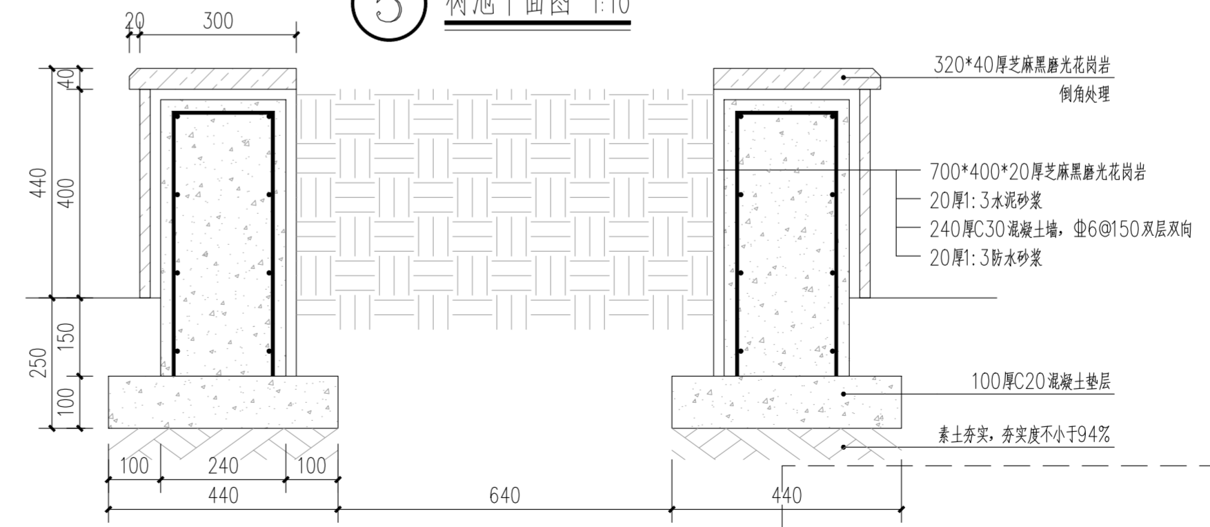
⑥ 1-1剖面图 1:10
