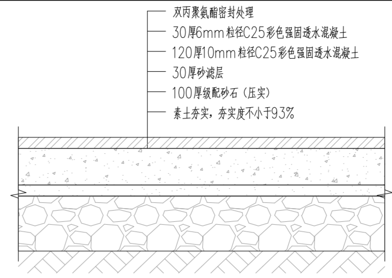
③ 彩色透水混凝土做法详图 1:10
