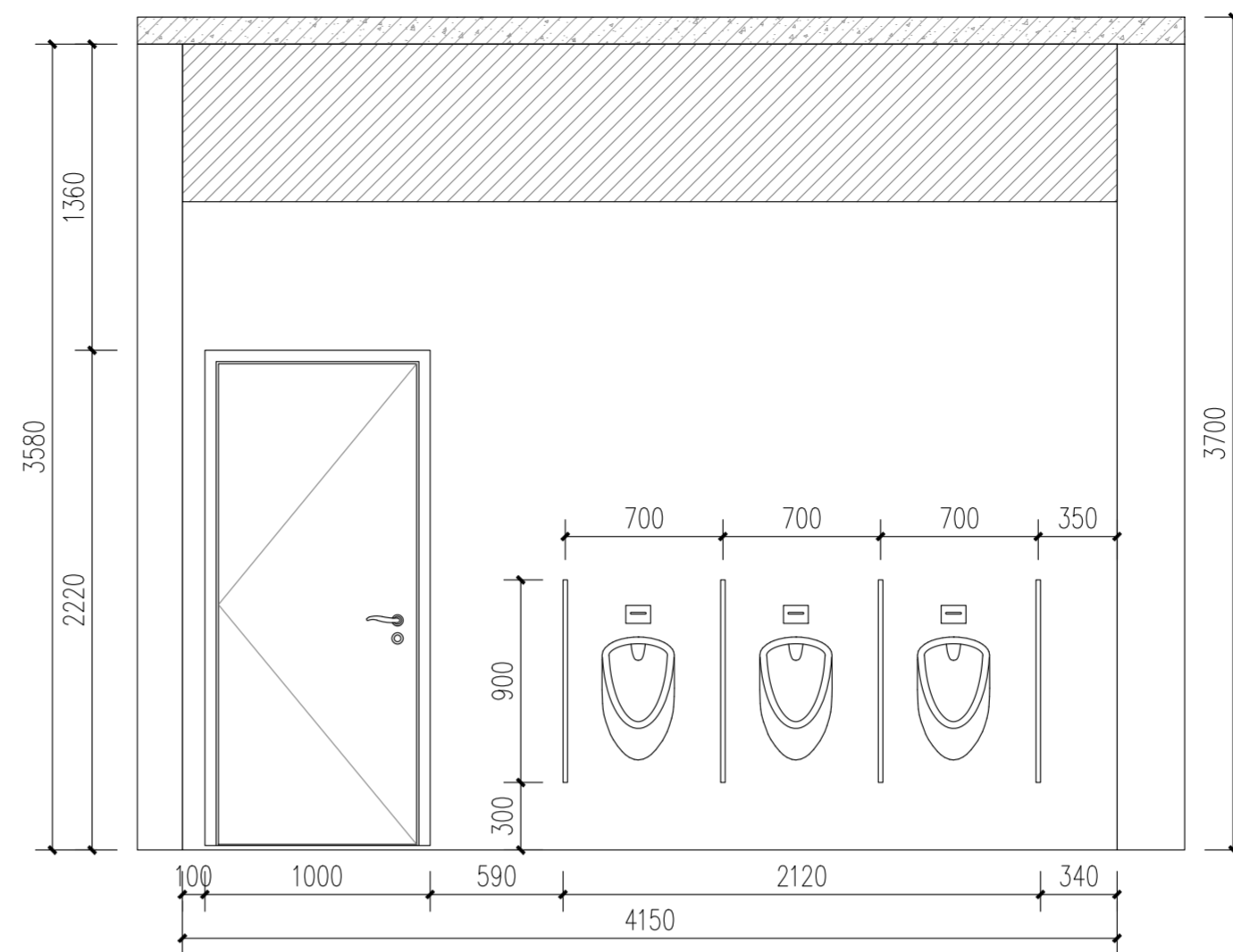
② 公厕立面图B 1:30
