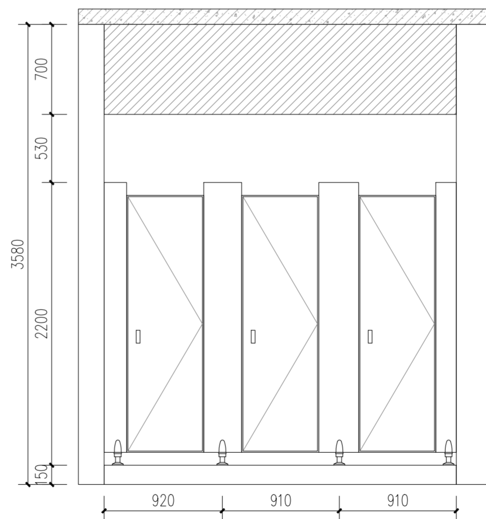
④ 公厕立面图D 1:30
