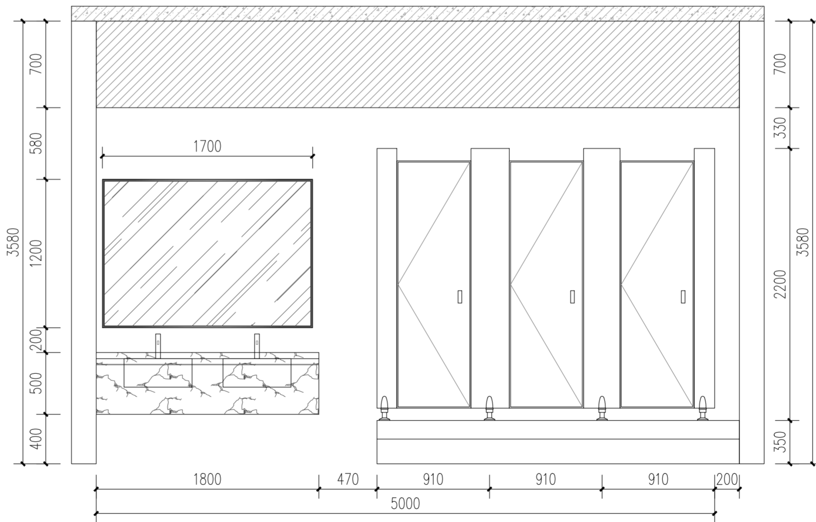
③ 公厕立面图G 1:30
