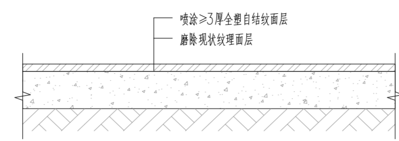
② 操场改造做法详图 1:10
