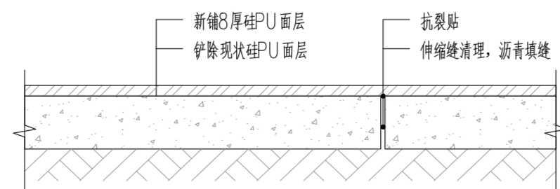
篮球场改造做法详图 1:10
