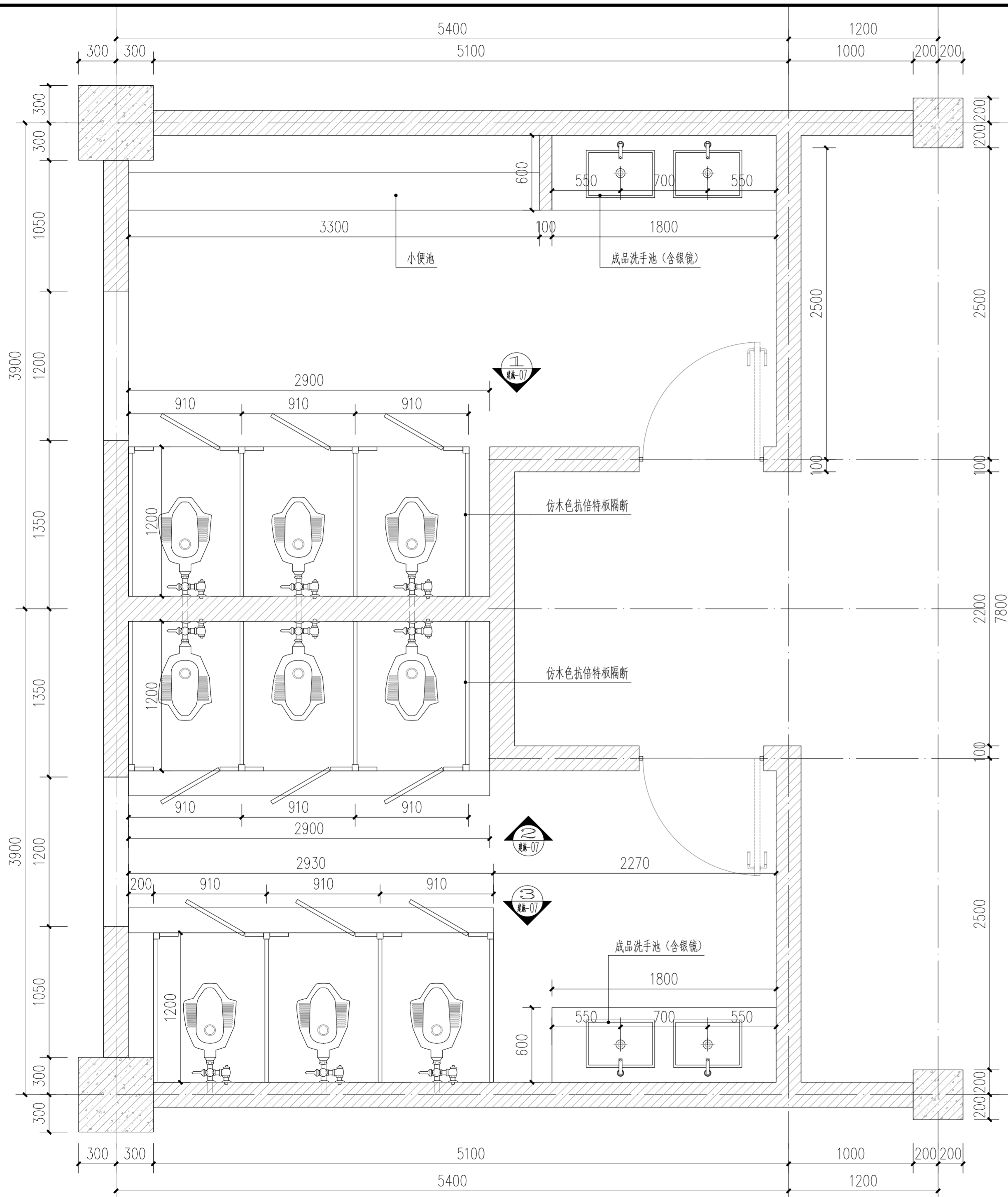
公厕二平面布置图 1:30
