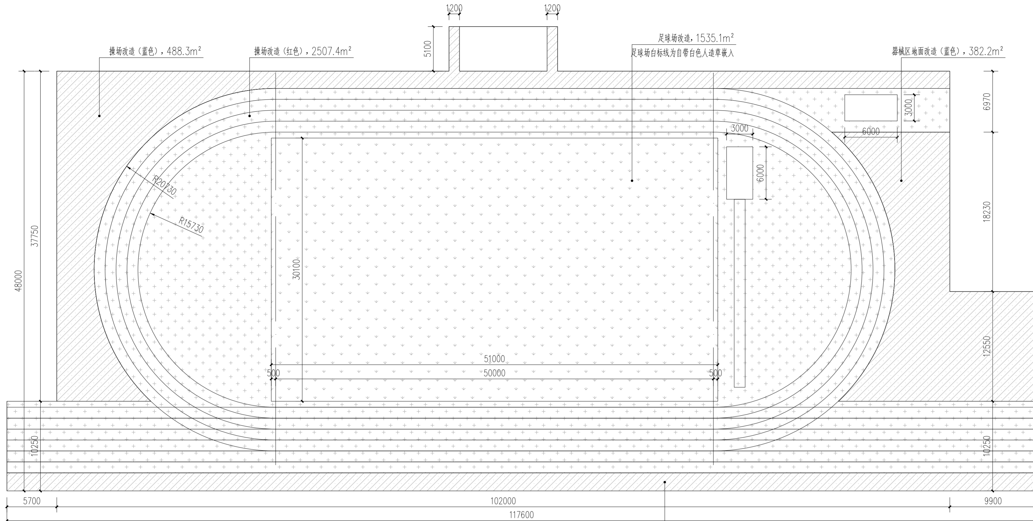
实验小学操场平面图 1:300
