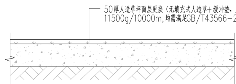
足球场改造做法详图 1:10
