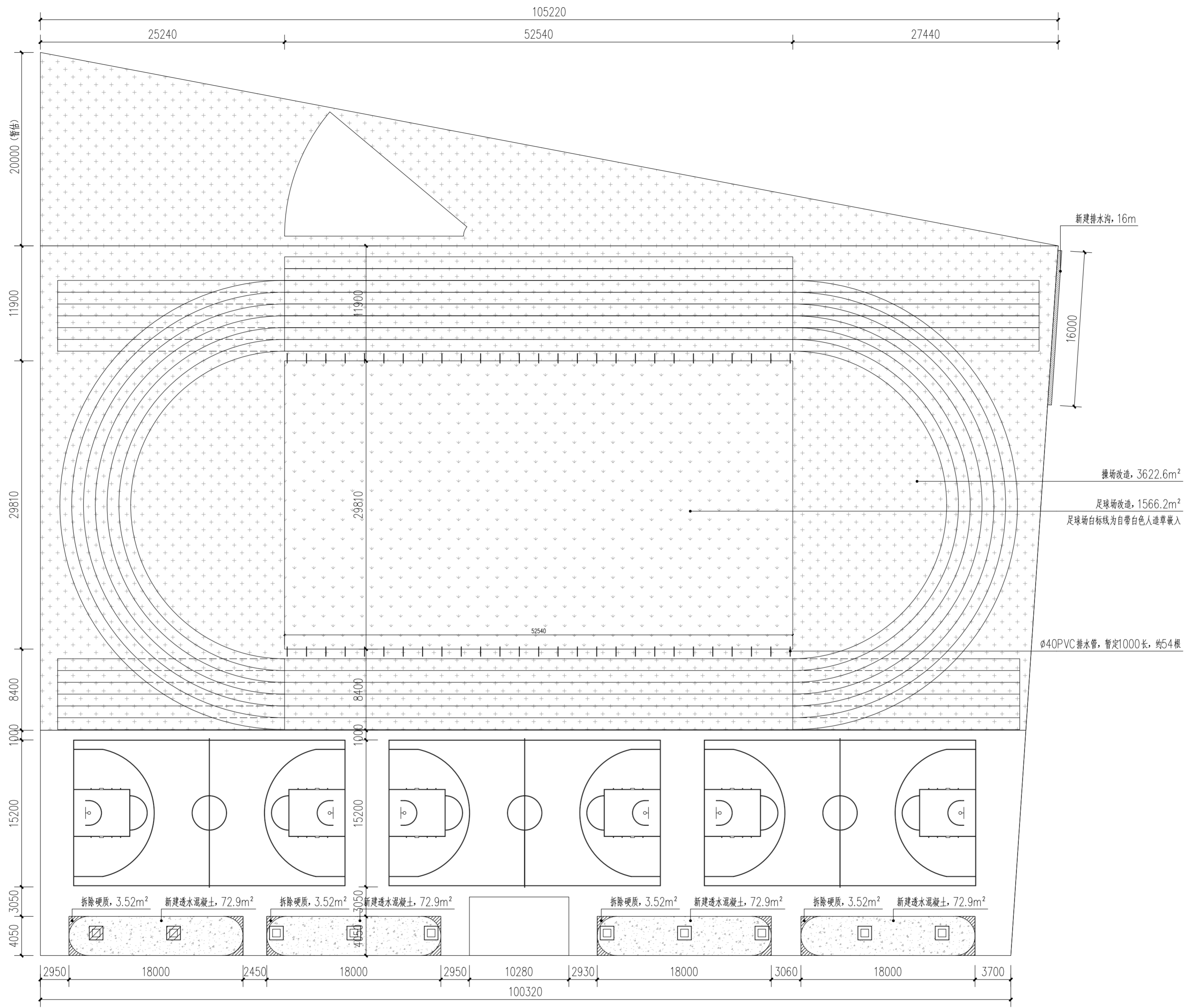
河滨路小学操场平面图 1:300
