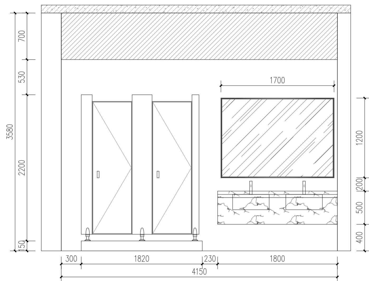
① 公厕立面图A 1:30
