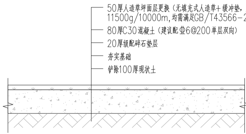
① 足球场改造做法详图 1:10
