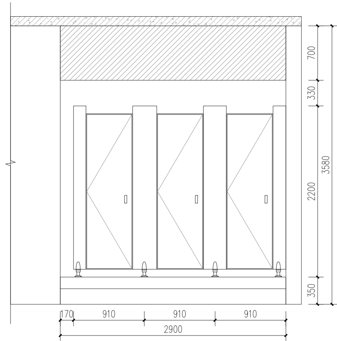
① 公厕立面图E 1:30
