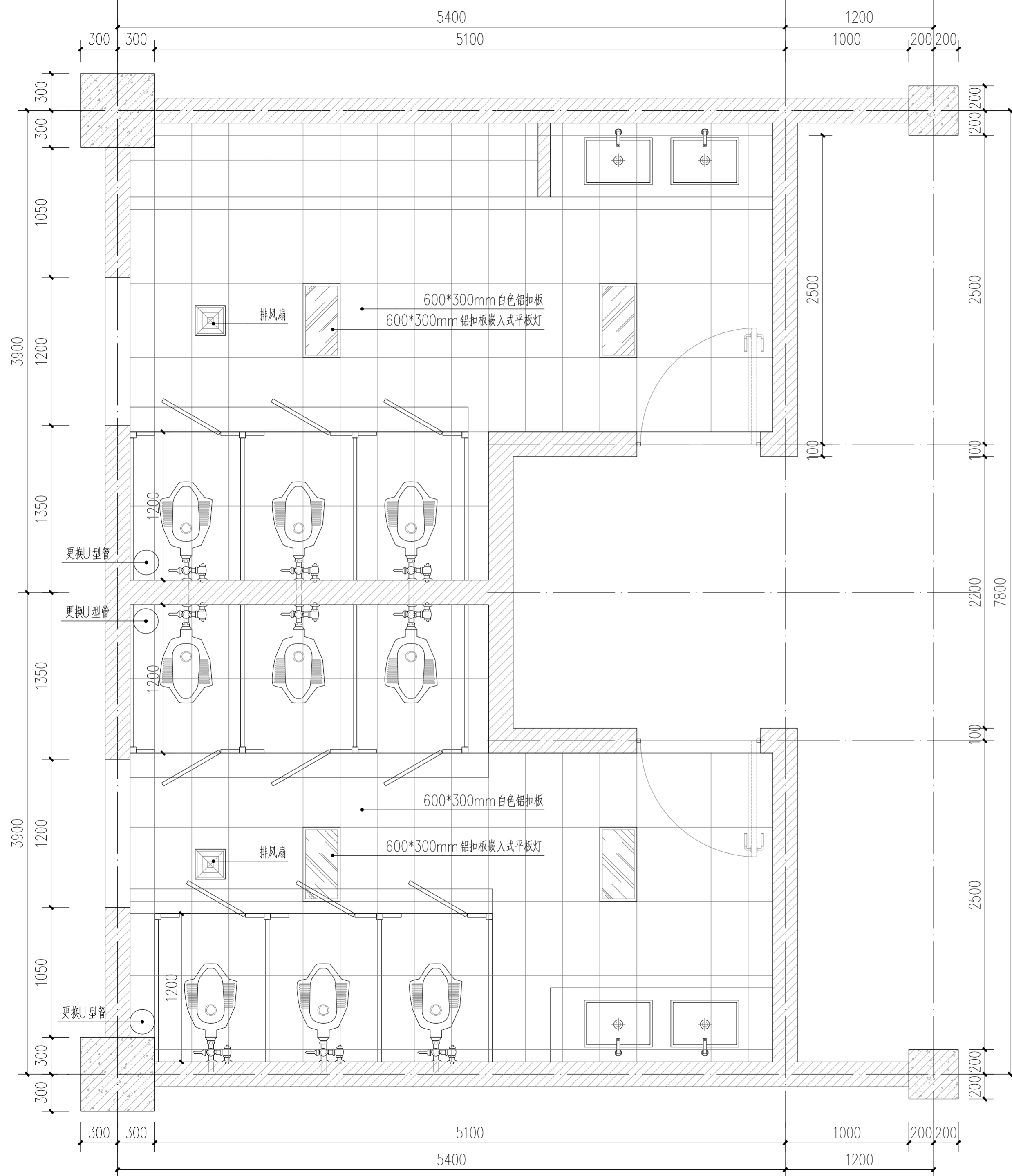
公厕二综合天花板平面图 1:30
