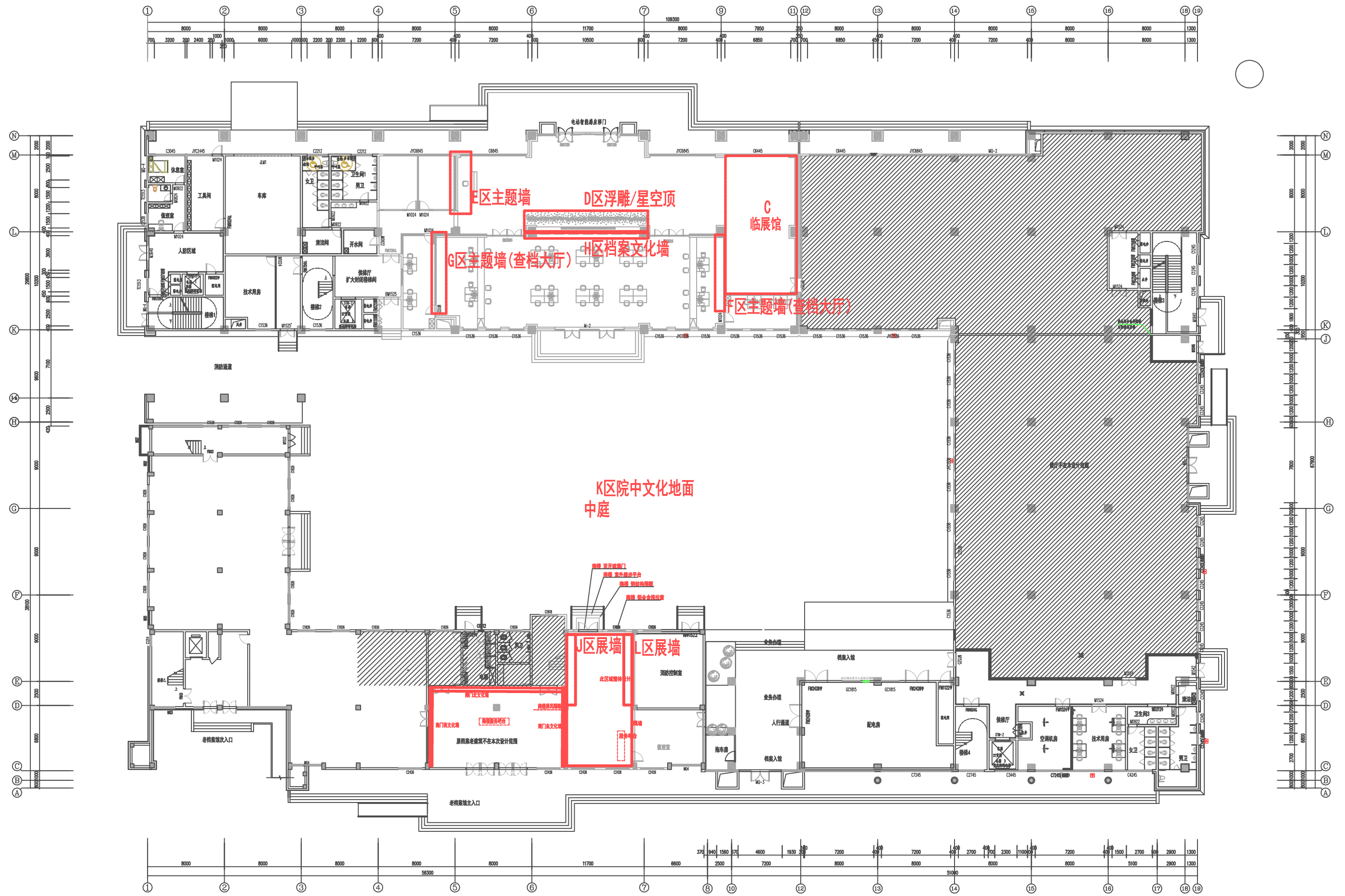
泗洪县档案馆档案库房一层平面图
