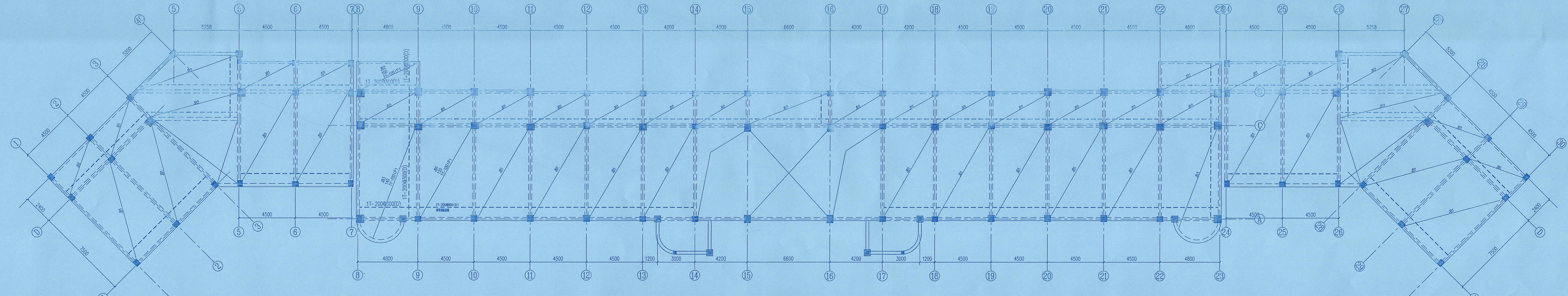
一层加固平面图 说明: 1. JCL1-JCL9系非承重墙体加固详图, 墙体大样见标准-04;
