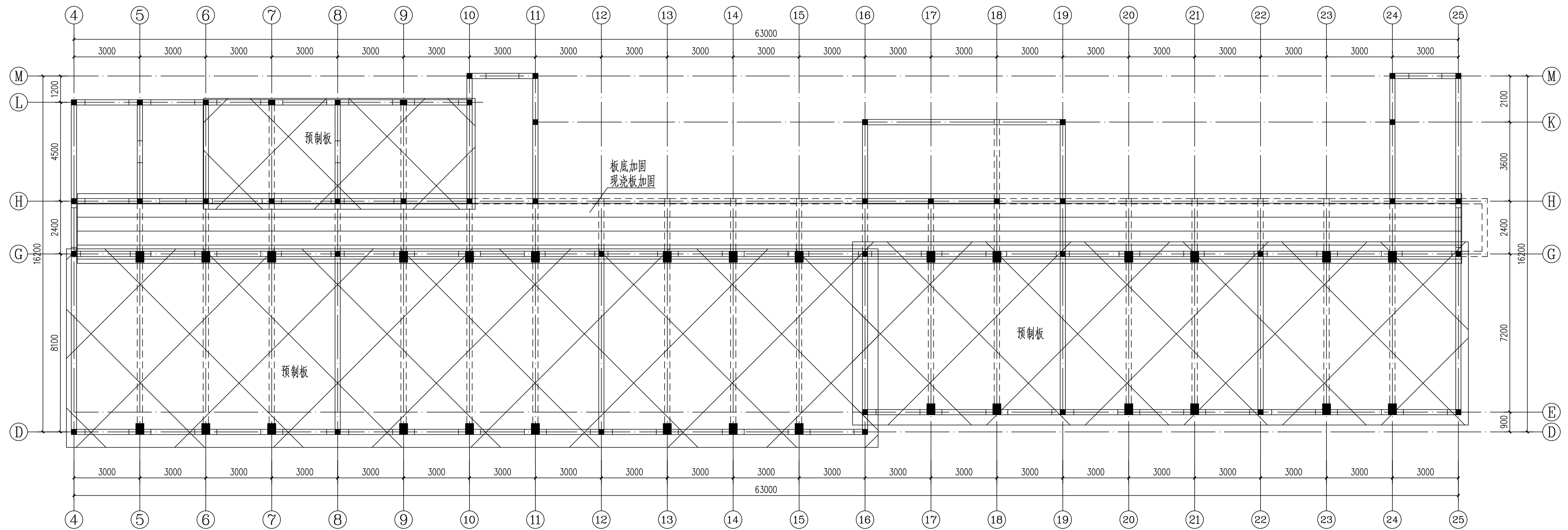
二、三、四层顶板加固布置图 1:100 7.150M 10.750M 14.350M
