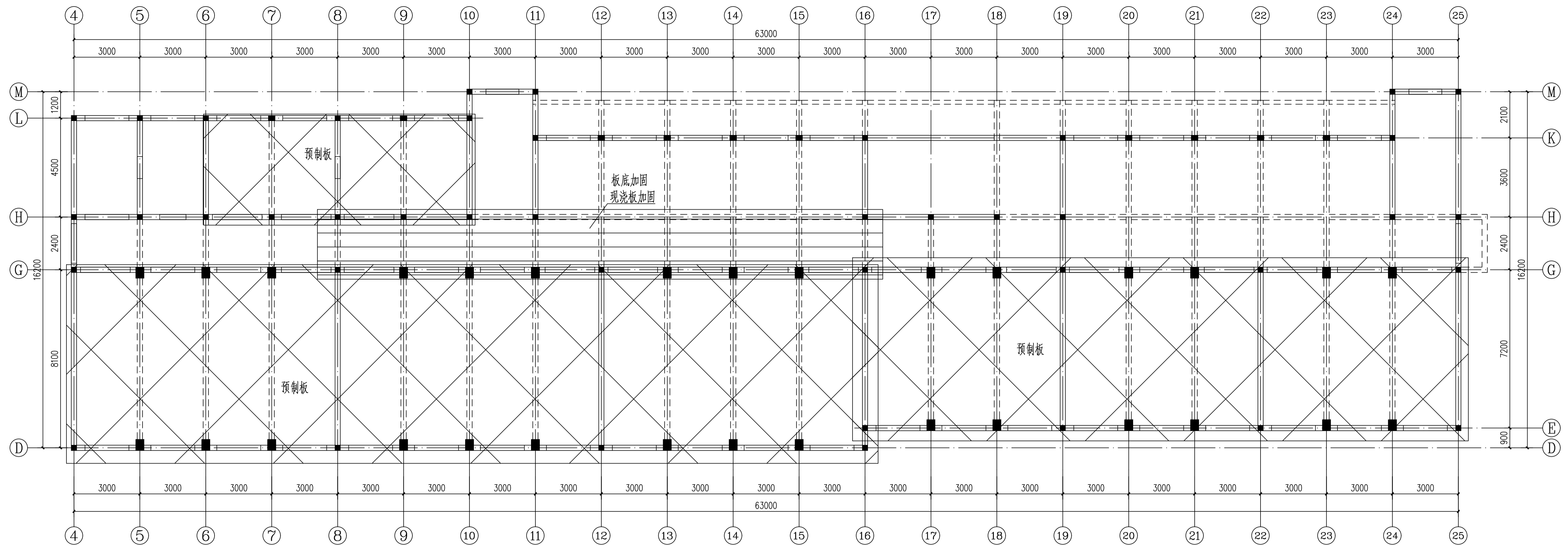
一层顶板加固布置图 1:100 3.550M
