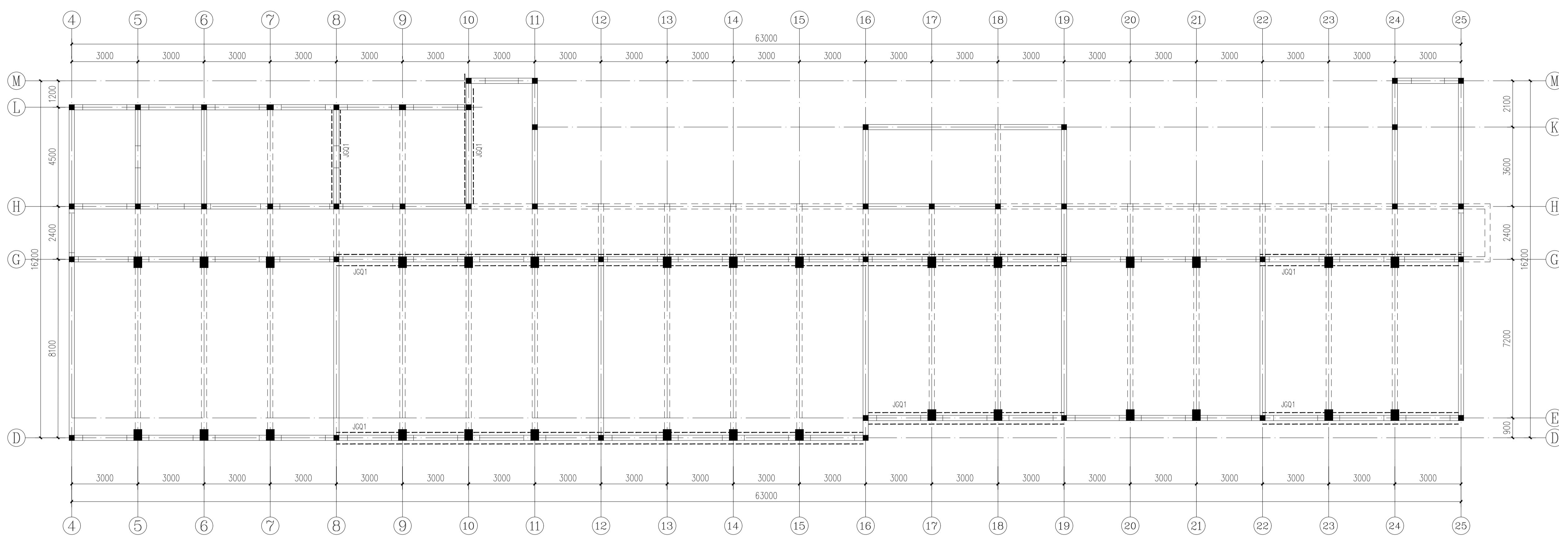
三层墙体加固布置图 1:100
