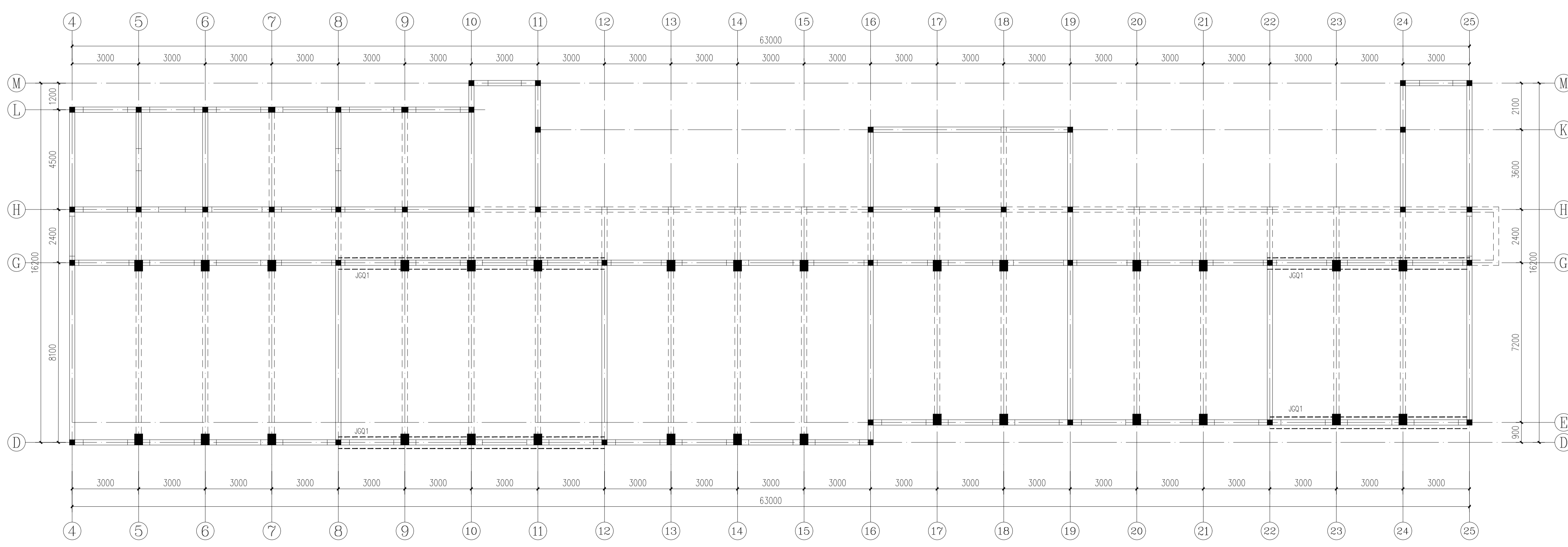
四层墙体加固布置图 1:100
