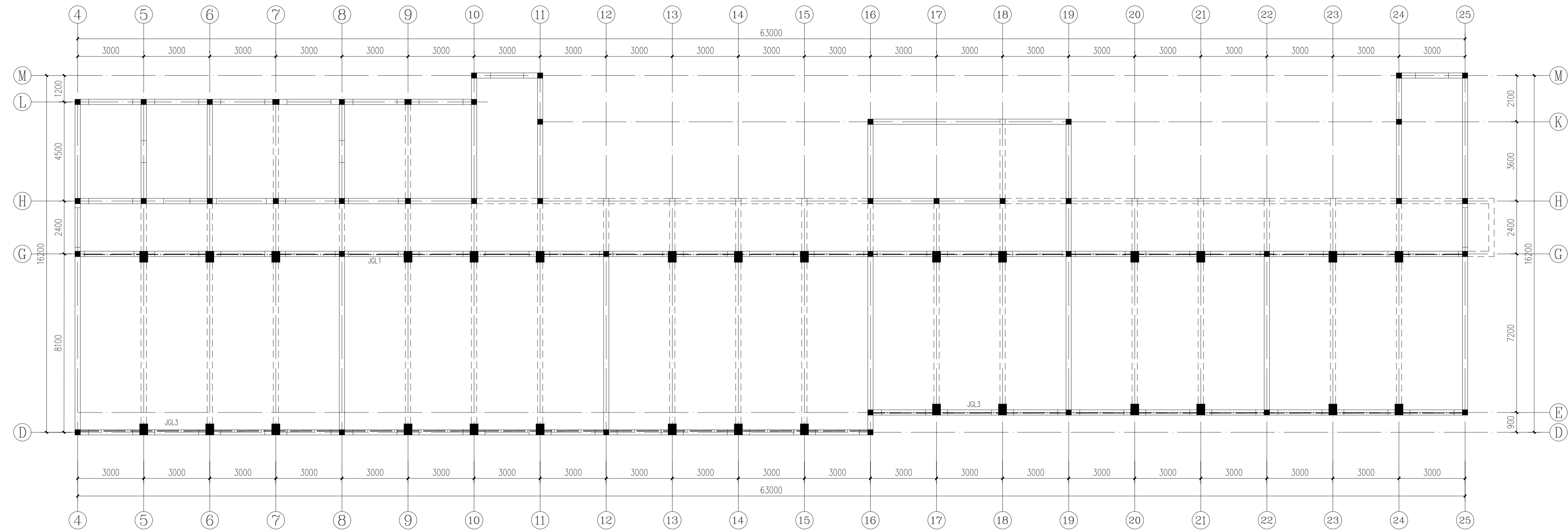
二、三、四层顶梁加固布置图 1:100 7.150M 10.750M 14.350M
