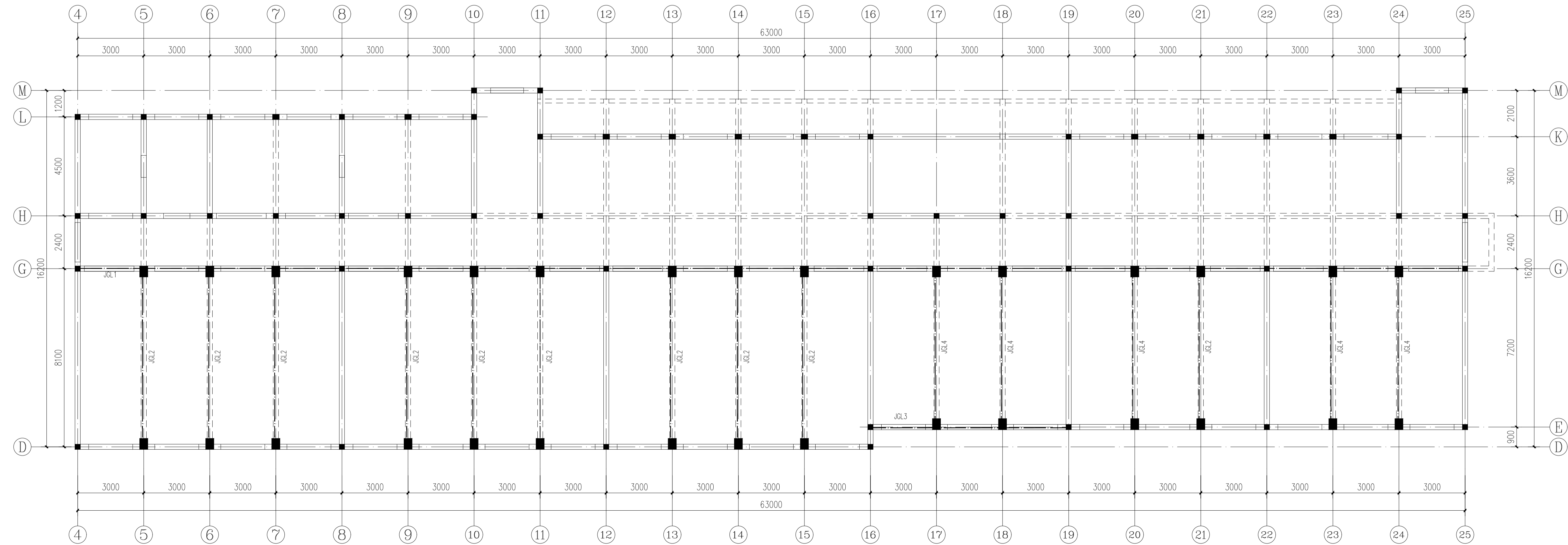
五层顶梁加固布置图 1:100 17.950M
