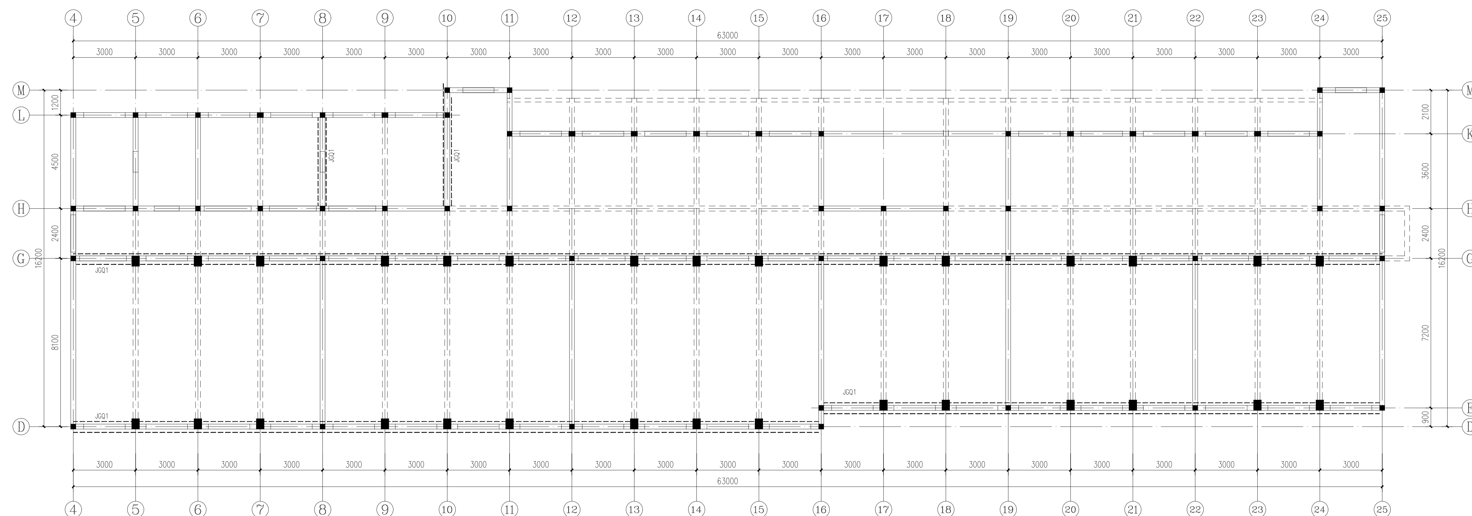
一层墙体加固布置图 1:100
