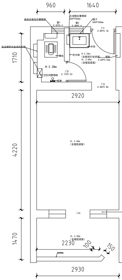
平面图
