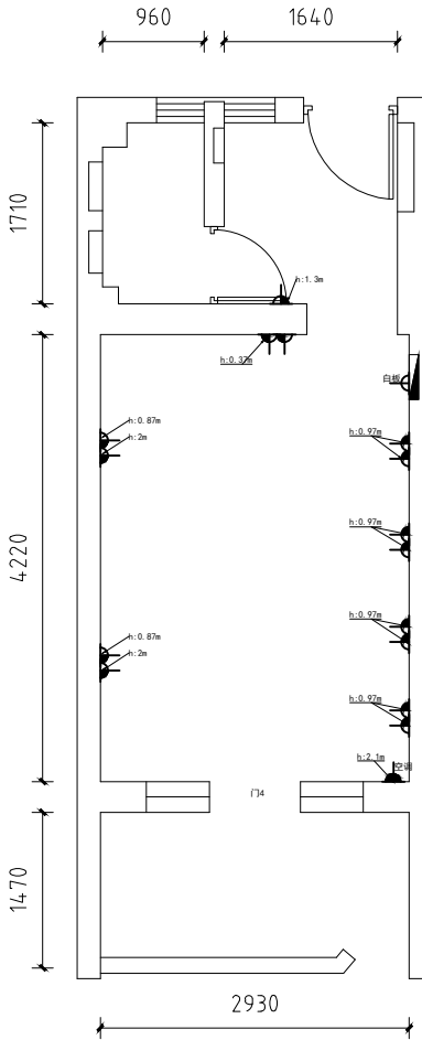
插座位置
