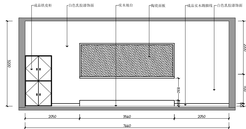
02 1F 普通教室02立面图
