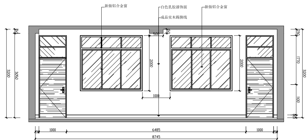
03 1F 普通教室03立面图
