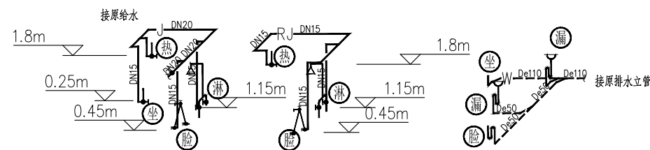
宿舍三层教师宿舍给排水布置图
