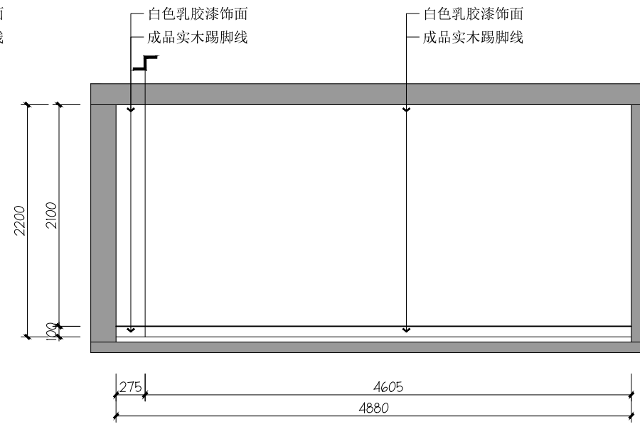
06 体育馆二层办公室06立面图
