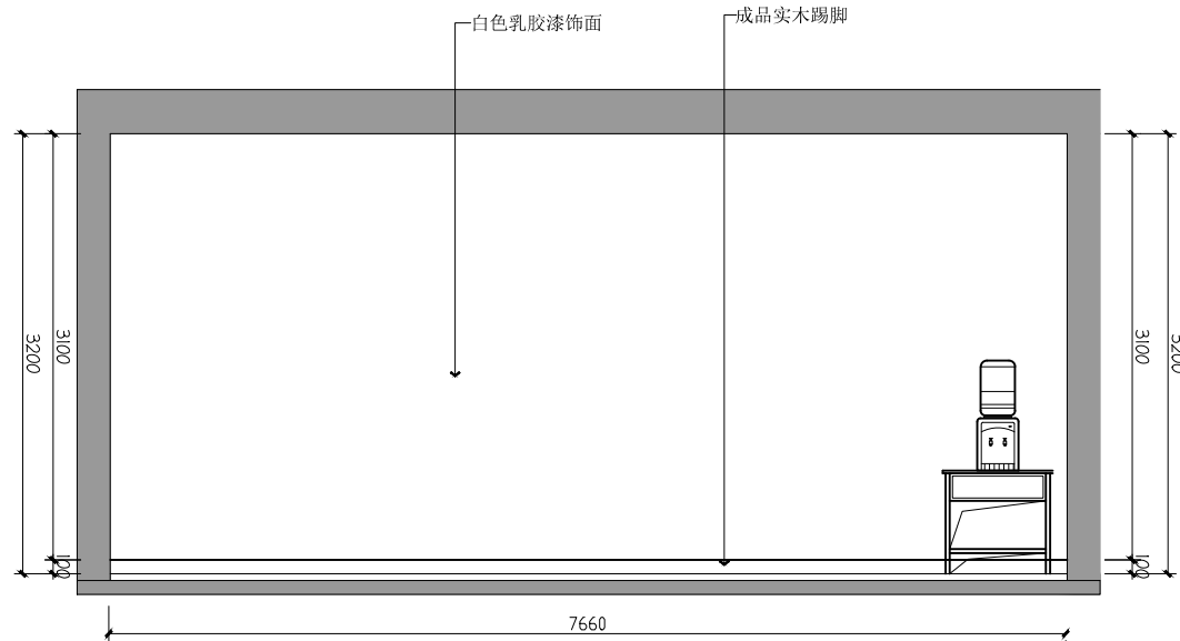
08 办公室08立面图 1F Scale 1:60
