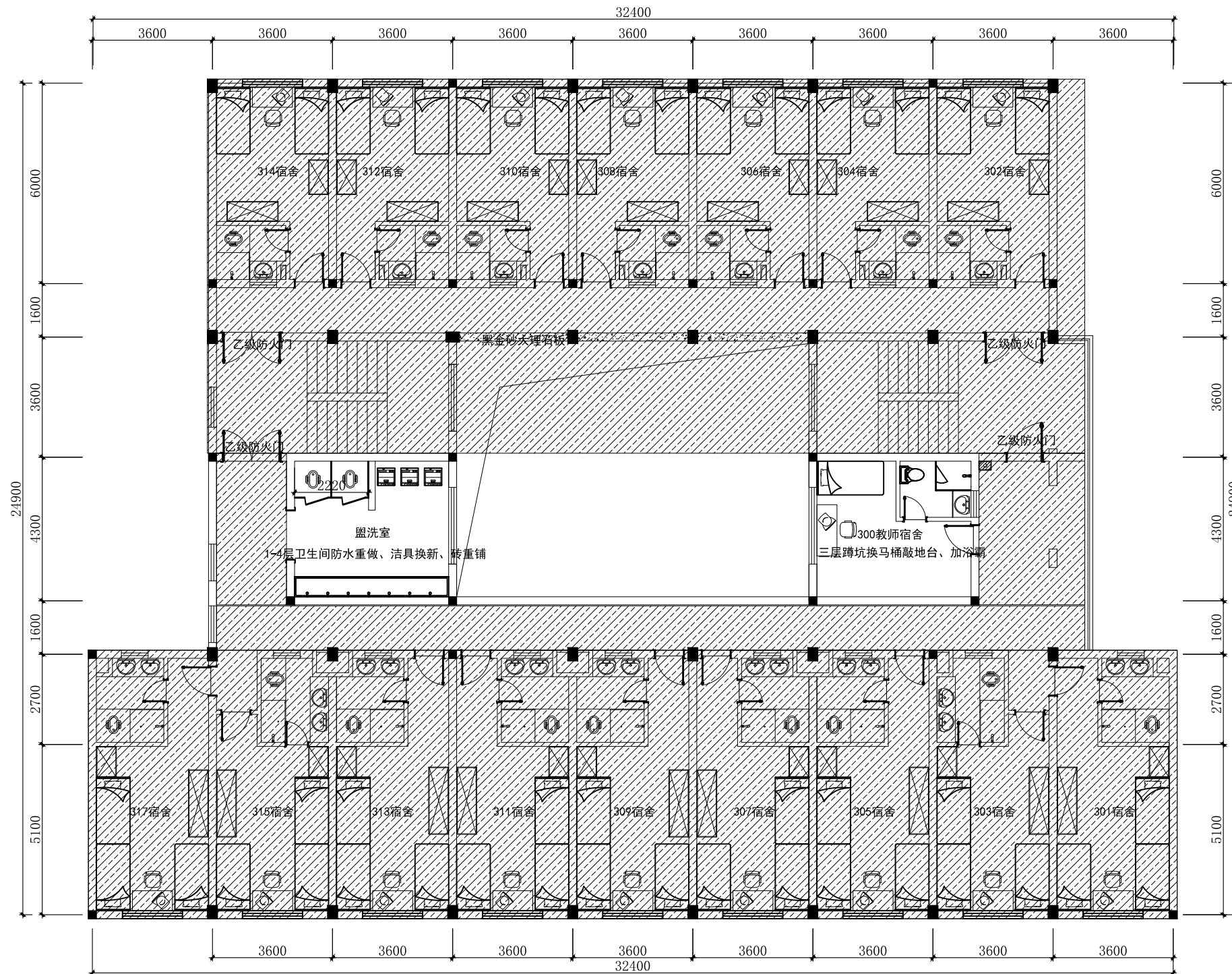
宿舍三层平面布置图
