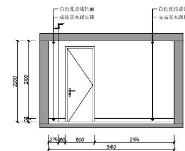
02 体育馆二层02立面图
