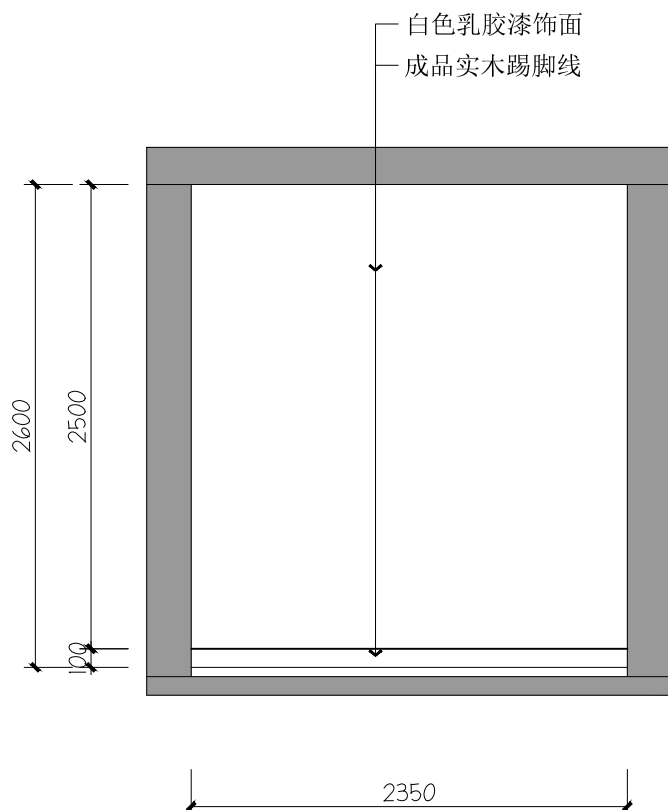
21 体育馆一层21立面图
