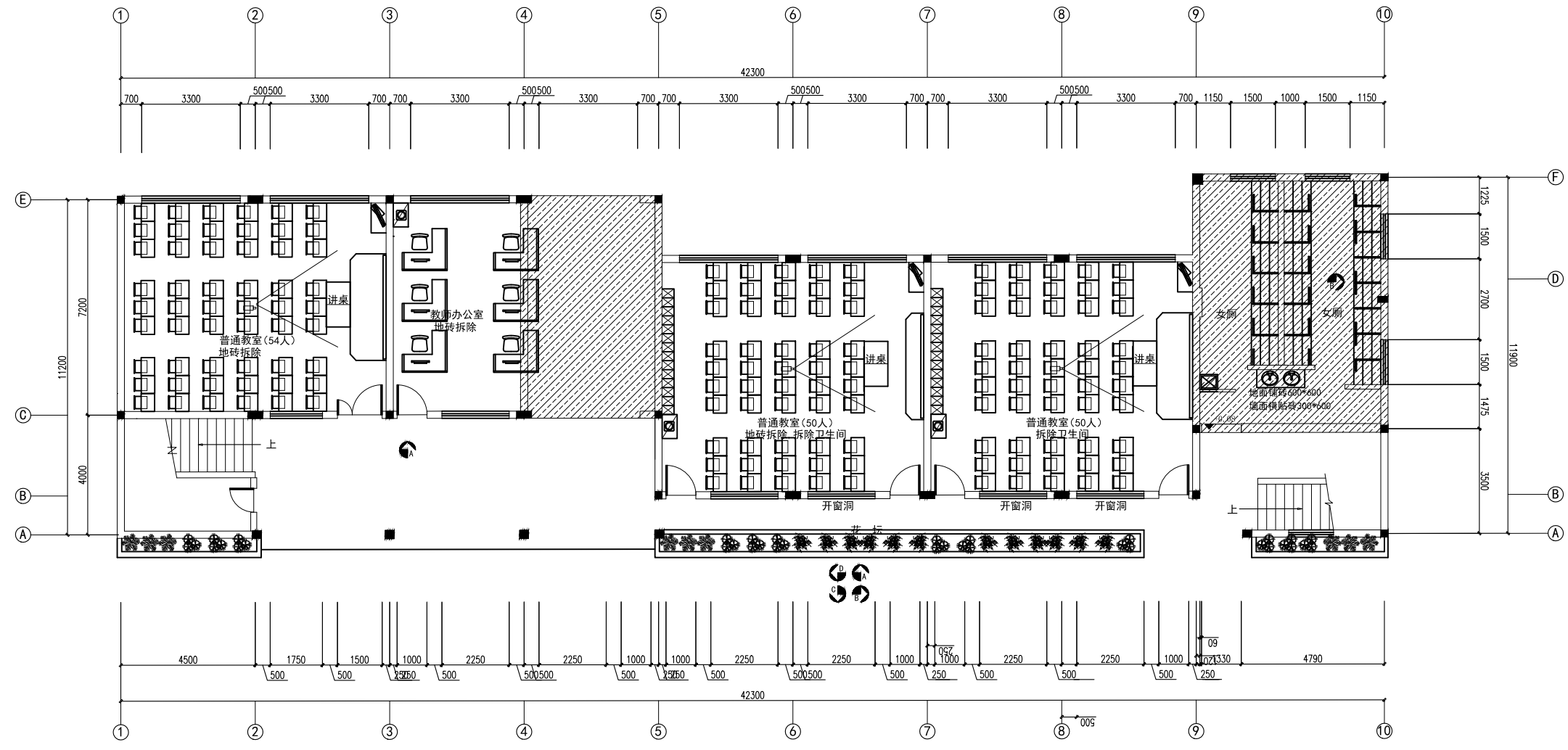
志学楼一层平面布置图
