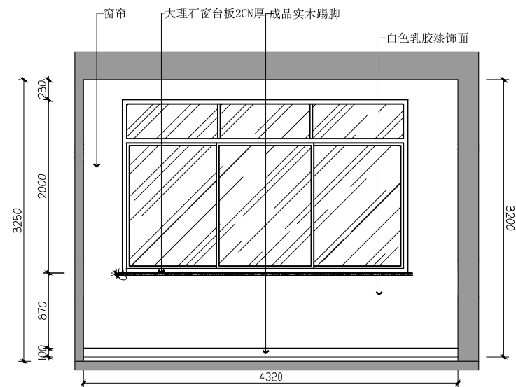
05 办公室05立面图 1F Scale 1:60
