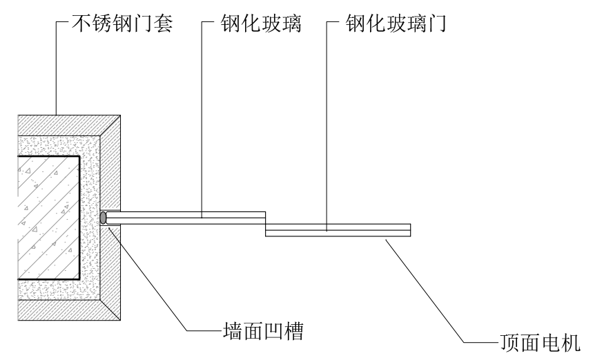
自动感应门节点图
