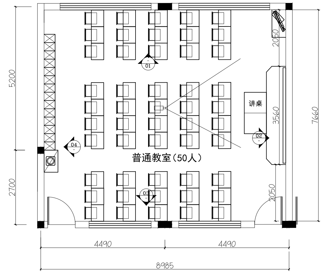
普通教室索引图
