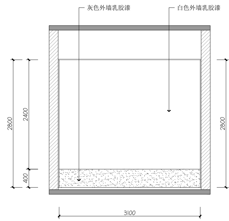
04 1F 仓库04立面图
