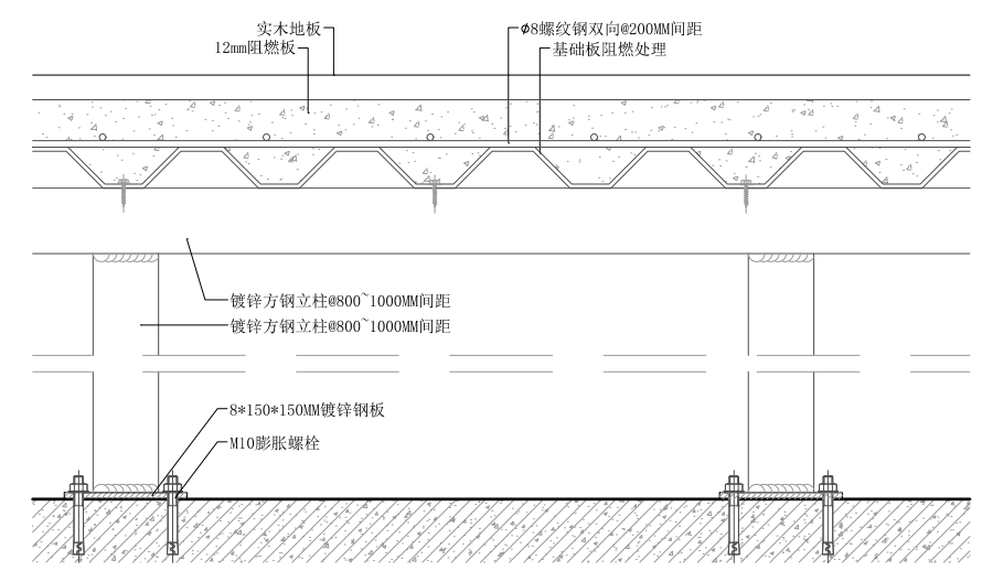
实木地台节点图
