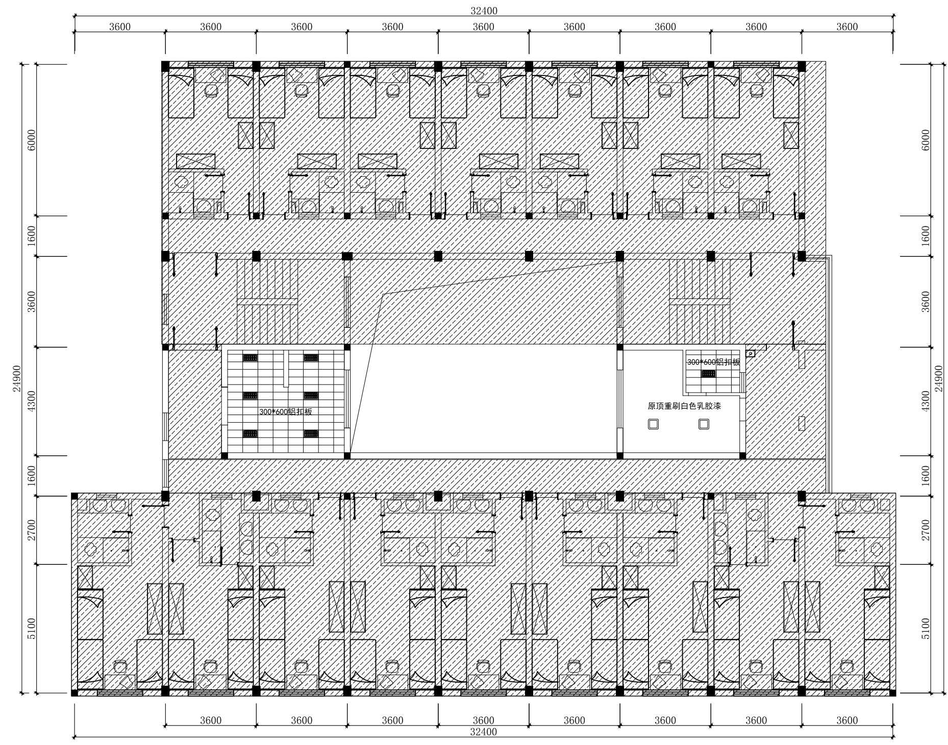
宿舍三层顶面布置图
