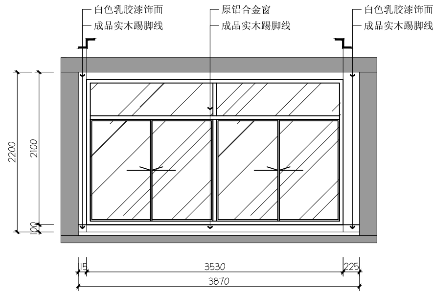
05 体育馆二层办公室05立面图
