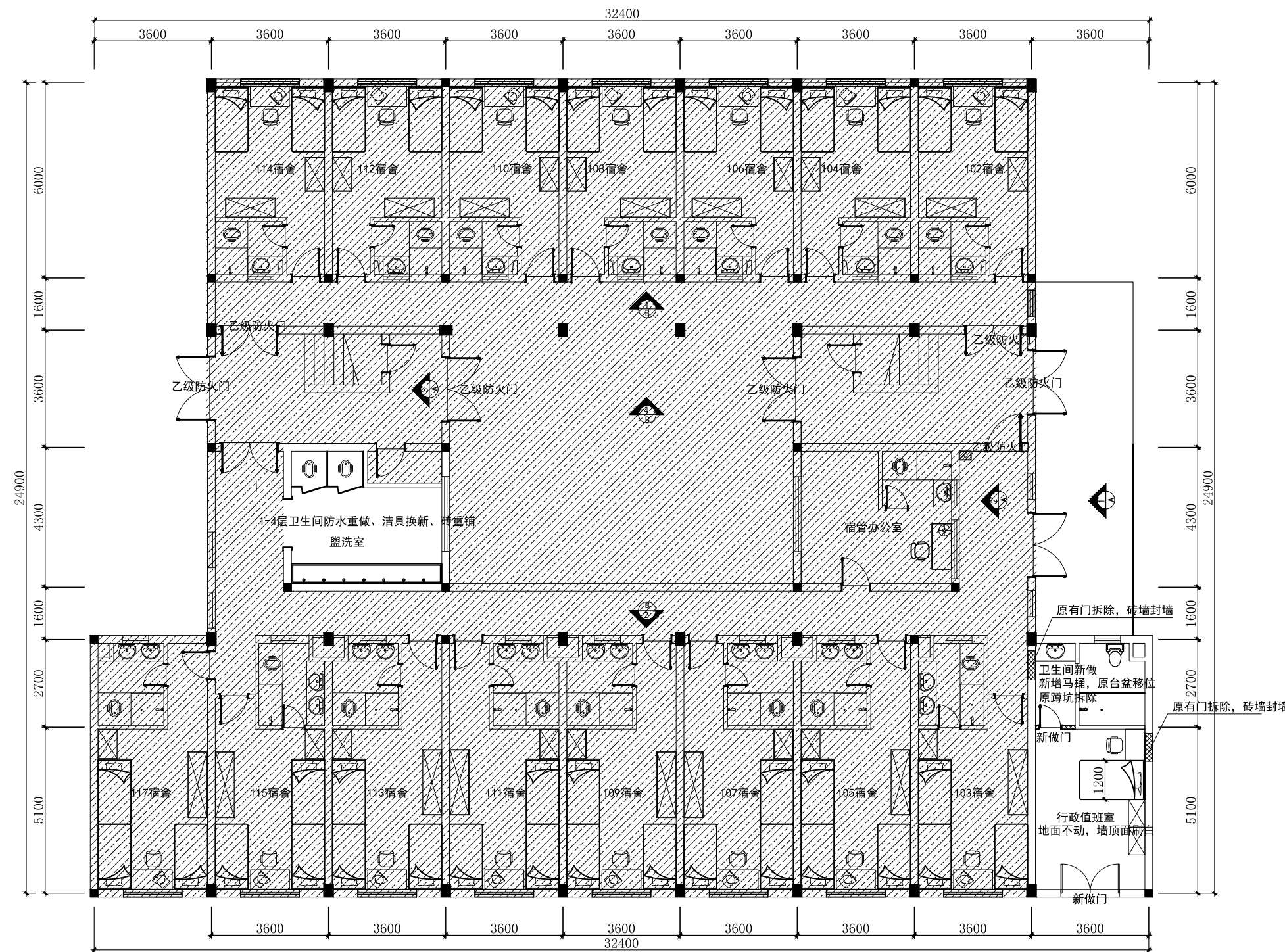
宿舍一层至四层平面布置图
