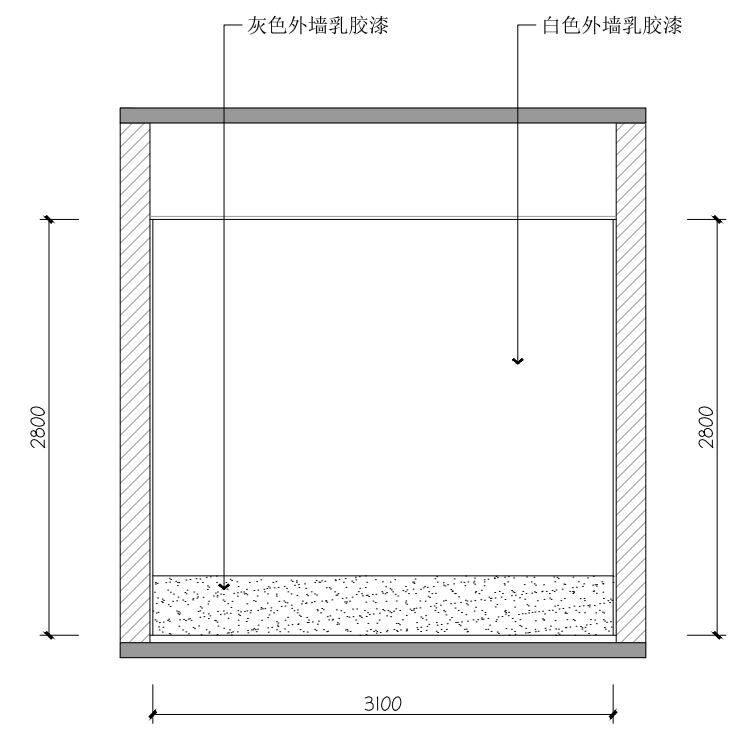
02 1F 仓库02立面图
