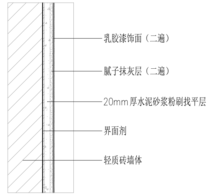
墙面乳胶漆节点图
