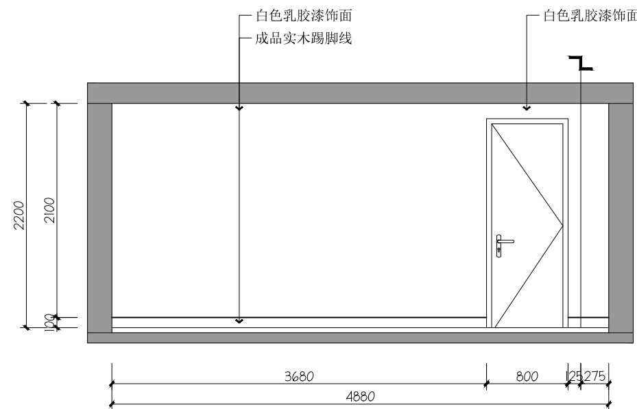
08 体育馆二层办公室08立面图
