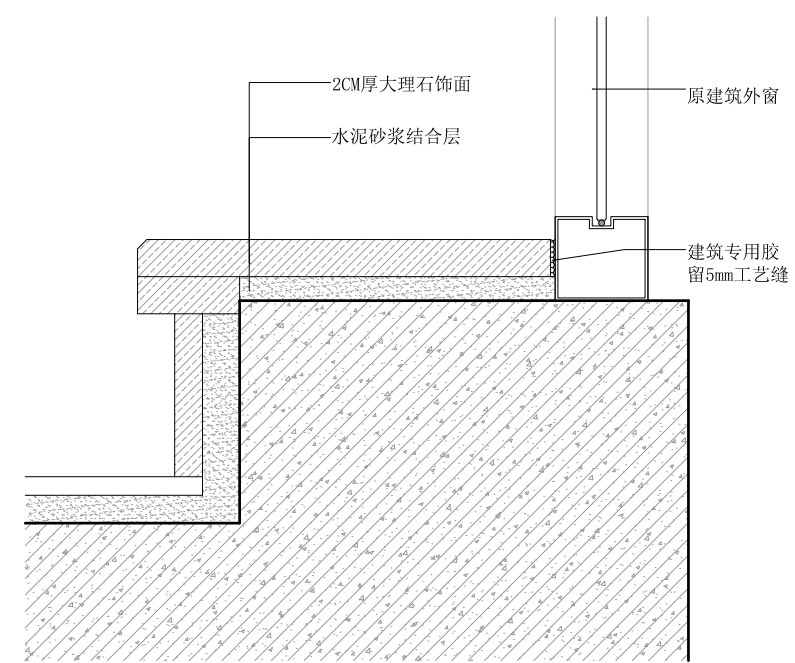
窗台大理石节点图
