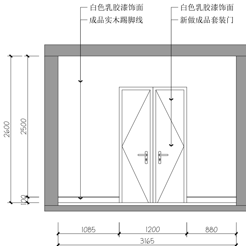
22 体育馆一层22立面图
