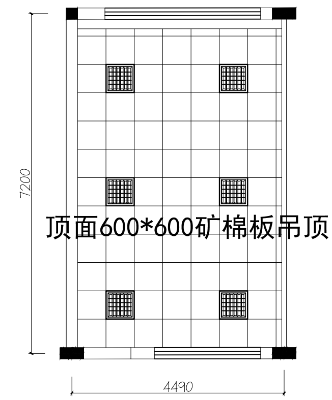
办公室顶面图
