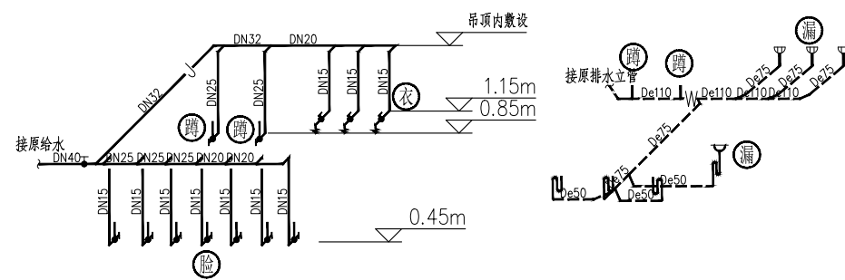
宿舍一~四层公共卫生间给排水布置图 共四间
