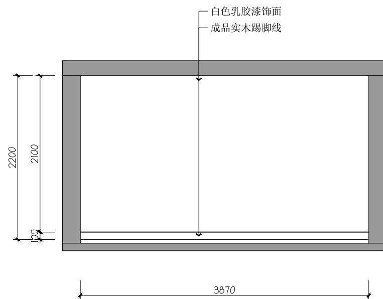
07 体育馆二层办公室07立面图
