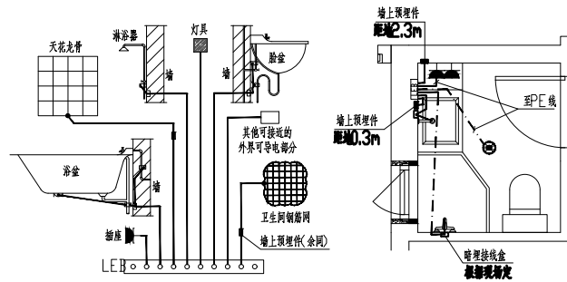
有淋浴设施的卫生间局部等电位连接原理图 有淋浴设施的卫生间局部等电位连接平面图
