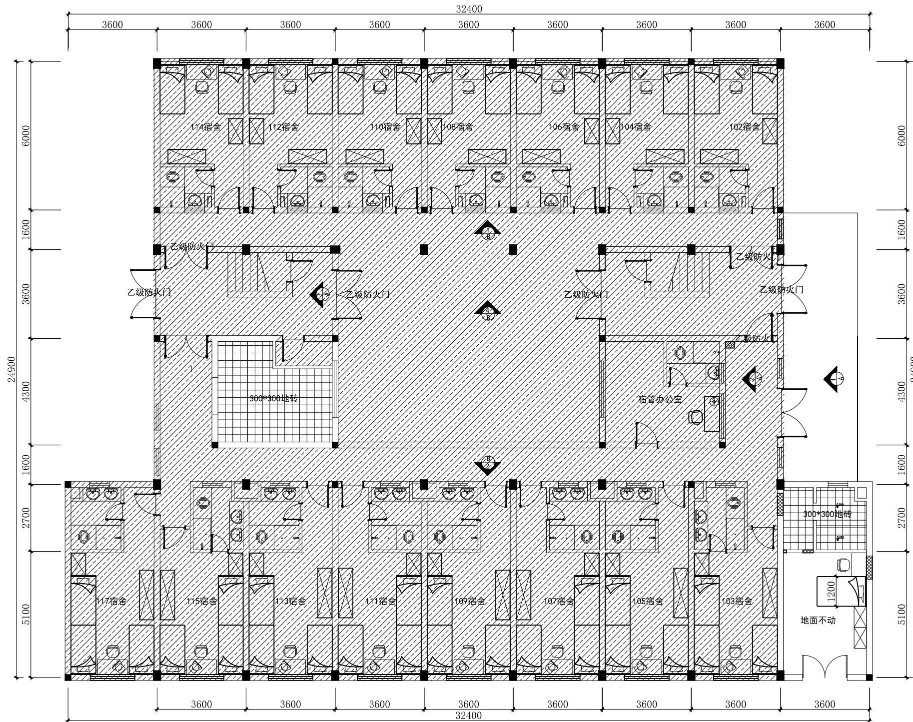
宿舍一层至四层地面材质图
