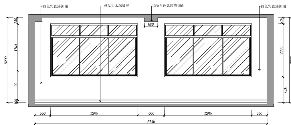
01 1F 普通教室01立面图
