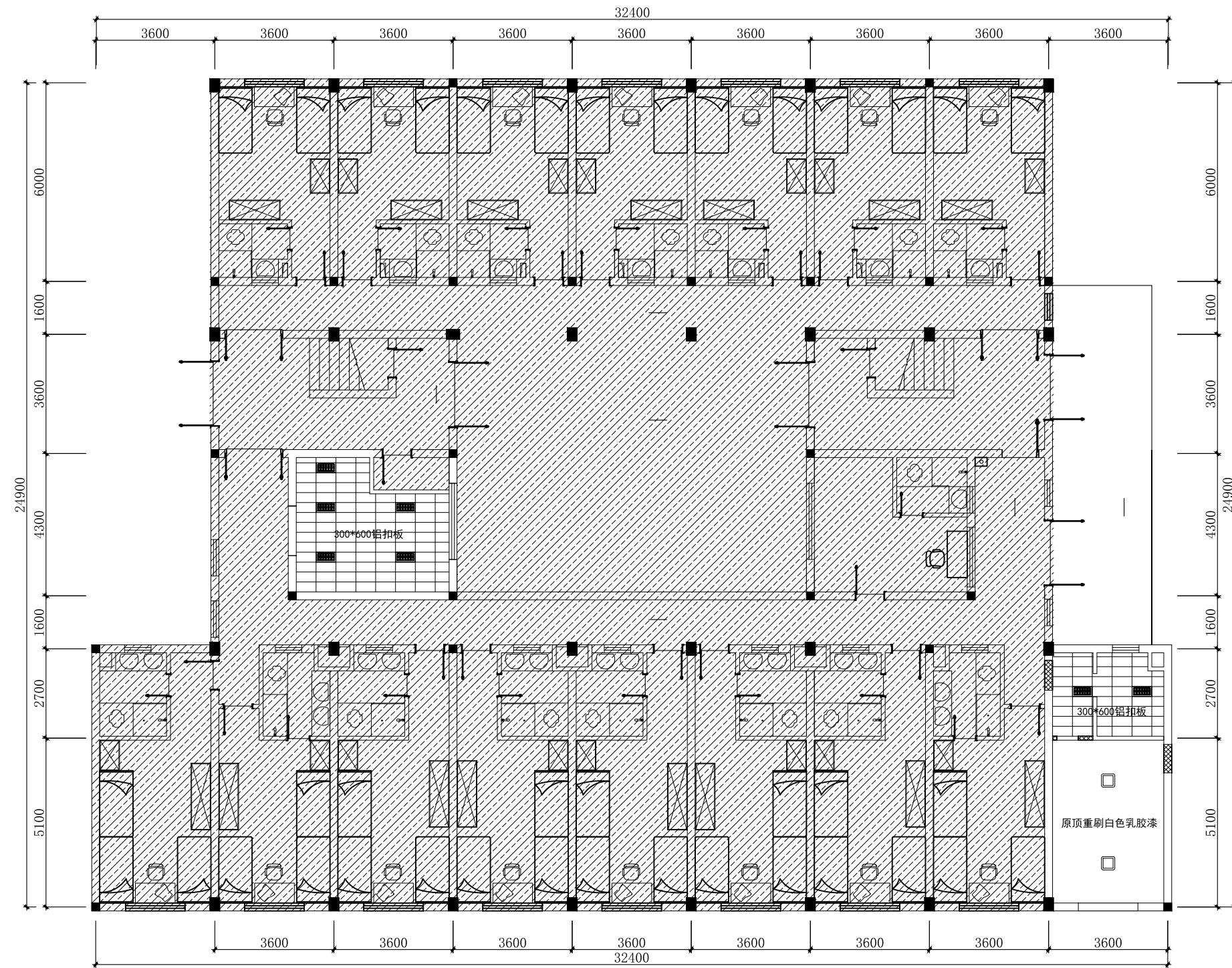
宿舍一层至四层顶面布置图
