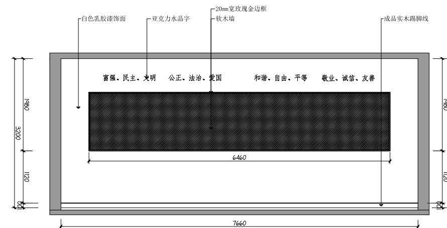
04 1F 普通教室04立面图
