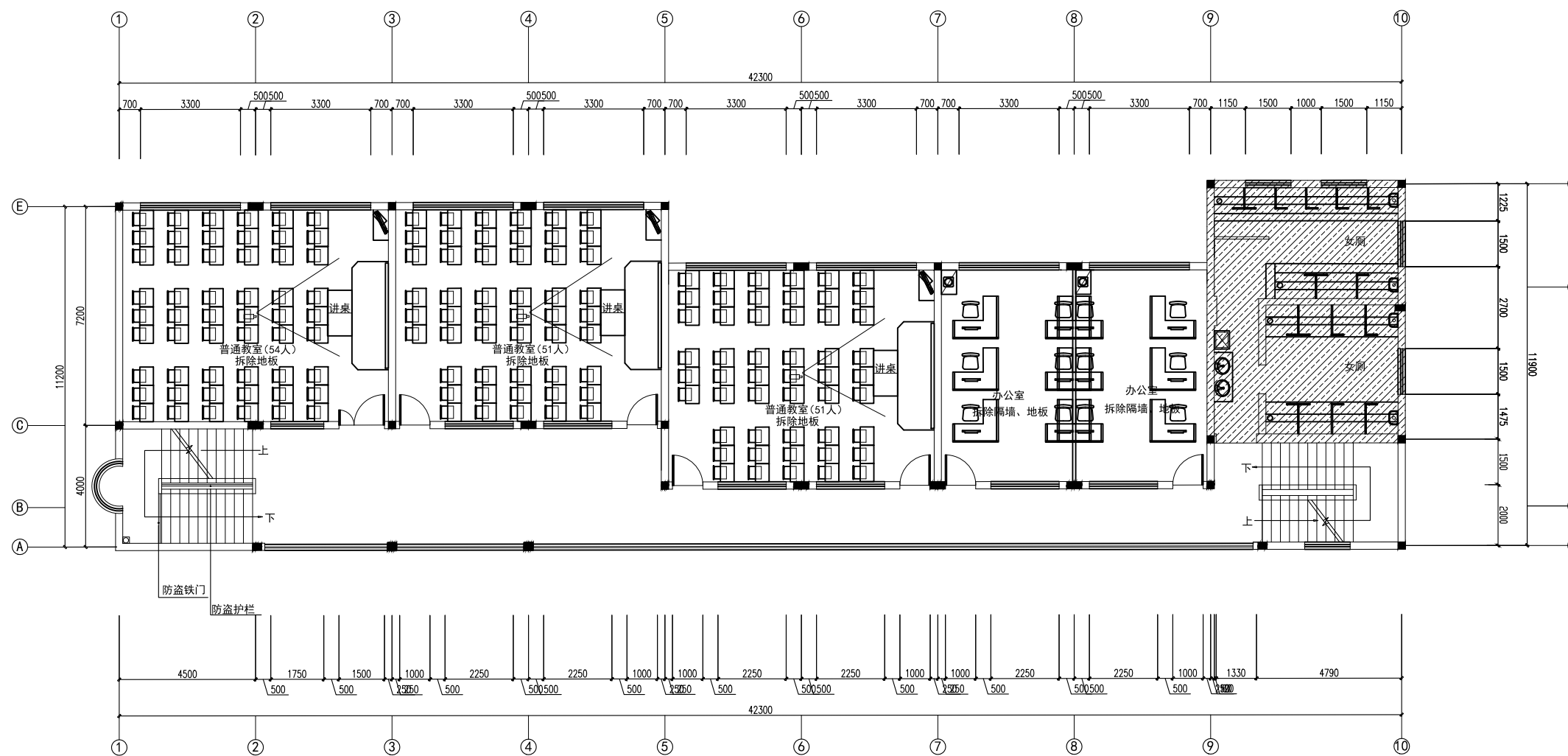
志学楼二层平面布置图
