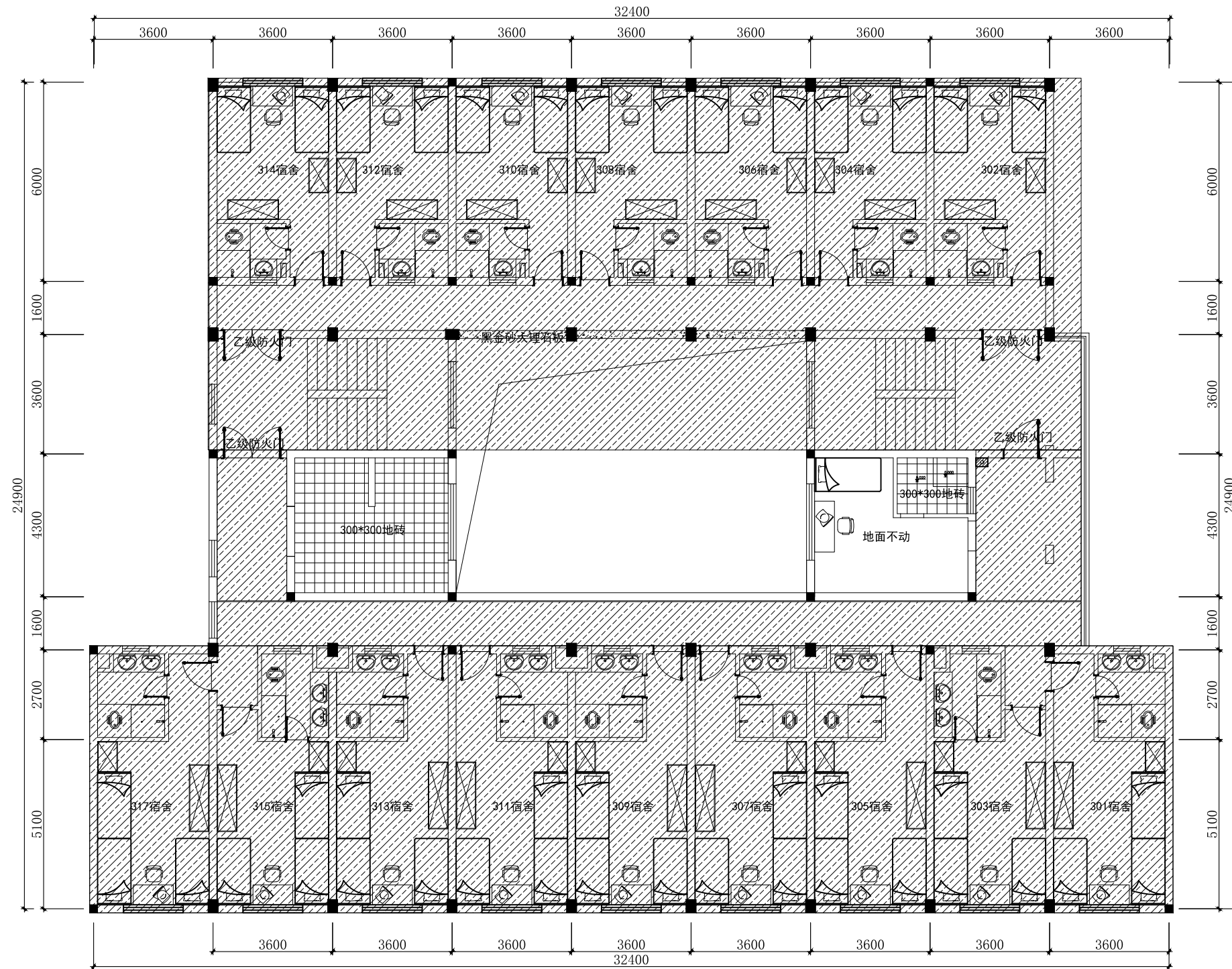
宿舍三层地面材质图
