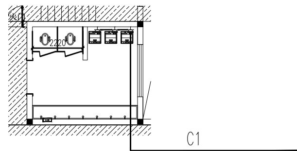
宿舍一~四层卫生间插座布置图
