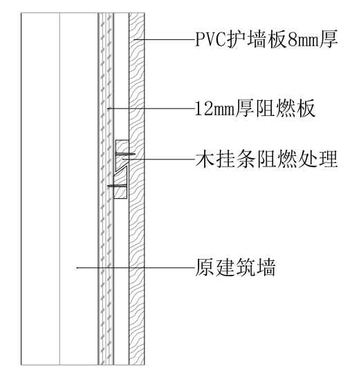
护墙板节点图
