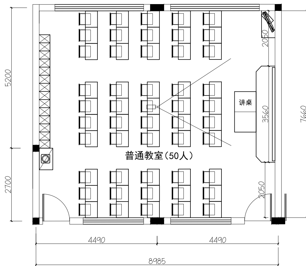
普通教室平面图
