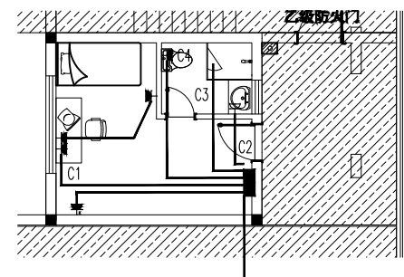
宿舍三层教师宿舍插座布置图
