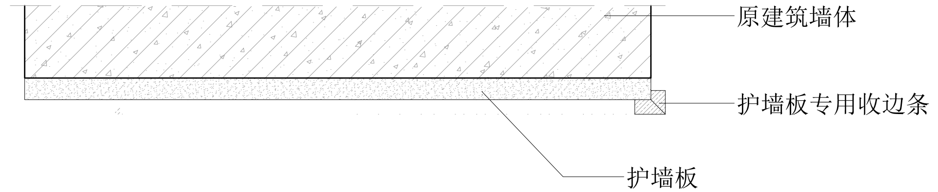
护墙板收口条节点图
