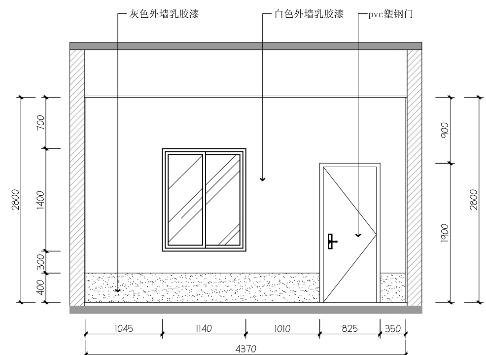
01 1F 仓库01立面图
