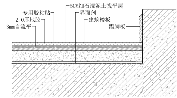
地胶节点图
