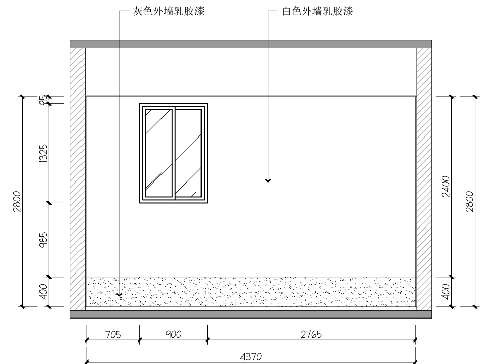
03 1F 仓库03立面图
