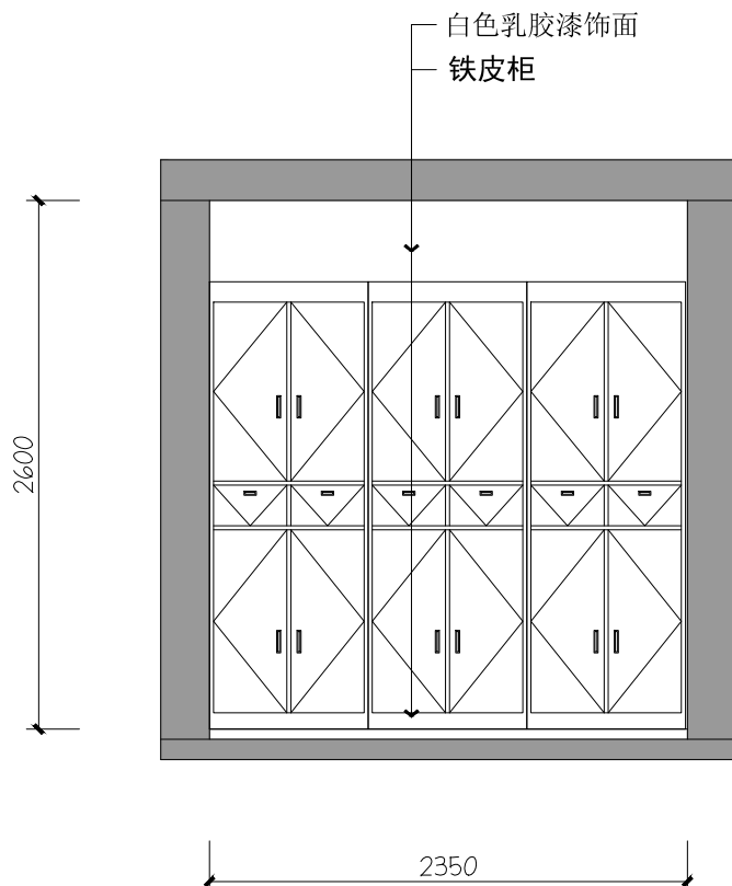
23 体育馆一层23立面图
