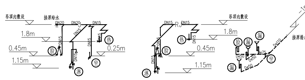
一层值班室给排水布置图
