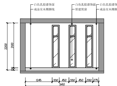
04 体育馆二层04立面图
