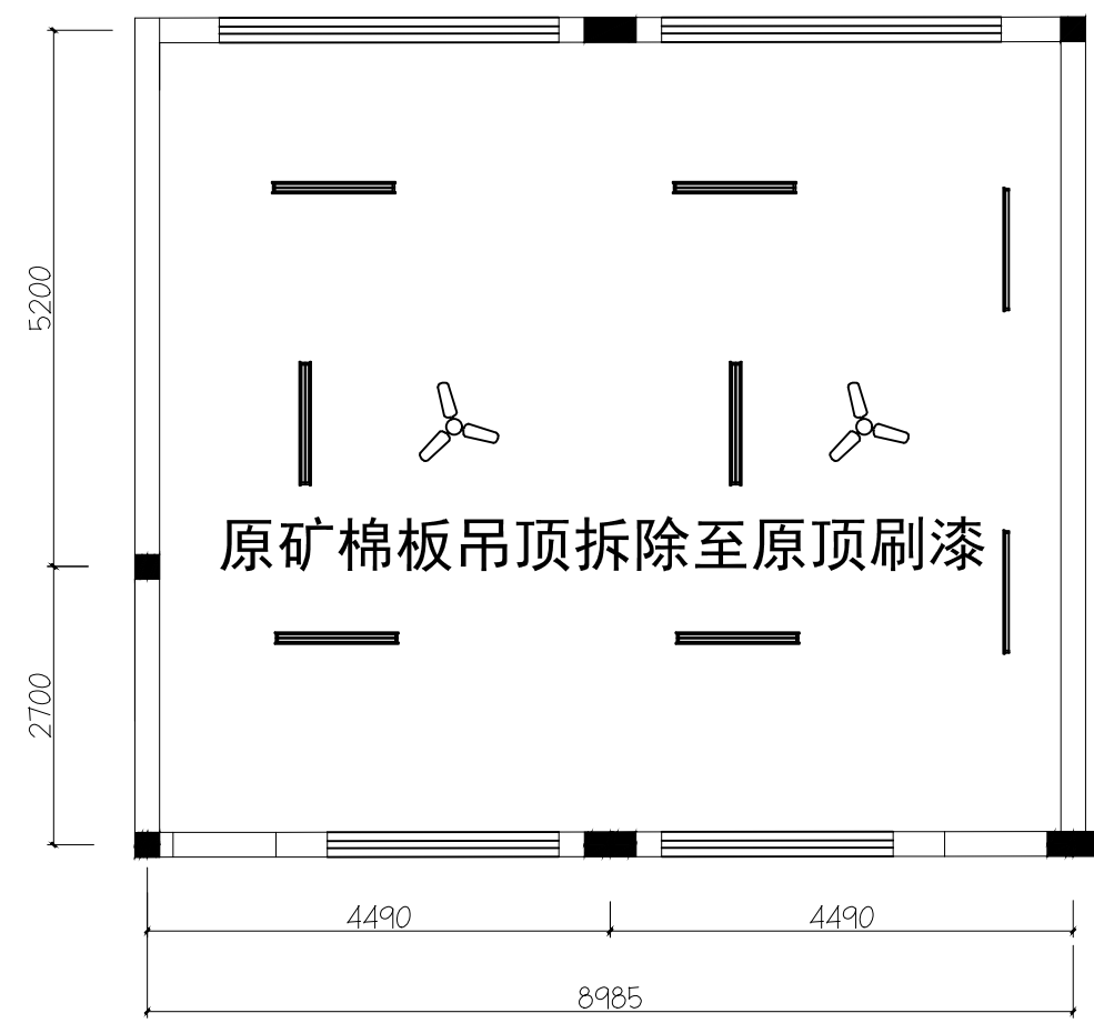
普通教室顶面图
