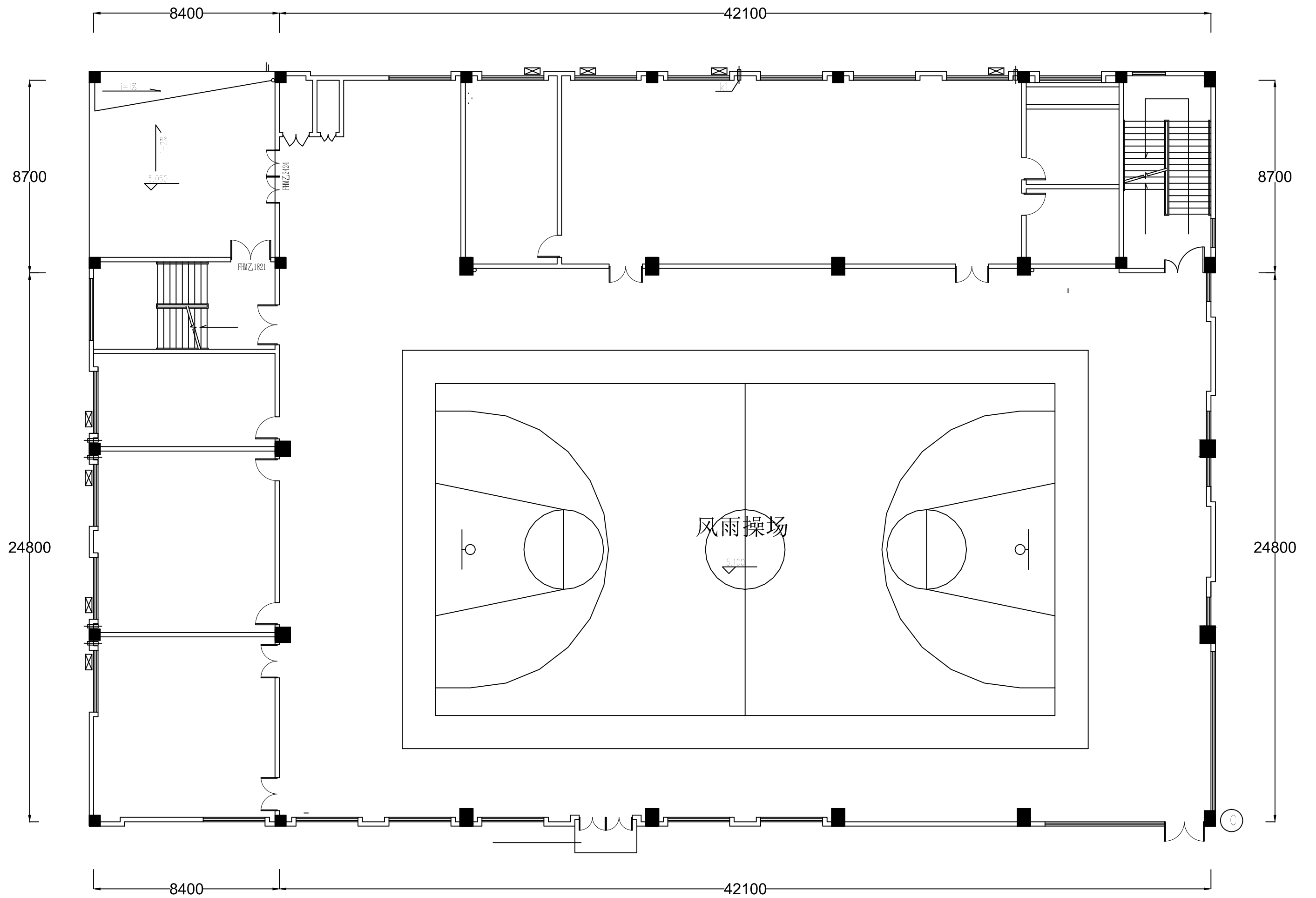
风雨操场平面图纸
