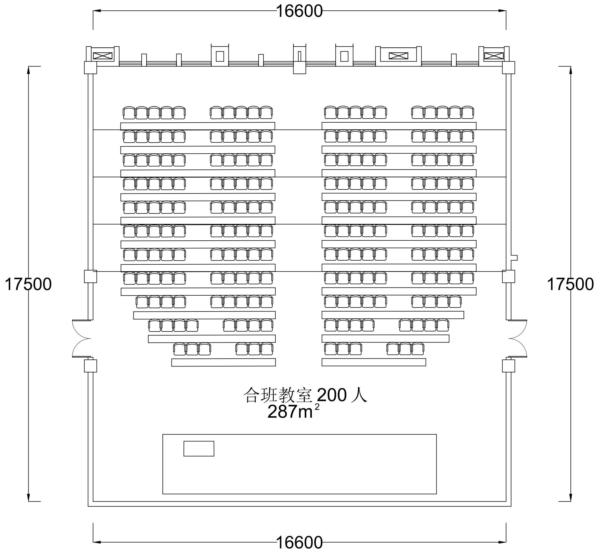
合班教室平面图纸
