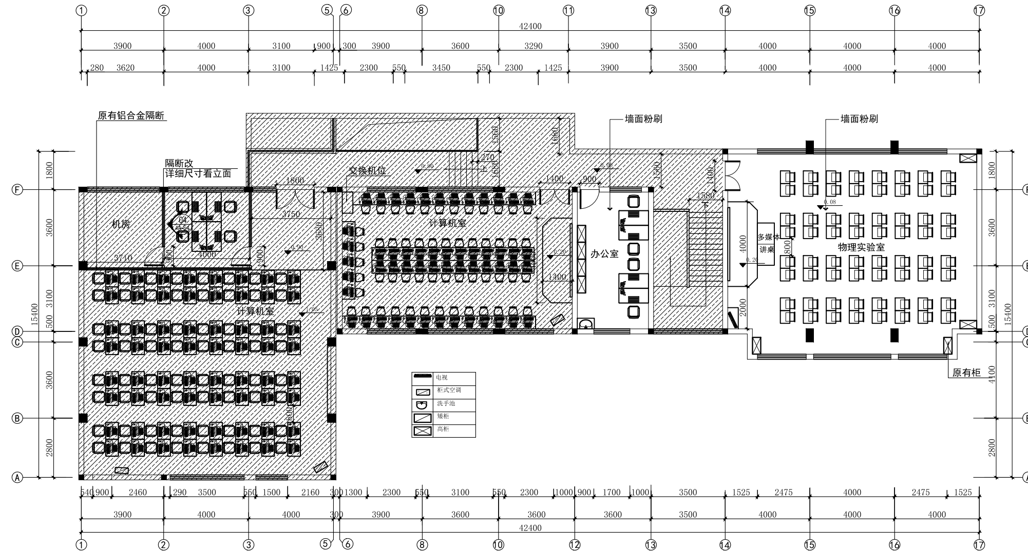
4F PLAN 实验楼 SCALE: 1:150
