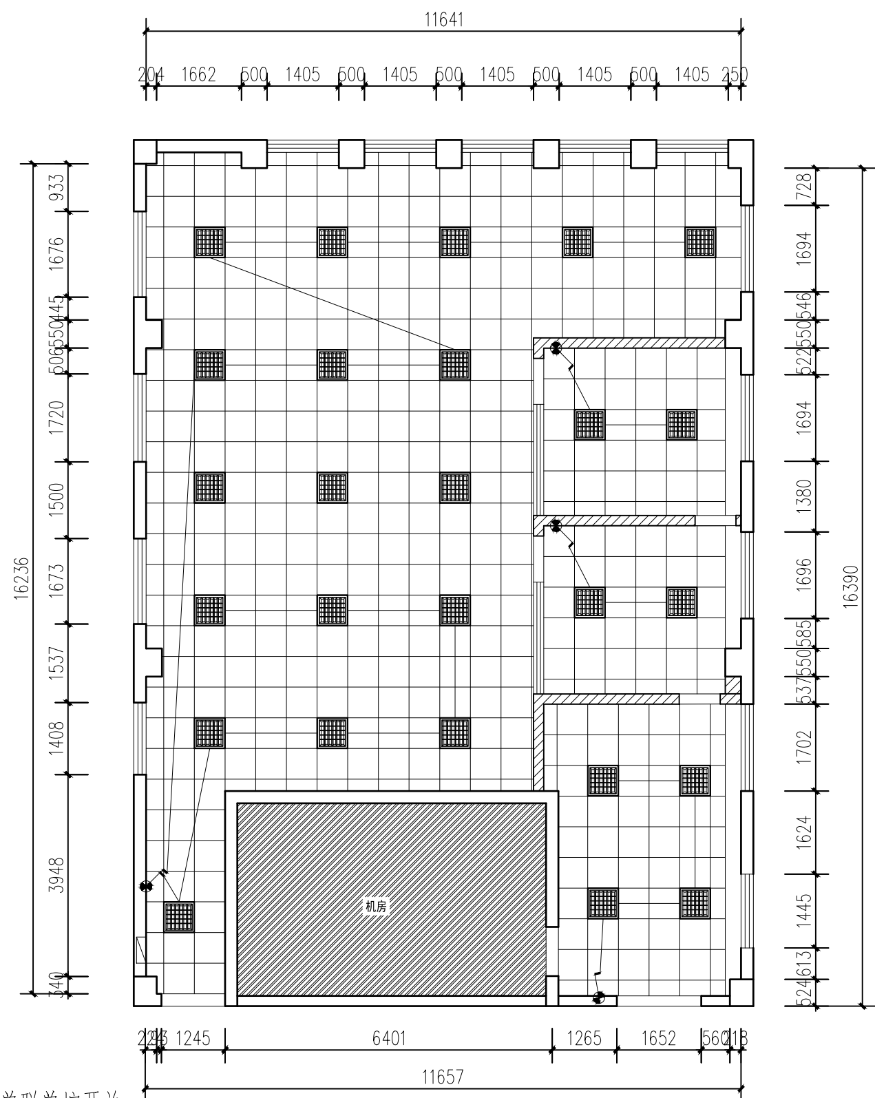
图书馆多媒体教室照明线路图
