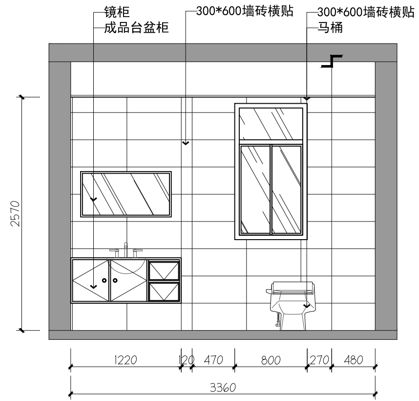
05 行政值班室05立面图 1F
