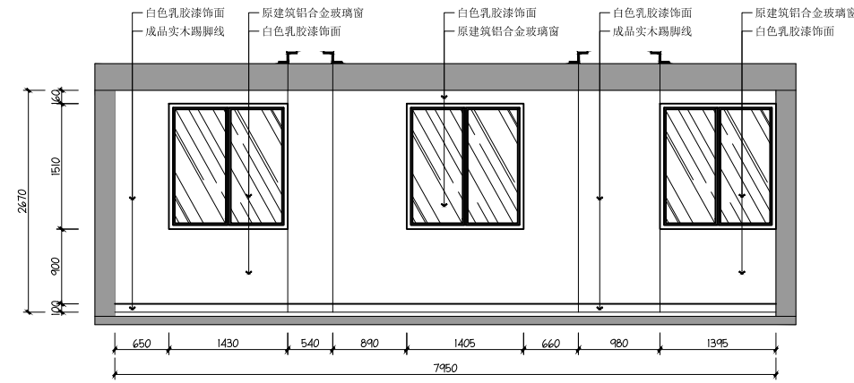
01 宣泄室01立面图 Scale 1:50
