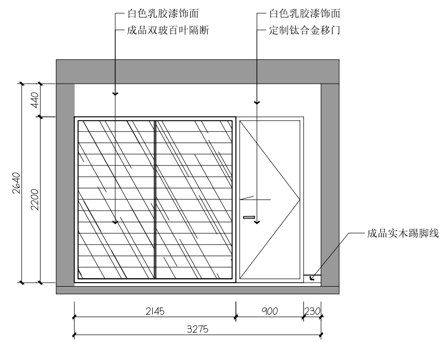
08 心理咨询室08立面图 Scale 1:50
