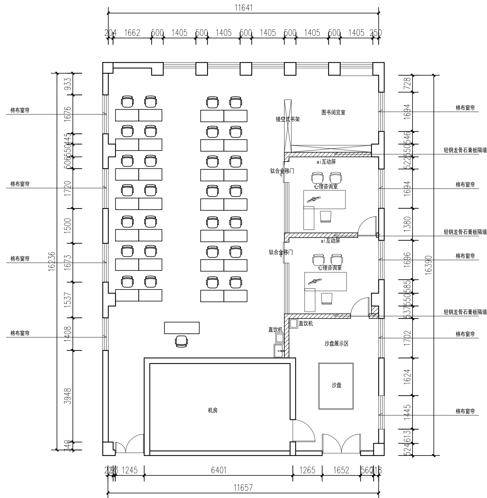
图书馆多媒体教室平面布置图
