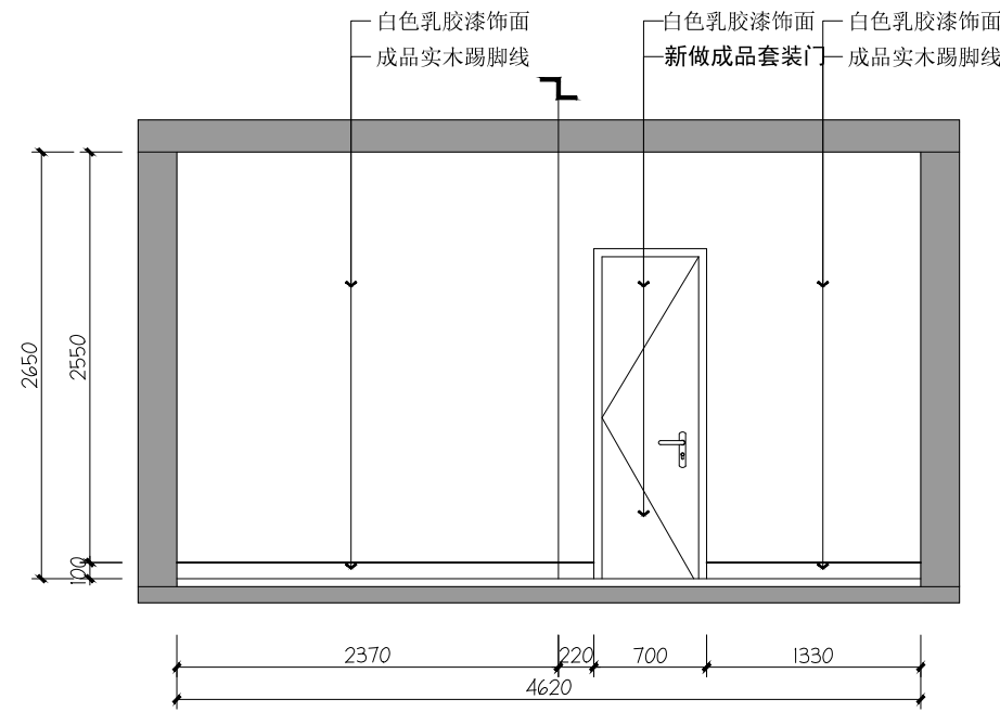
05 值班室05立面图 3F
