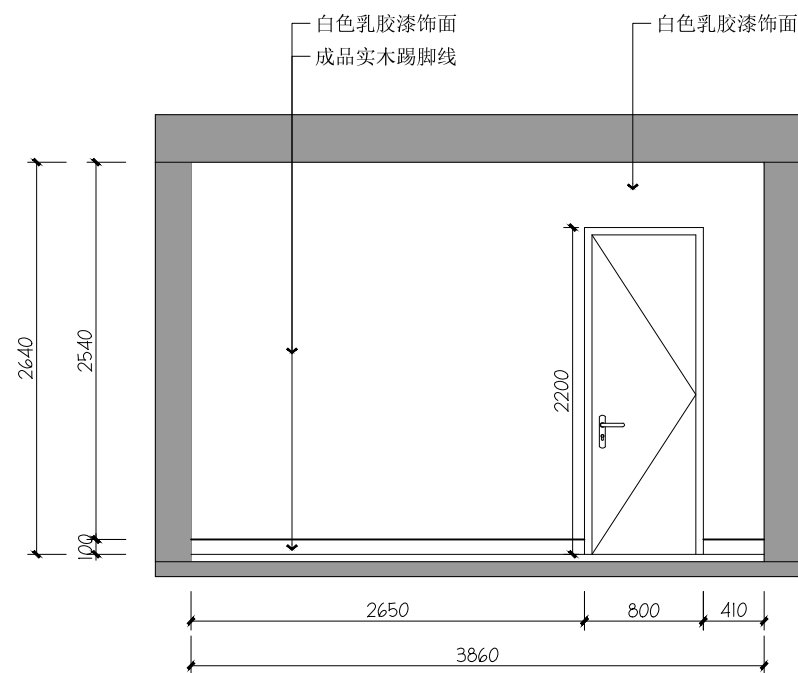
09 办公室09立面图 Scale 1:50
