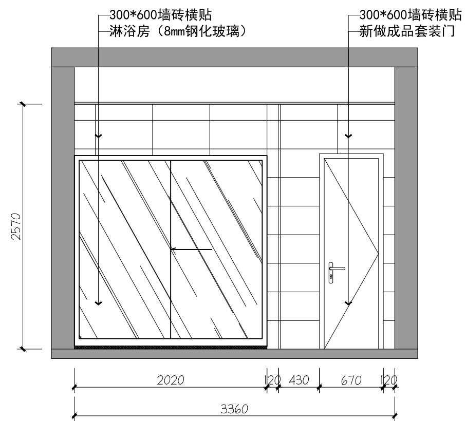
07 行政值班室07立面图 1F
