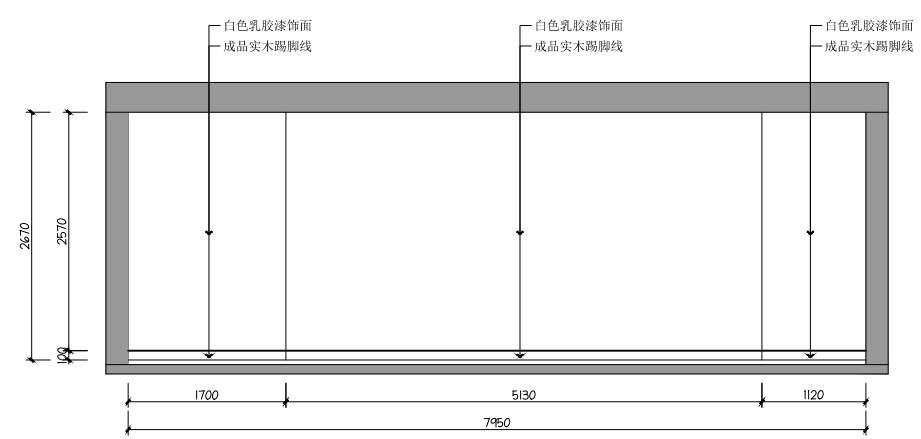
03 宣泄室03立面图 Scale 1:50
