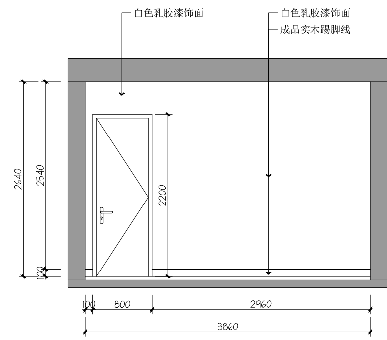
07 心理咨询室07立面图 Scale 1:50
