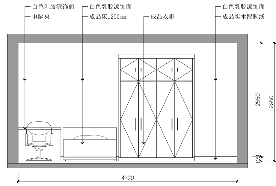
10 1F 值班室10立面图
