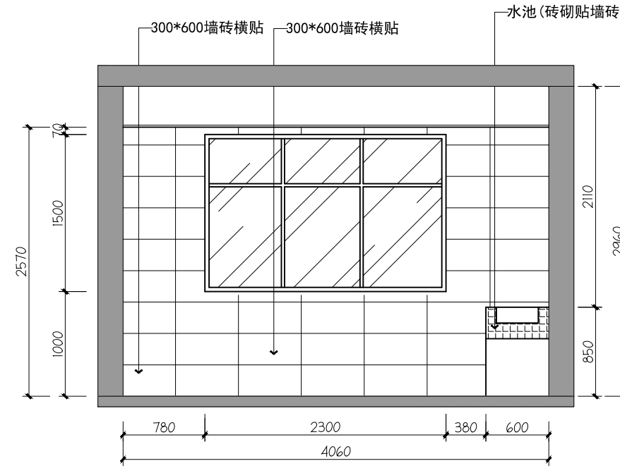
02 卫生间02立面图 1F
