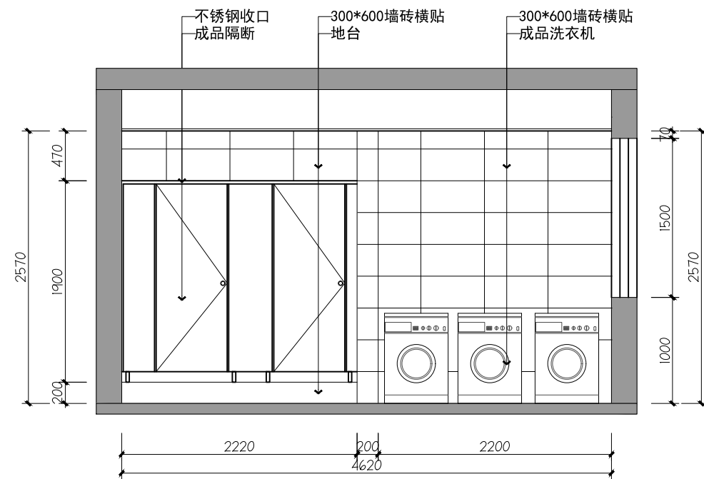
01 卫生间01立面图 3F
