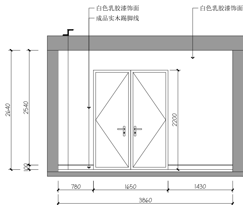
11 办公室11立面图 Scale 1:50
