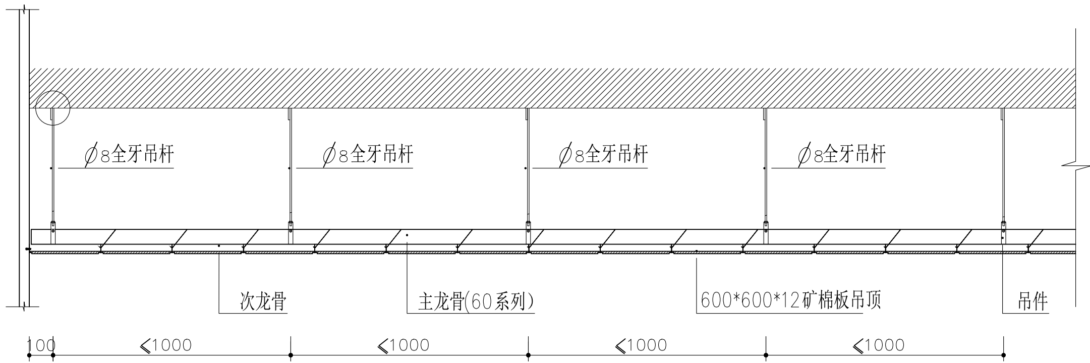
矿棉板吊顶节点图
