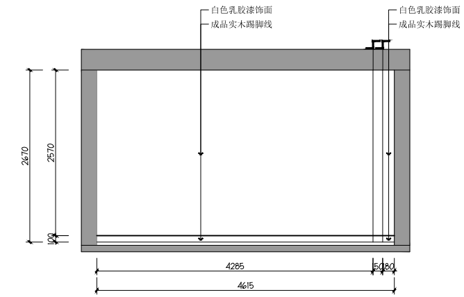
02 宣泄室02立面图 Scale 1:50
