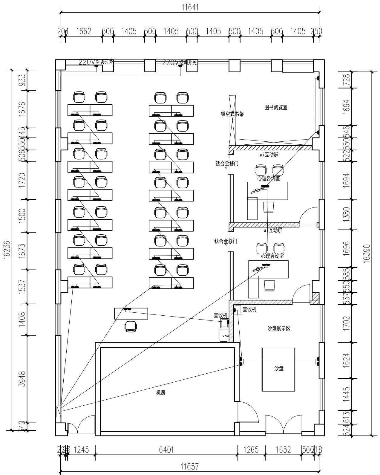
图书馆多媒体教室插座连线图
