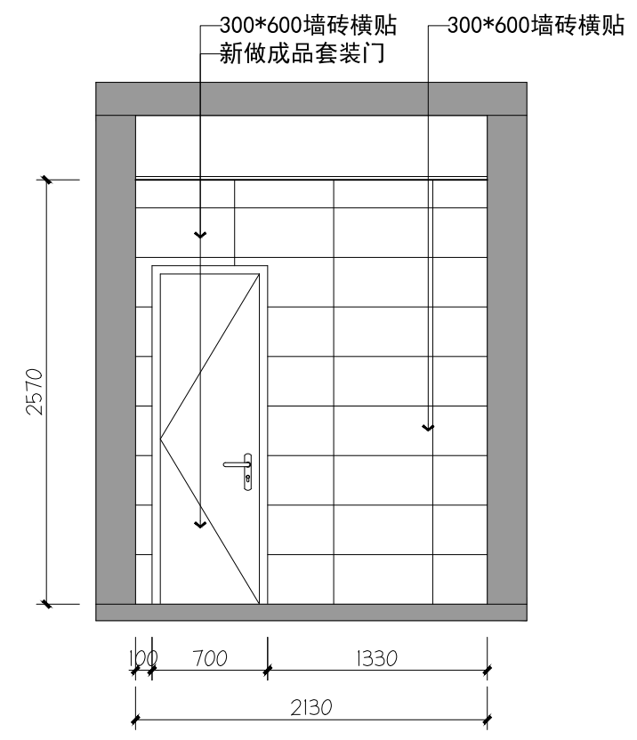
11 值班室卫生间11立面图 3F Scale 1:40
