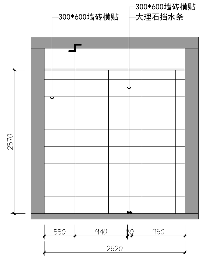
06 行政值班室06立面图 1F
