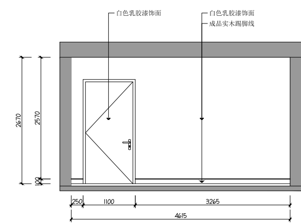
04 宣泄室04立面图 Scale 1:50
