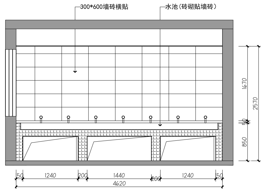
03 卫生间03立面图 3F
