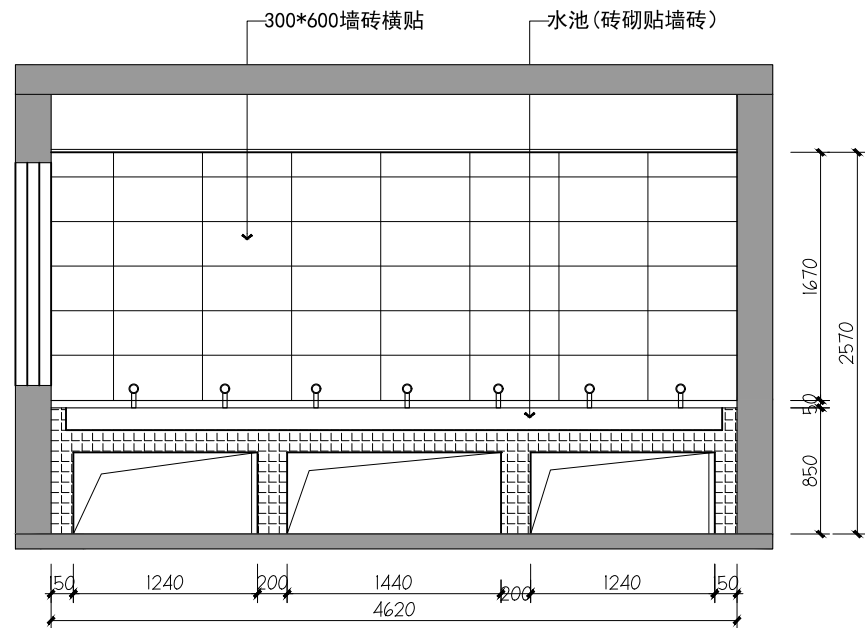
03 卫生间03立面图 1F
