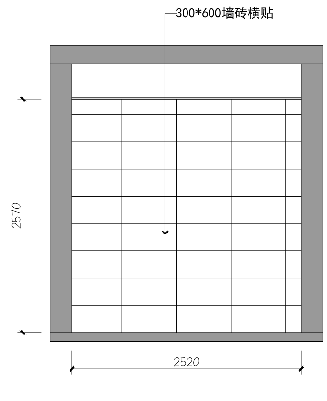
08 行政值班室08立面图 1F
