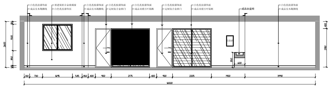
02 图书馆多媒体教室02立面图 Scale 1:100
