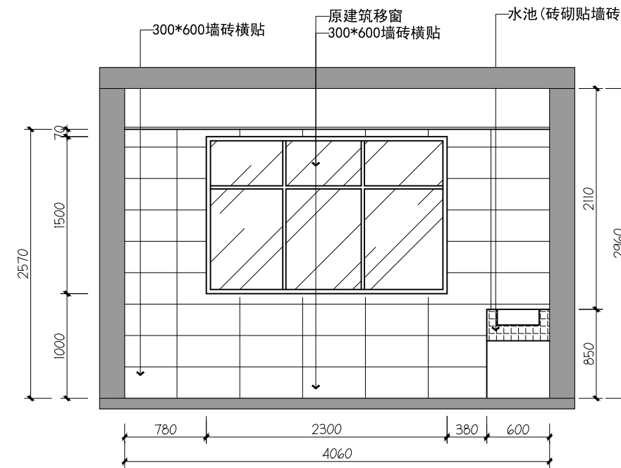
02 卫生间02立面图 3F
