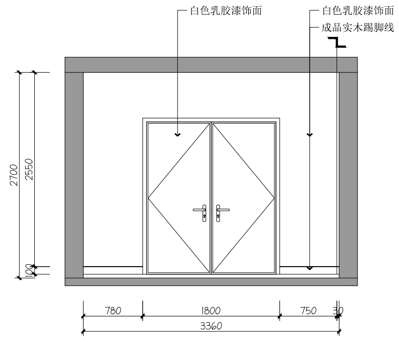
11 1F 值班室11立面图
