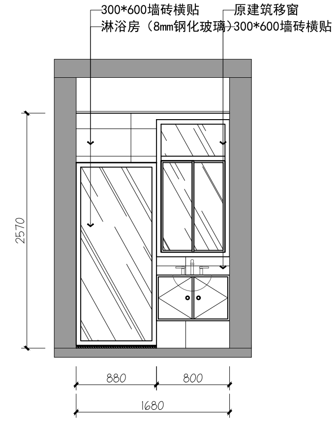
10 值班室卫生间10立面图 3F Scale 1:40
