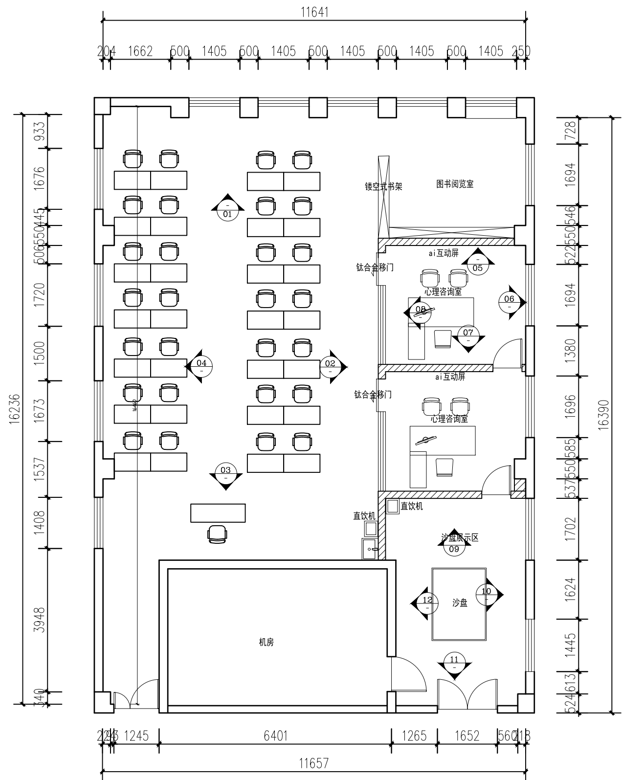
图书馆多媒体教室立面索引图
