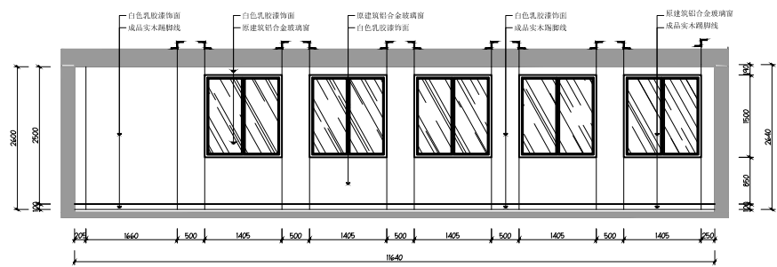
01 图书馆多媒体教室01立面图 Scale 1:100
