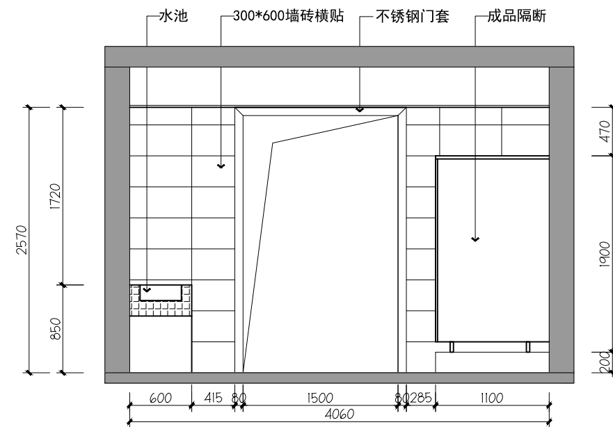
04 卫生间04立面图 3F
