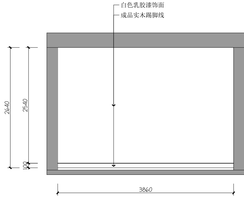
05 心理咨询室05立面图 Scale 1:50
