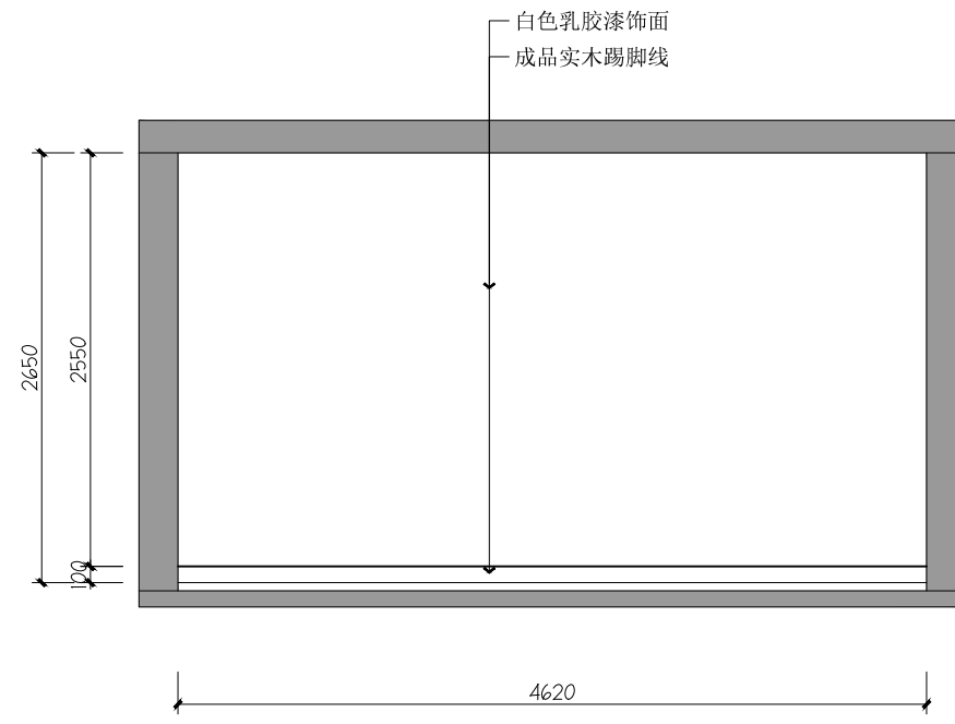
07 值班室07立面图 3F
