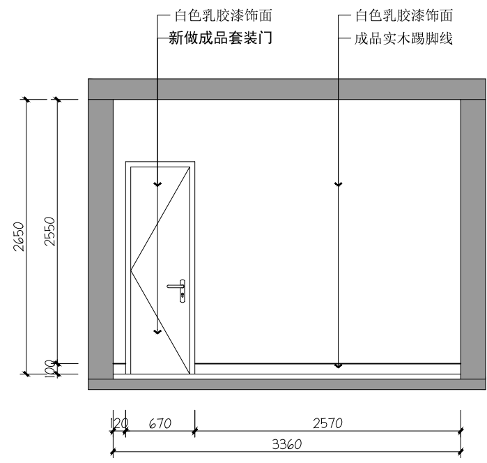
09 1F 值班室09立面图
