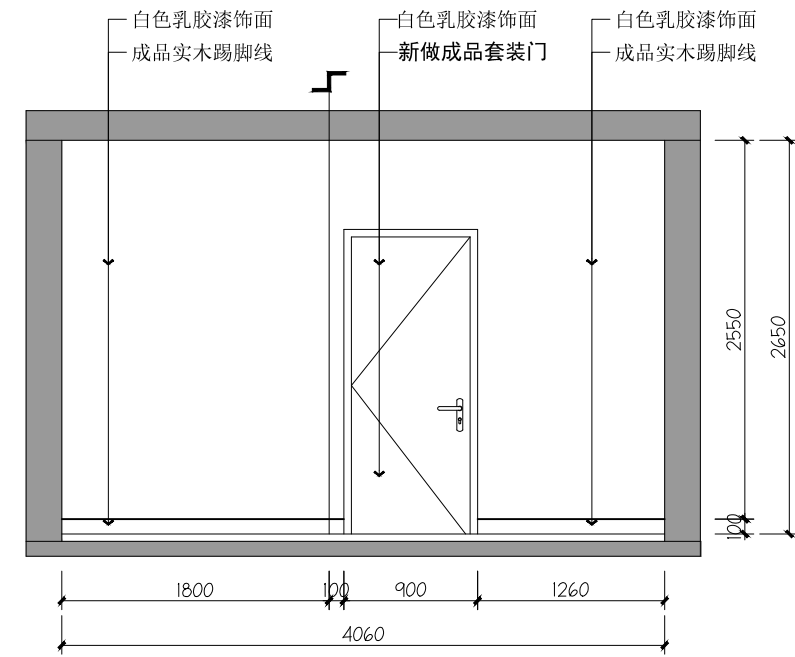
06 值班室06立面图 3F
