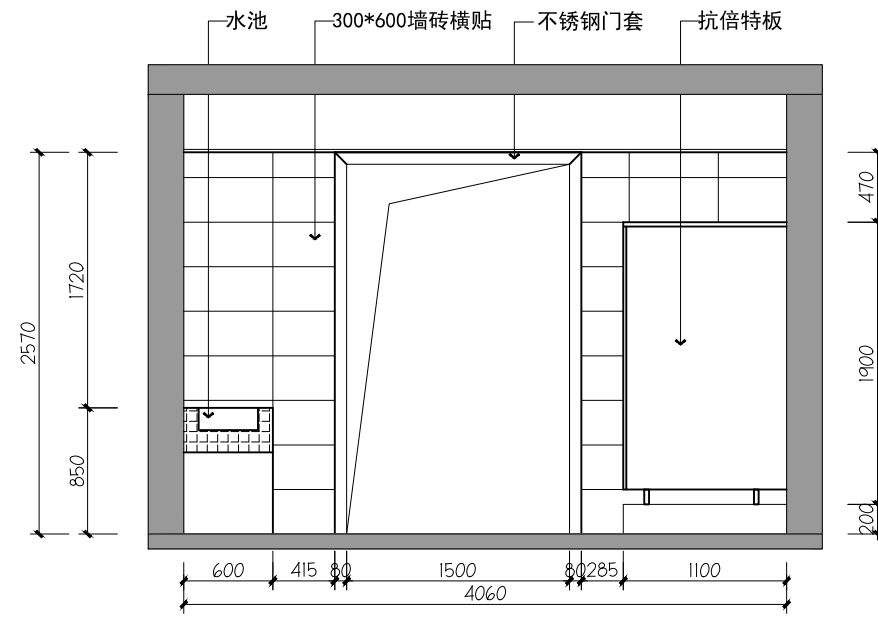
04 卫生间04立面图 1F
