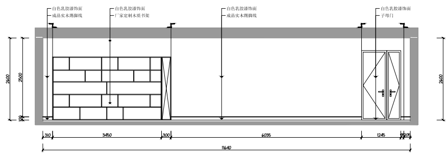
03 图书馆多媒体教室03立面图 Scale 1:100
