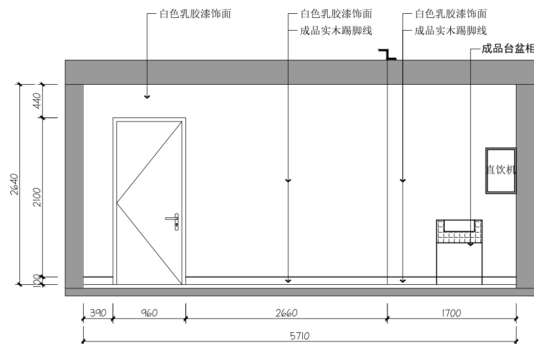
12 办公室12立面图 Scale 1:50
