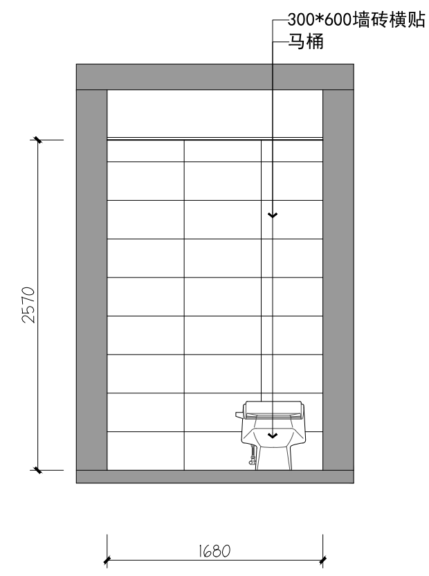
12 值班室卫生间12立面图 3F Scale 1:40
