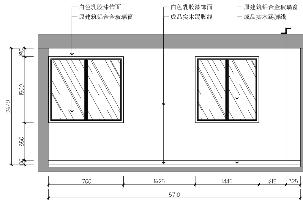
10 办公室10立面图 Scale 1:50
