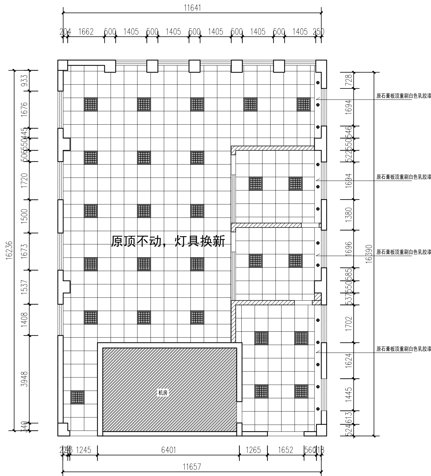
图书馆多媒体教室顶面布置图
