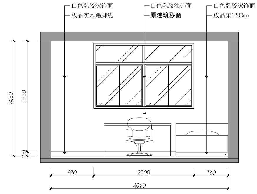
08 值班室08立面图 3F
