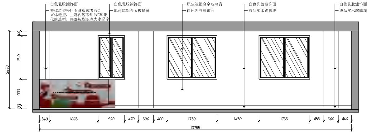
01 党建室01立面图 Scale 1:50
