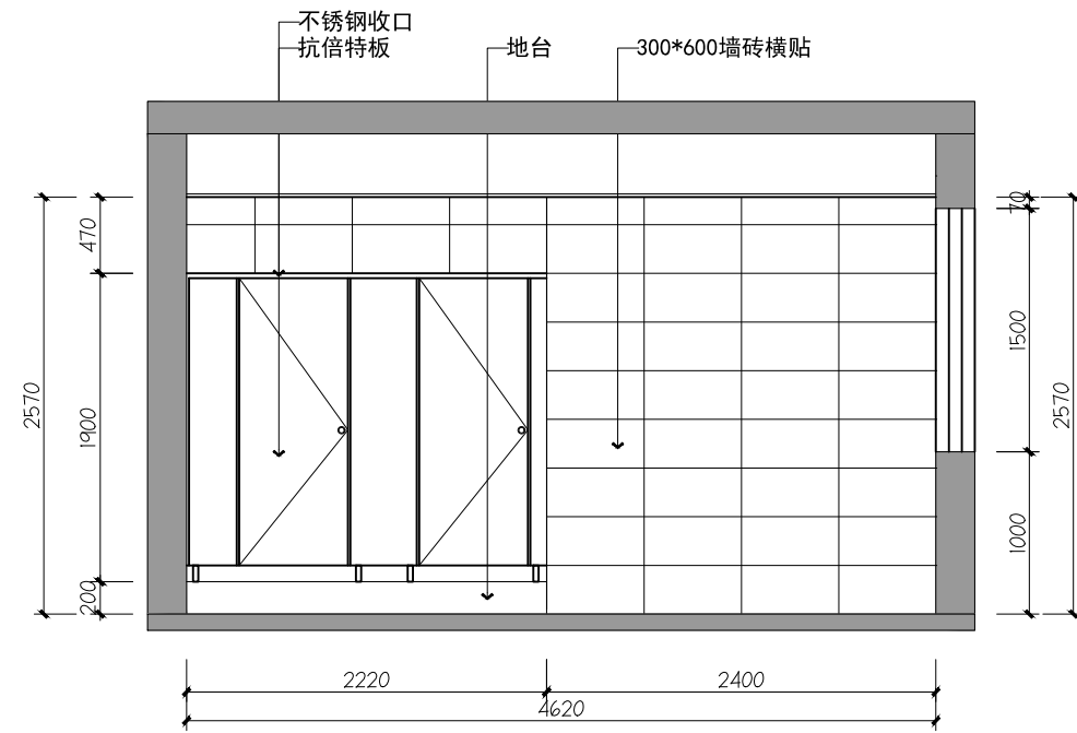
01 卫生间01立面图 1F
