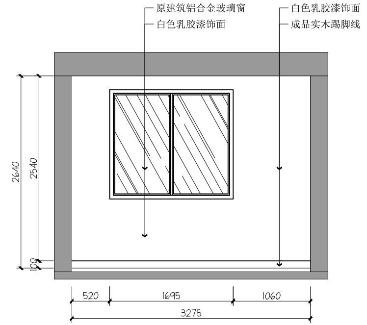
06 心理咨询室06立面图 Scale 1:50
