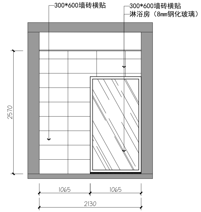
09 值班室卫生间09立面图 3F Scale 1:40
