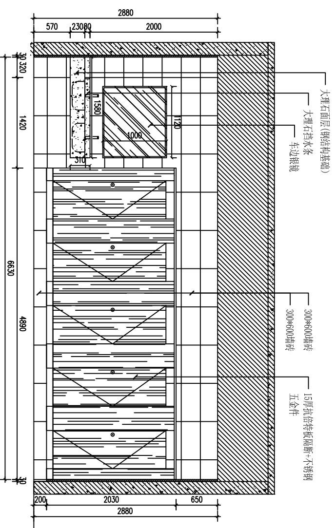
C SCALE 女卫 C立面图 1:40
