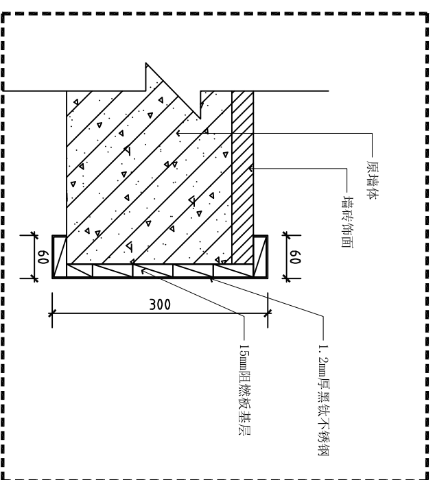
不锈钢门套节点图 JD SCALE 1:5
