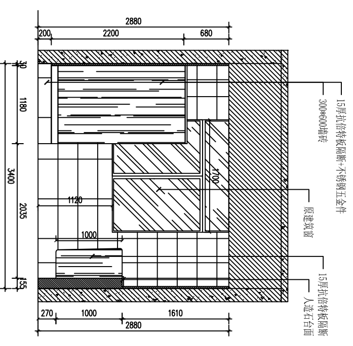
男卫 D立面图 SCALE 1:40
