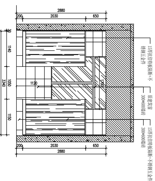
D SCALE 女卫 D立面图 1:40
