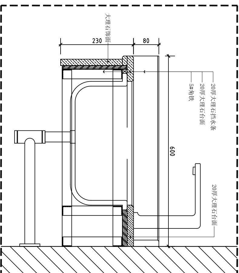
台盆柜剖面图 JD SCALE 1:5
