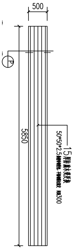
F1 SCALE 防腐木凳更换平面图 1:30
