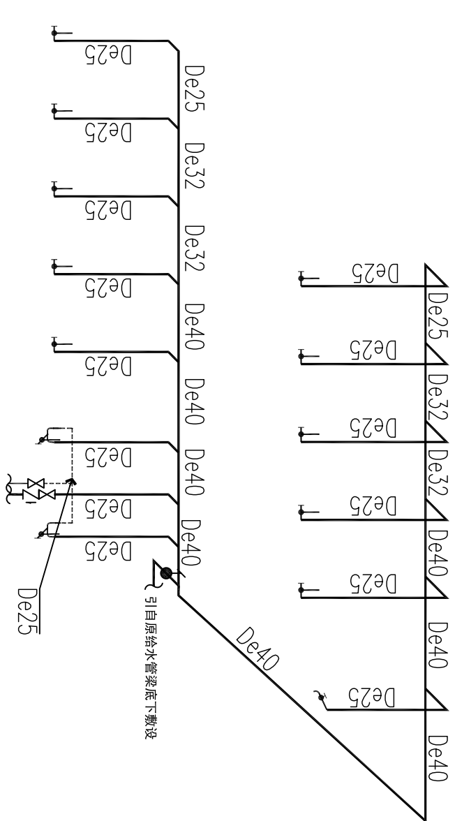
PLAN 女卫给水系统图 SCALE 1:100
