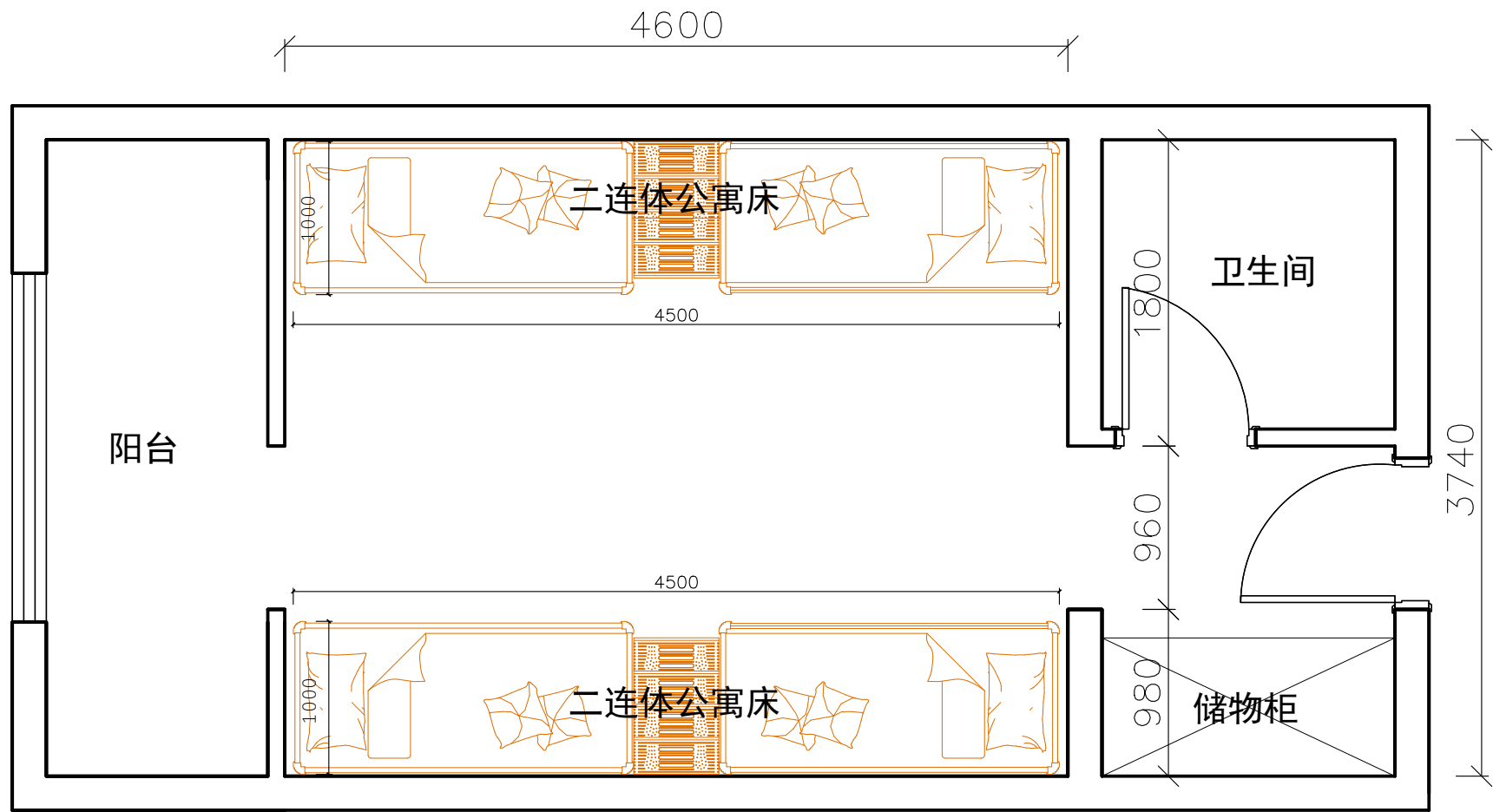
学生公寓家具平面布置图
