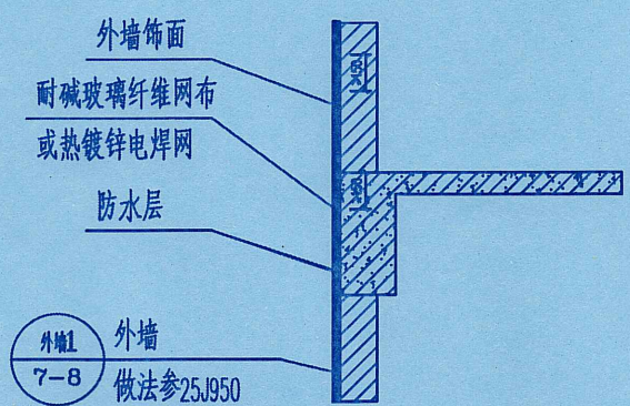
②外墙墙身防水构造做法 1:25
