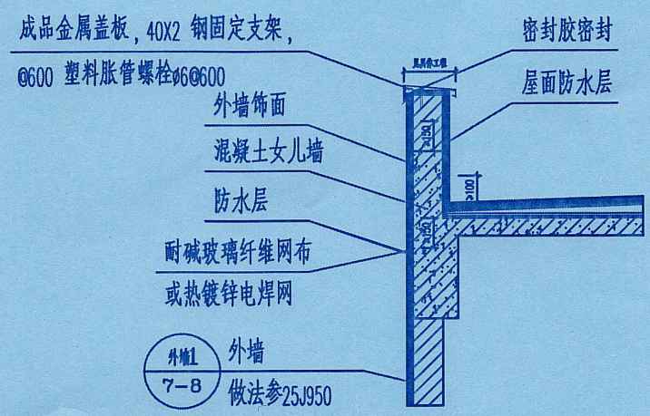
①女儿墙防水构造做法 1:25
