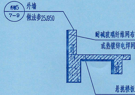
③悬挑外墙构造做法 1:25
