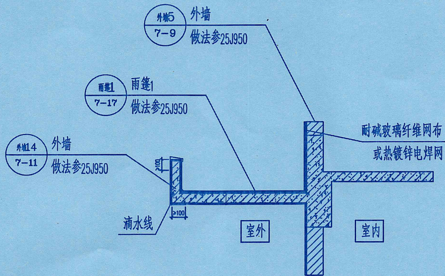
①开敞式外廊顶棚构造做法 1:25
