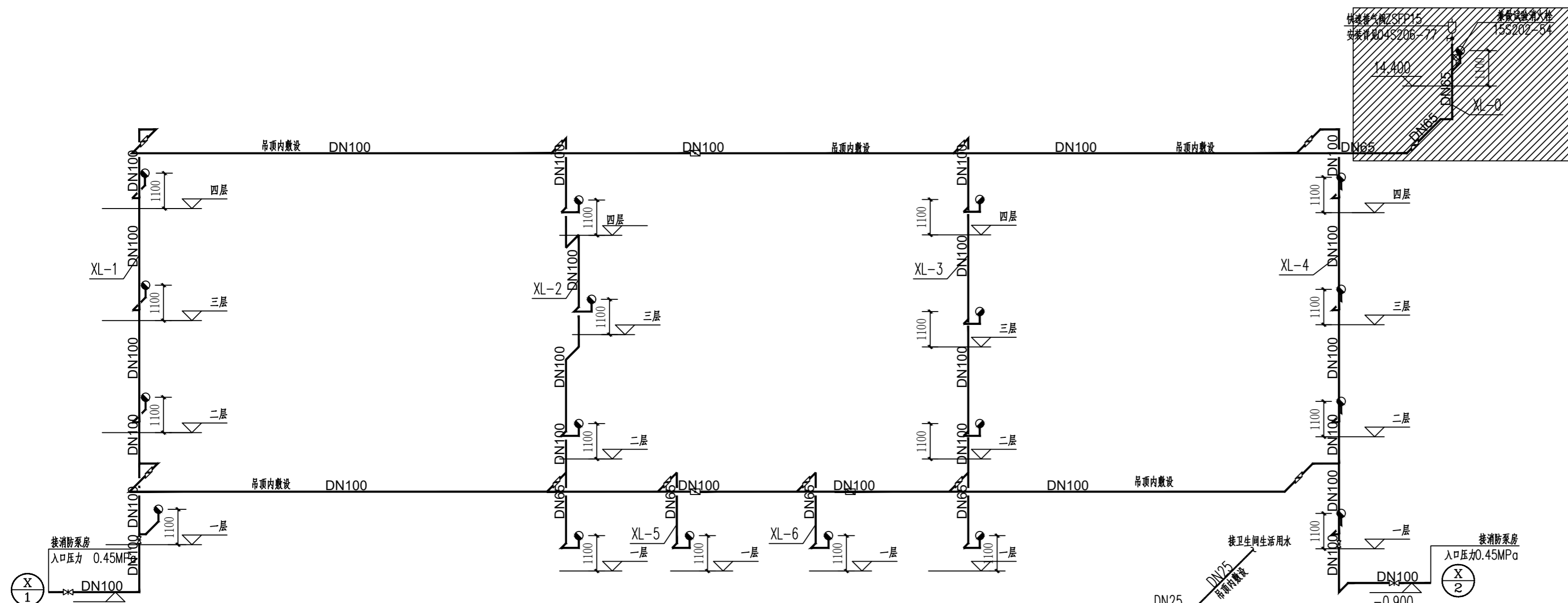
消火栓系统原理图
