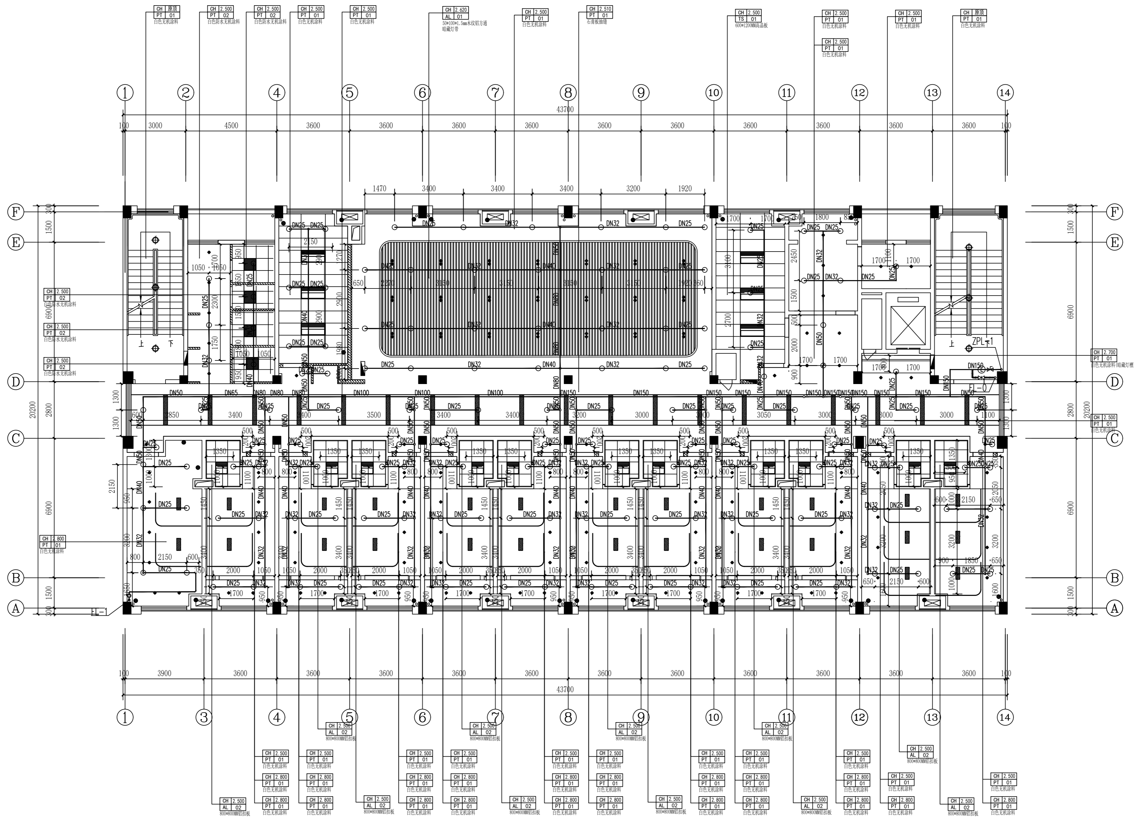
四层自动喷淋平面图 1:100
