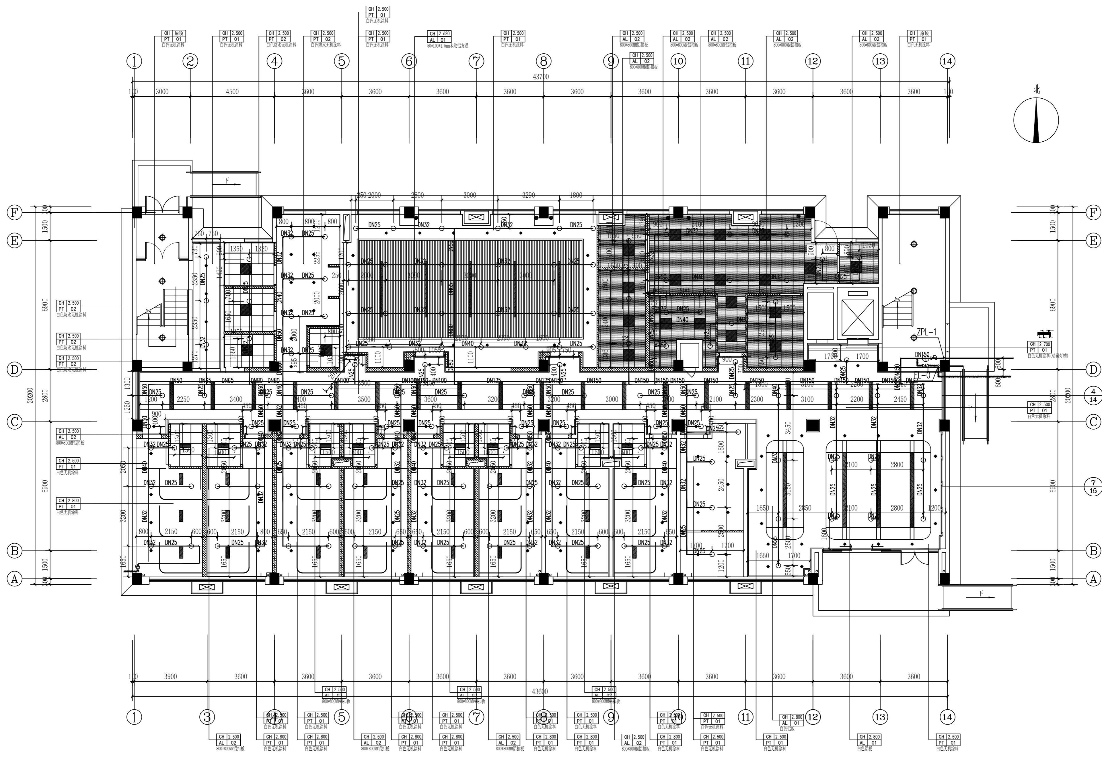
一层自动喷淋平面图 1:100
