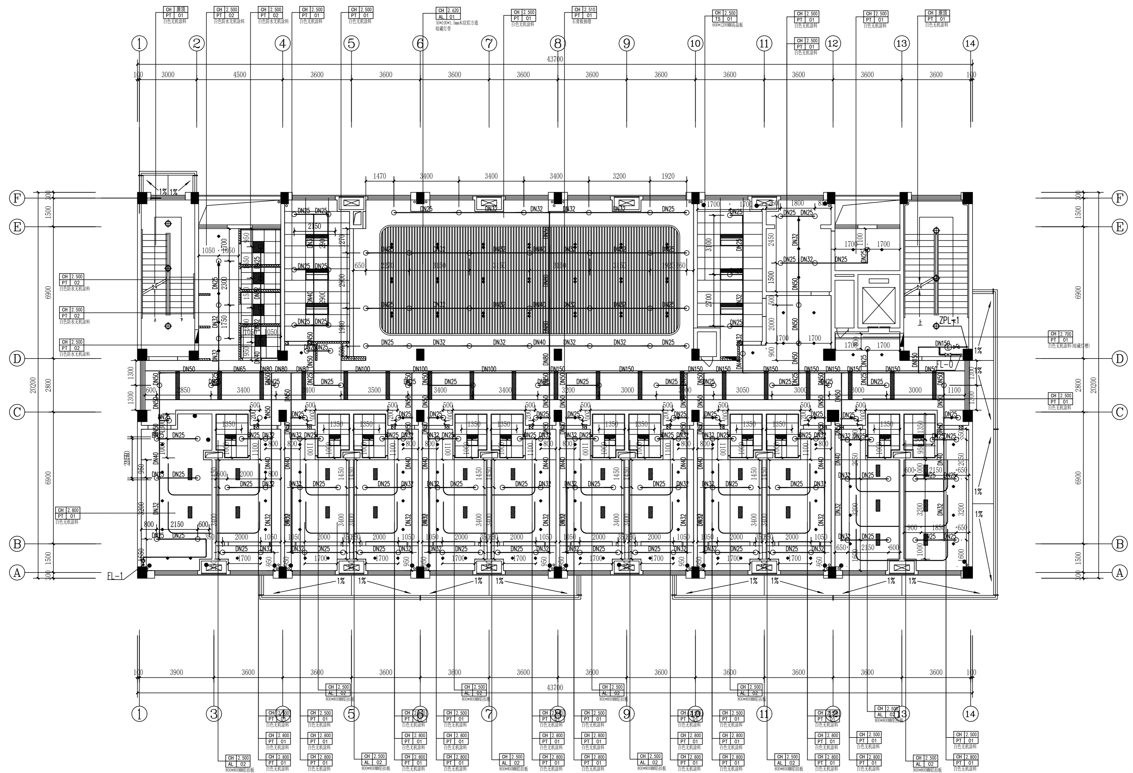
二层自动喷淋平面图 1:100
