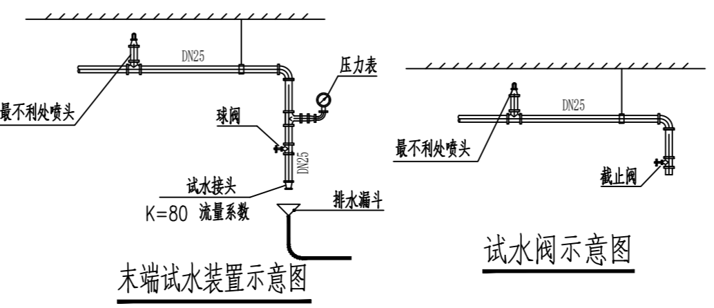
喷淋管路安装示意图
