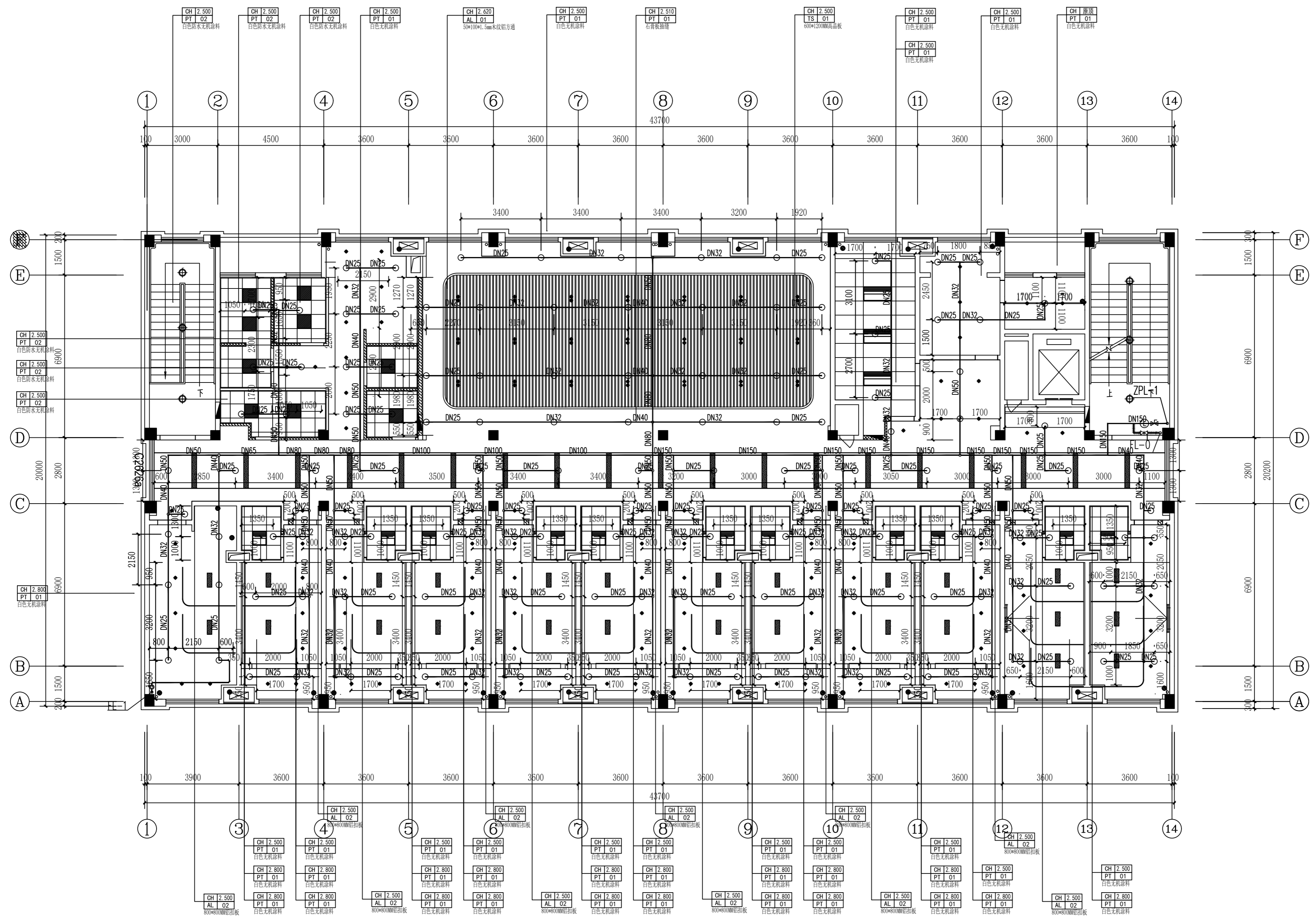
三层自动喷淋平面图 1:100
