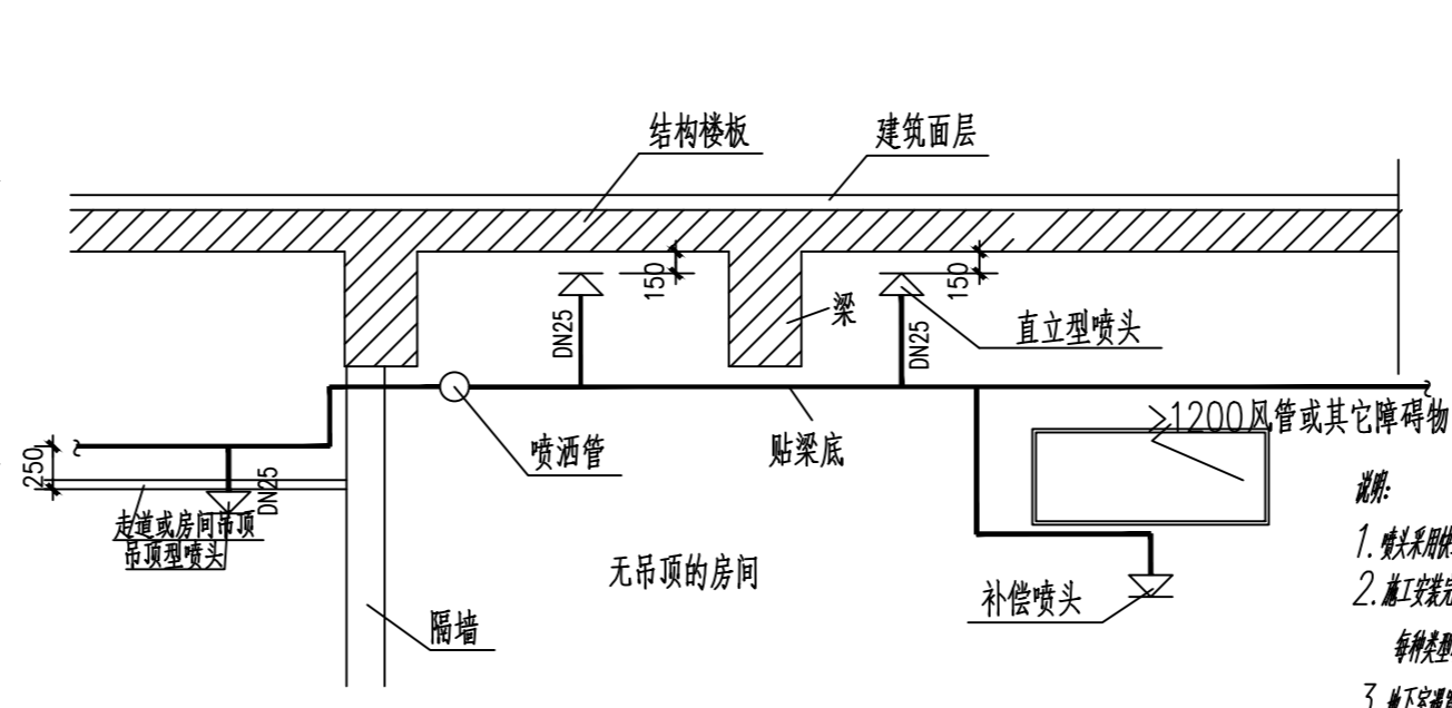
喷淋管路安装示意图
