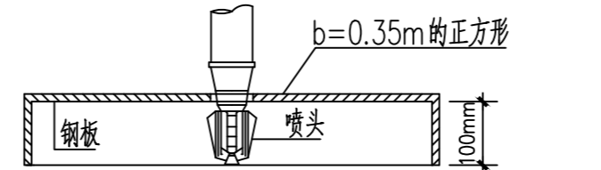
集热板安装示意图
